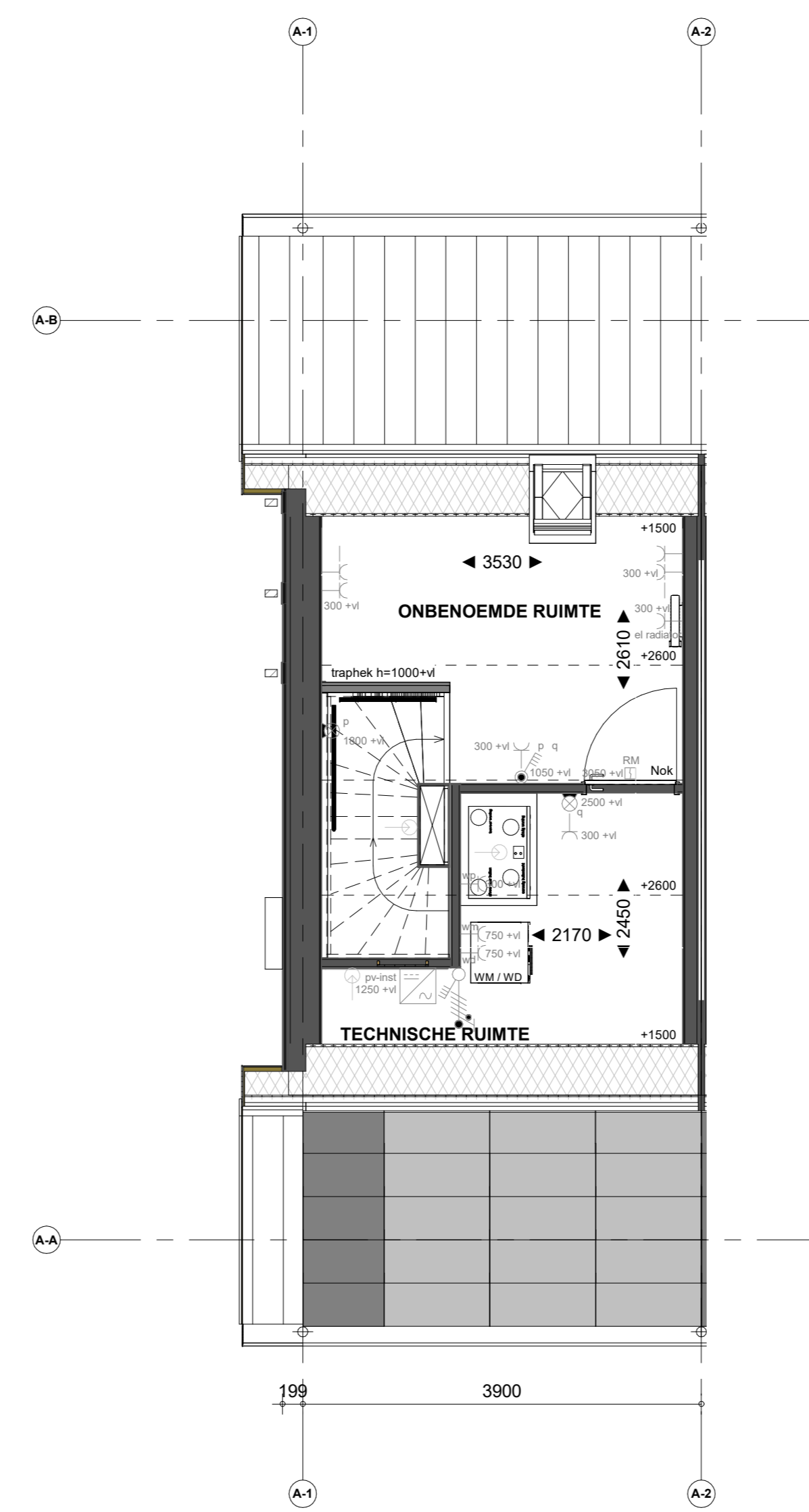
2e verdieping
