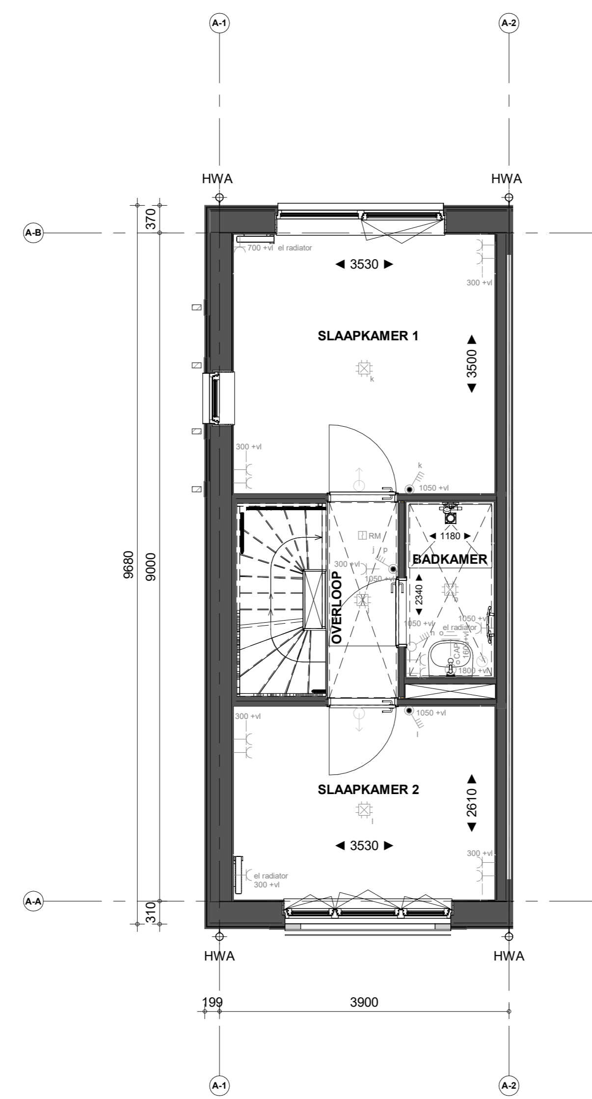
1e verdieping
