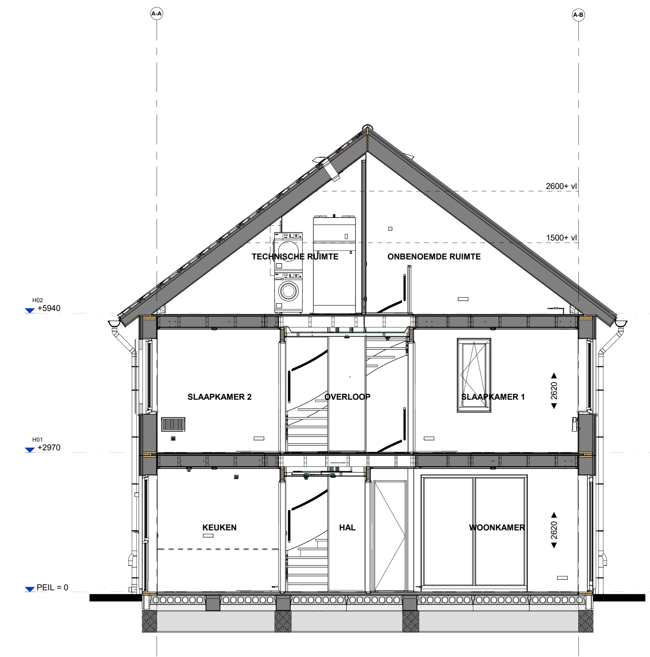
Doorsnede B501
