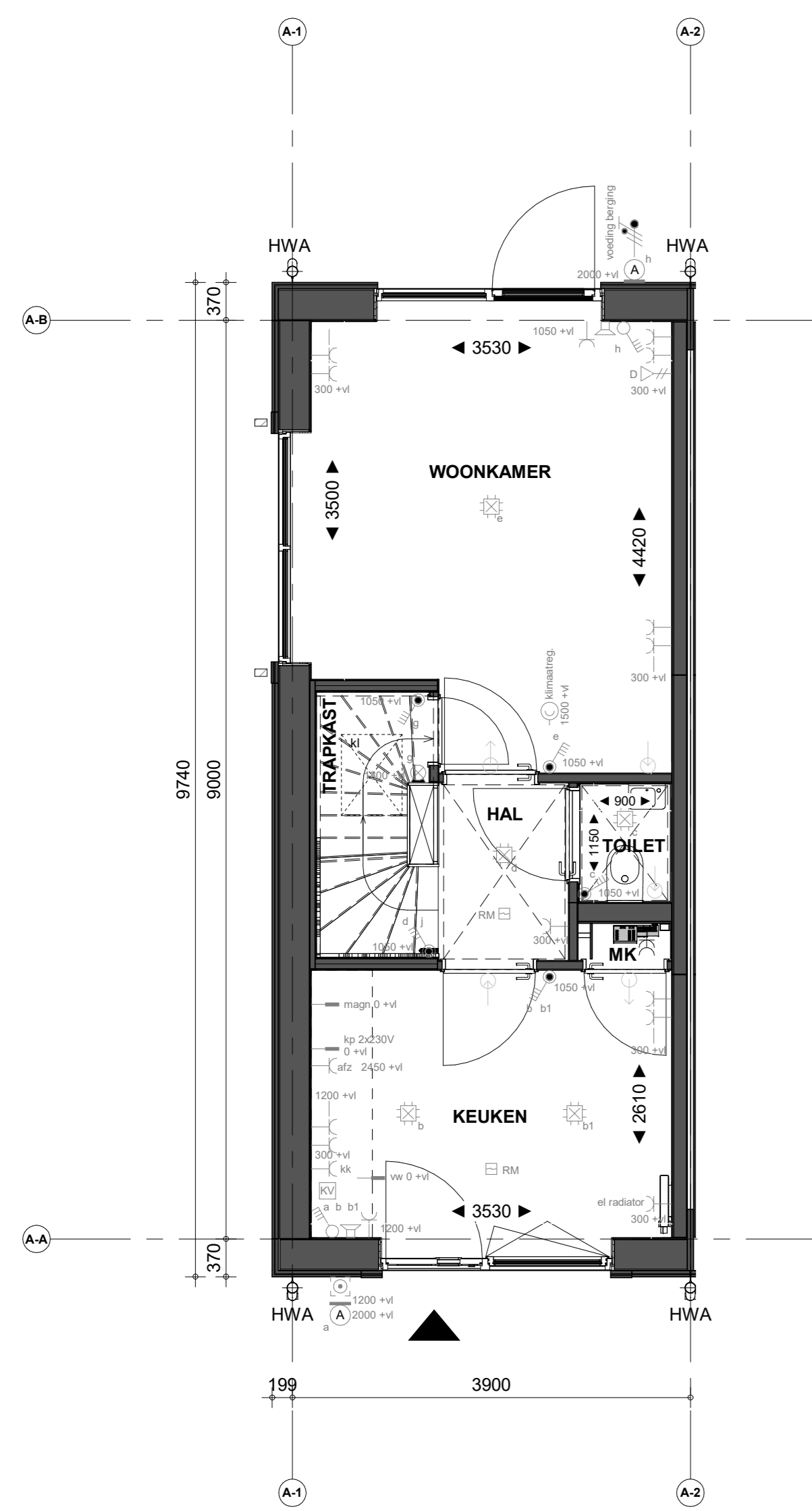
Begane grond
