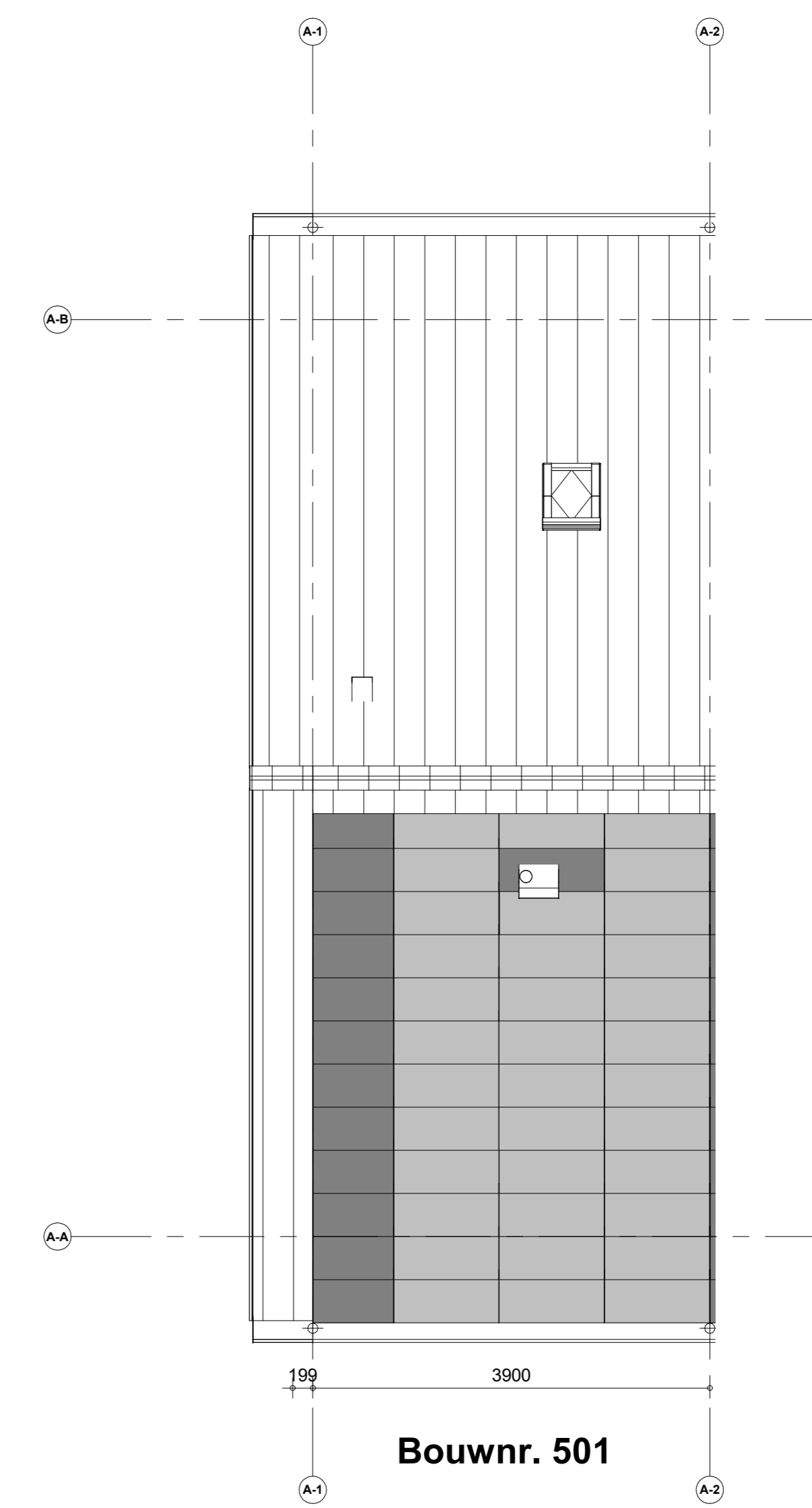
Dakaanzicht
