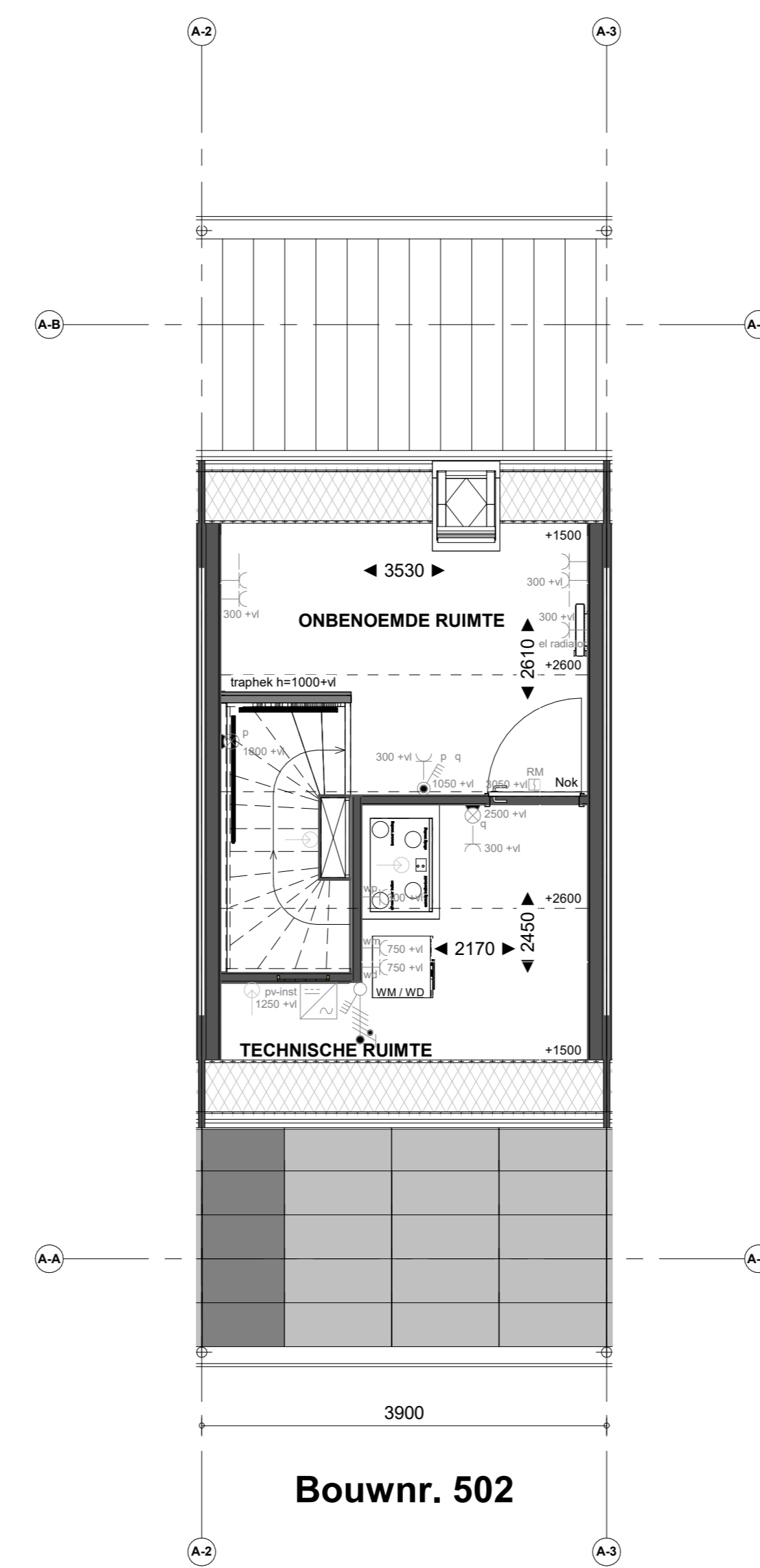
2e verdieping
