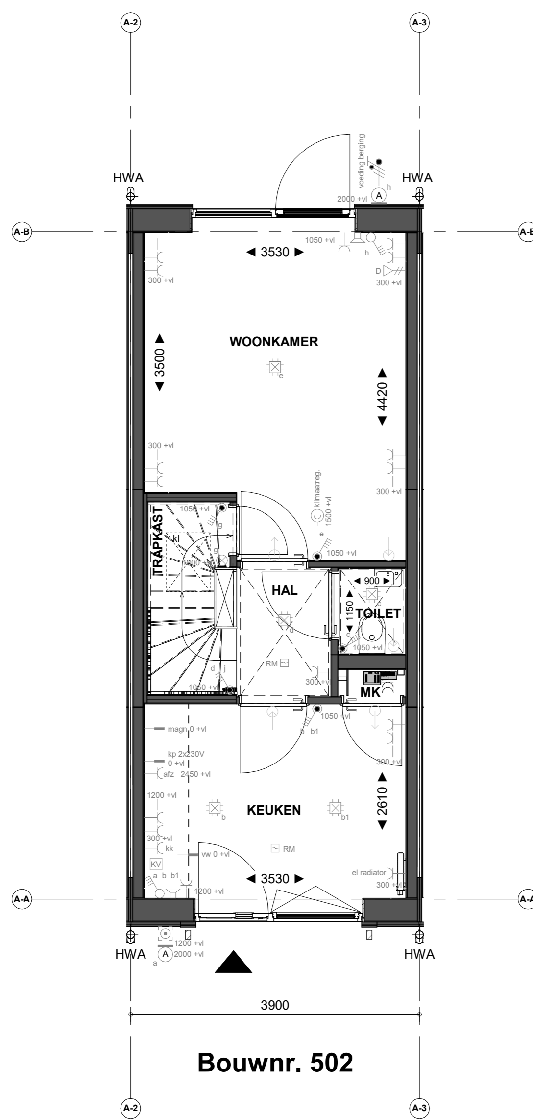
Begane grond
