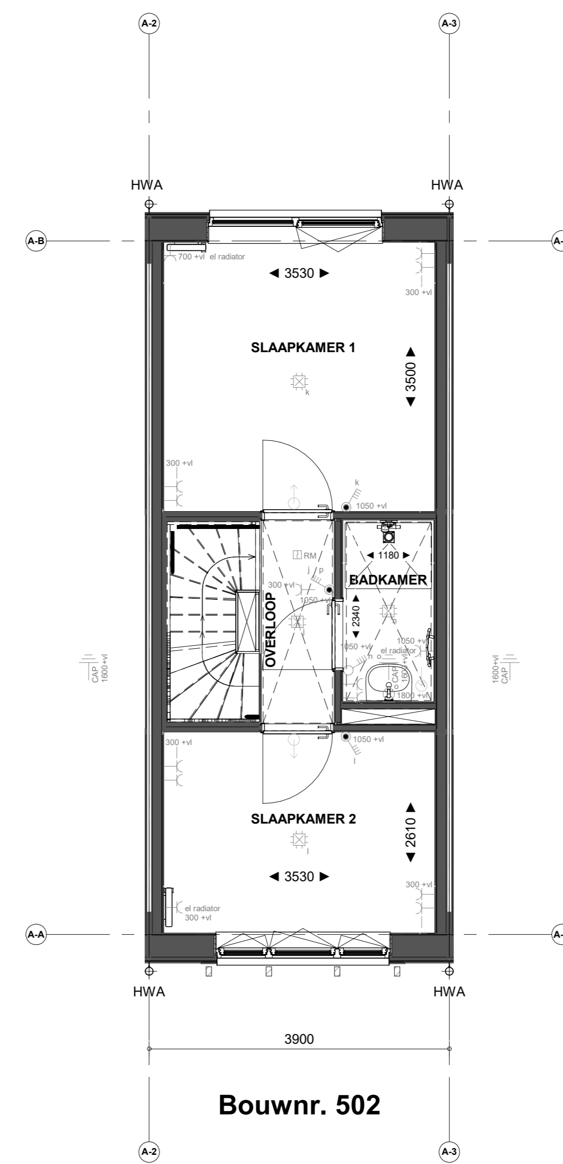
1e verdieping
