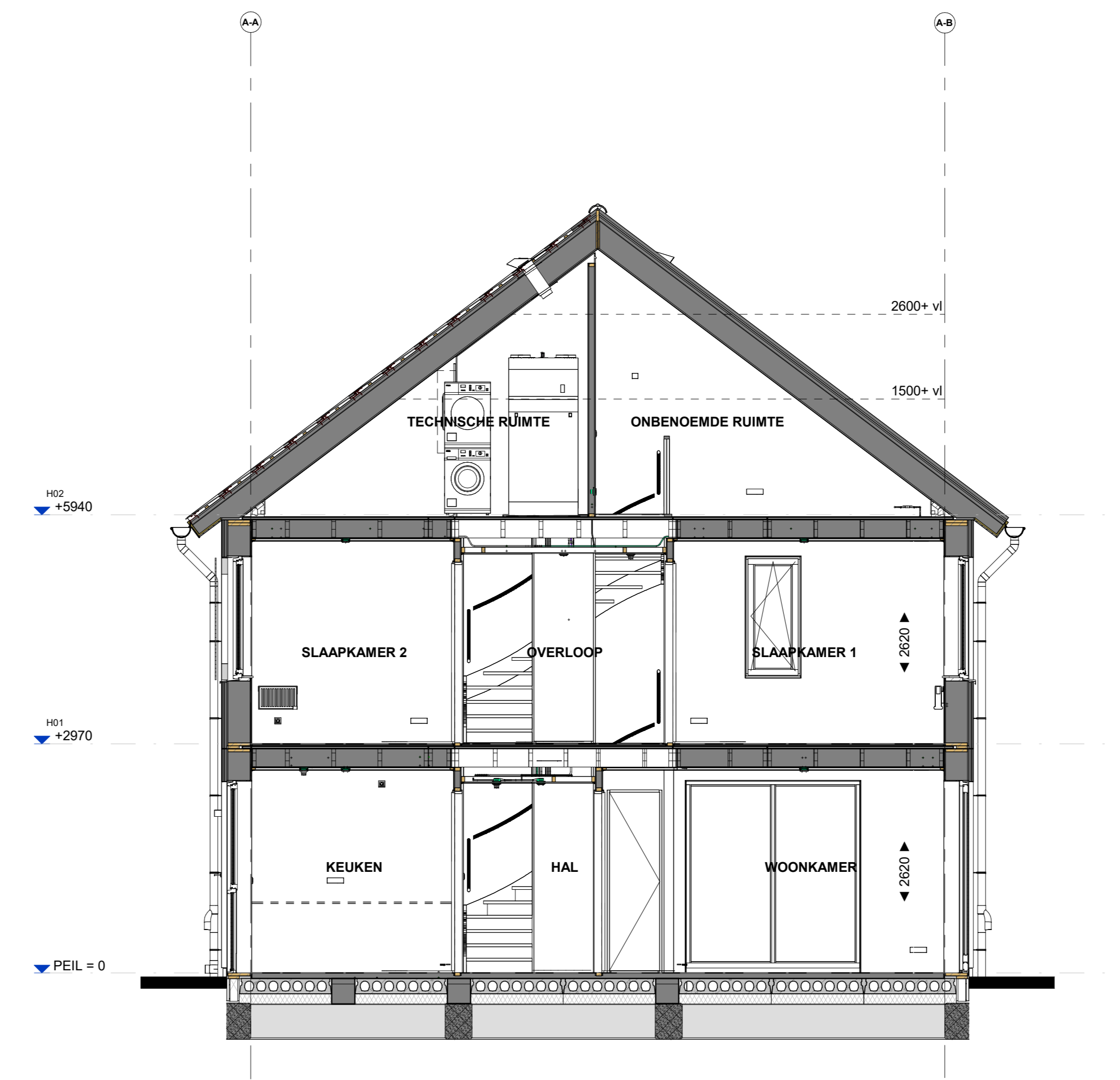
Doorsnede B502
