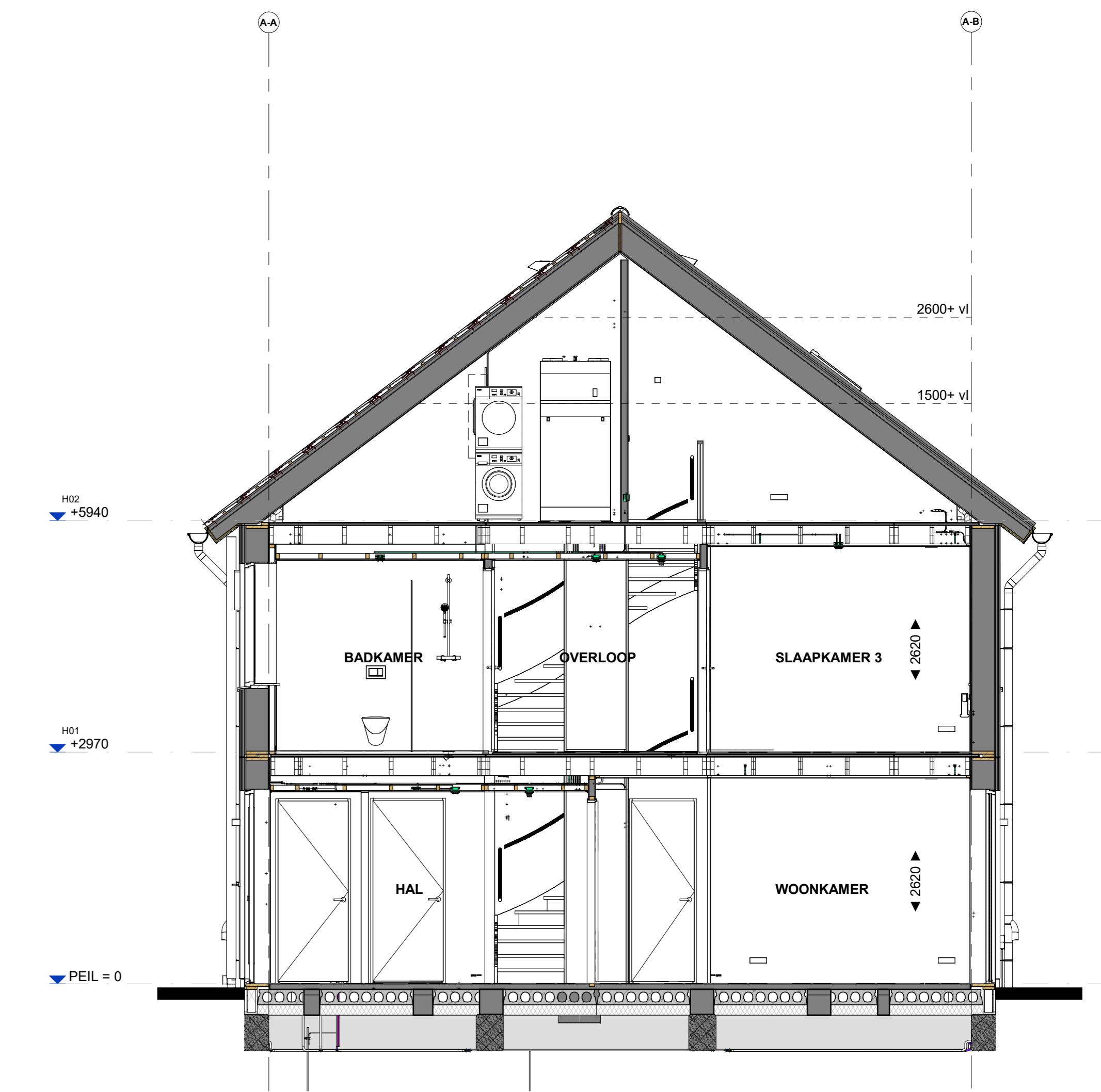
Doorsnede B504
