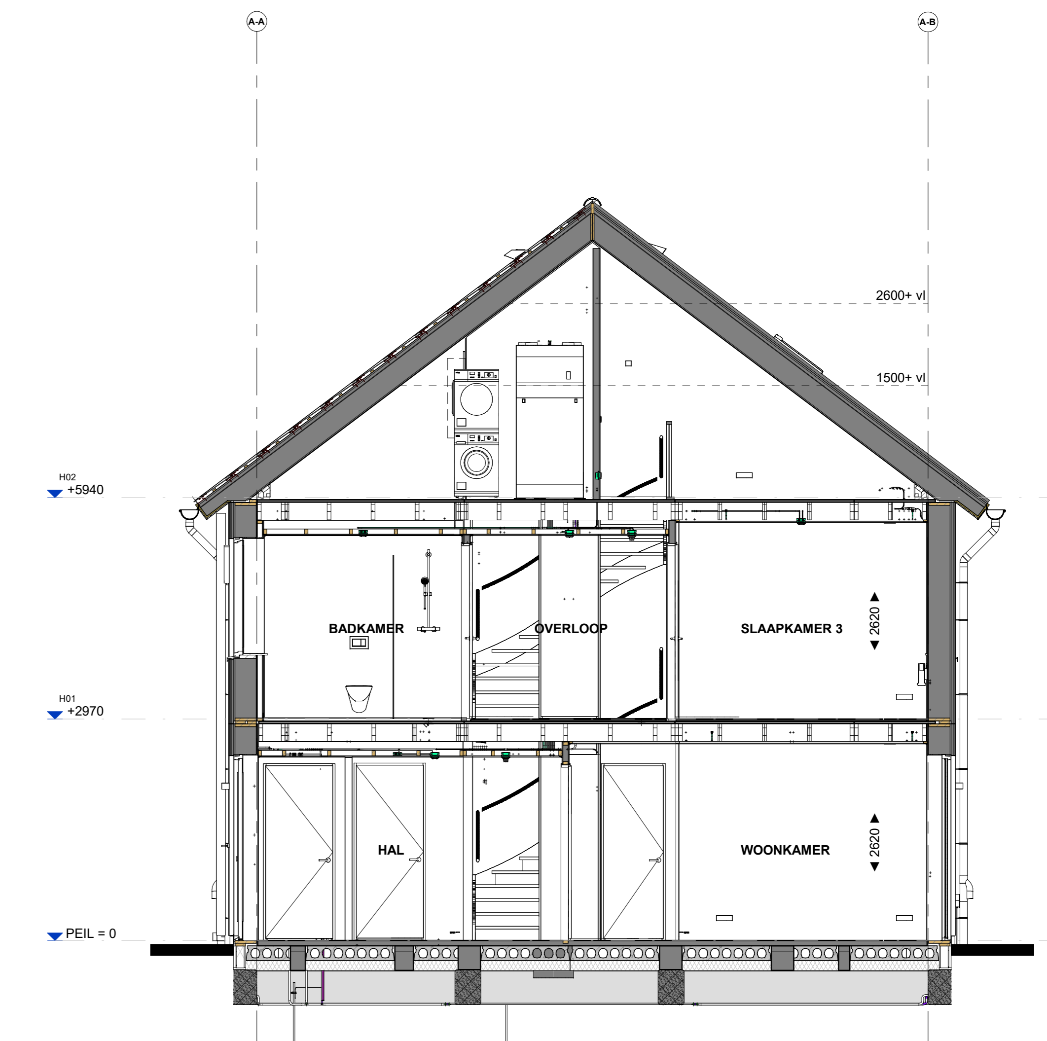
Doorsnede B505
