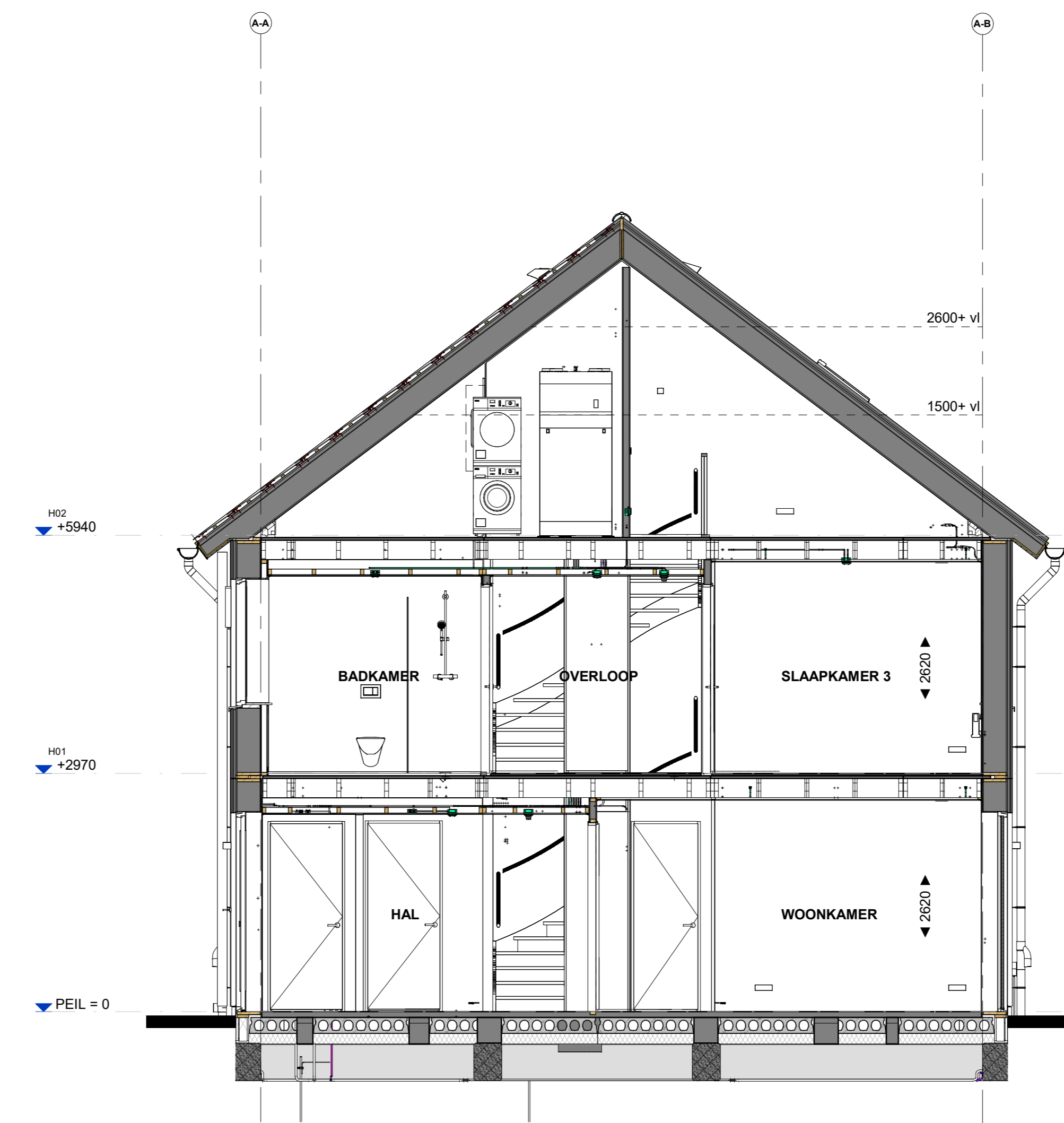
Doorsnede B507
