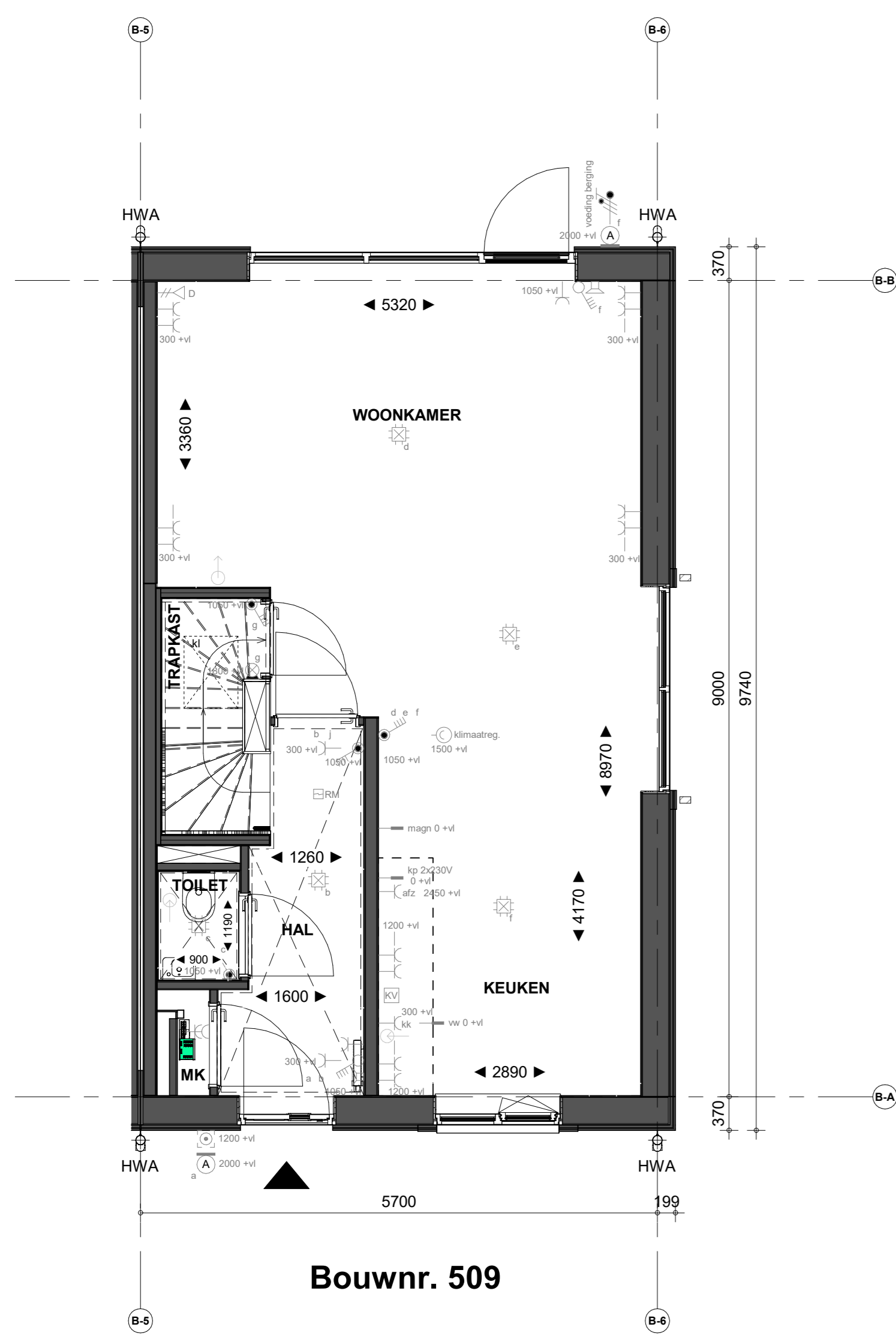
Begane grond
