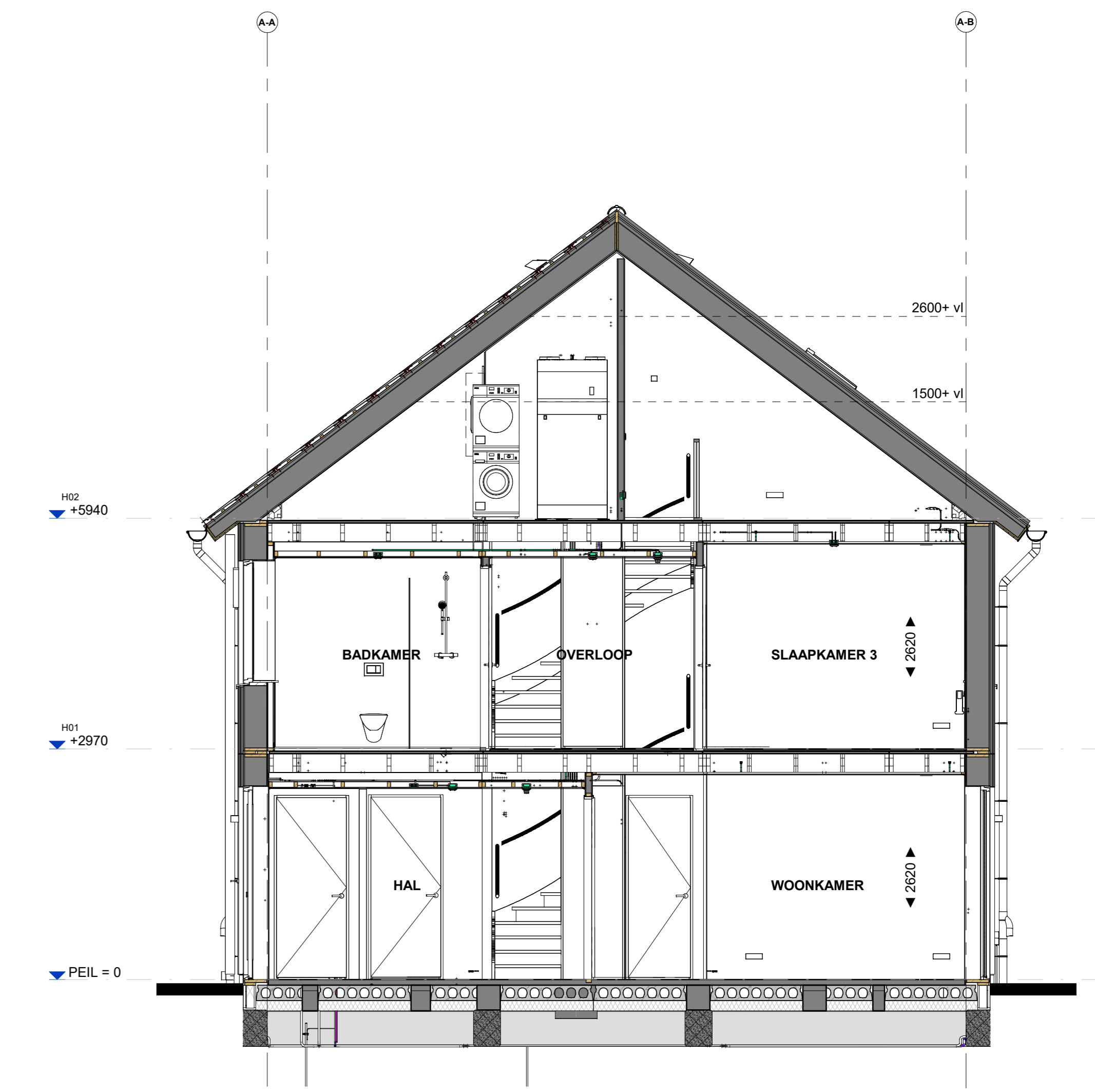
Doorsnede B509
