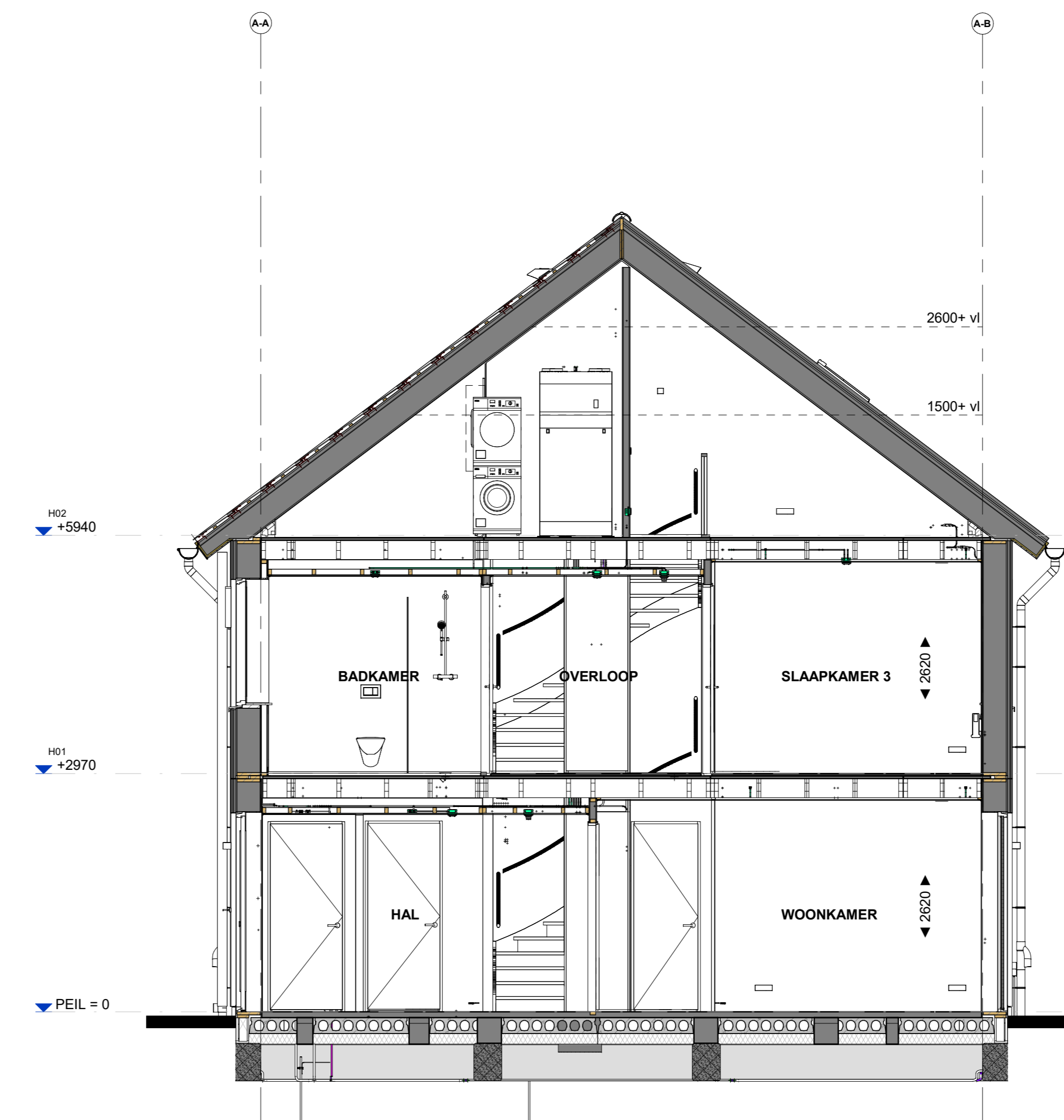
Doorsnede B511
