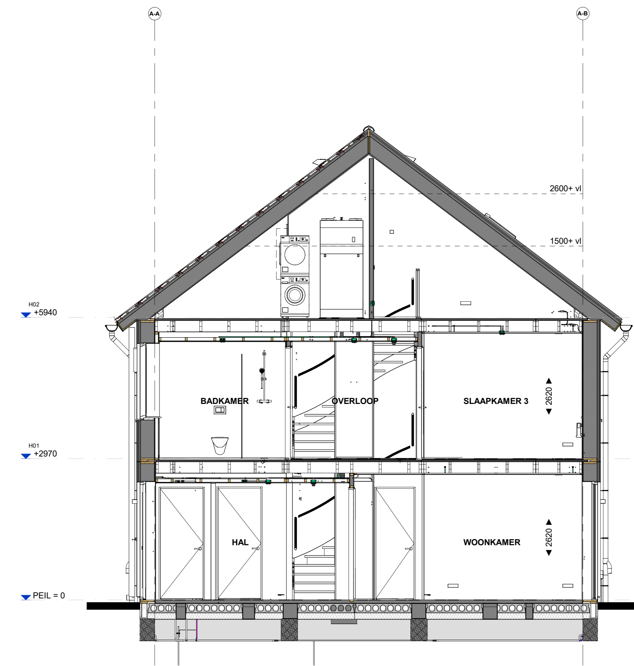
Doorsnede B512
