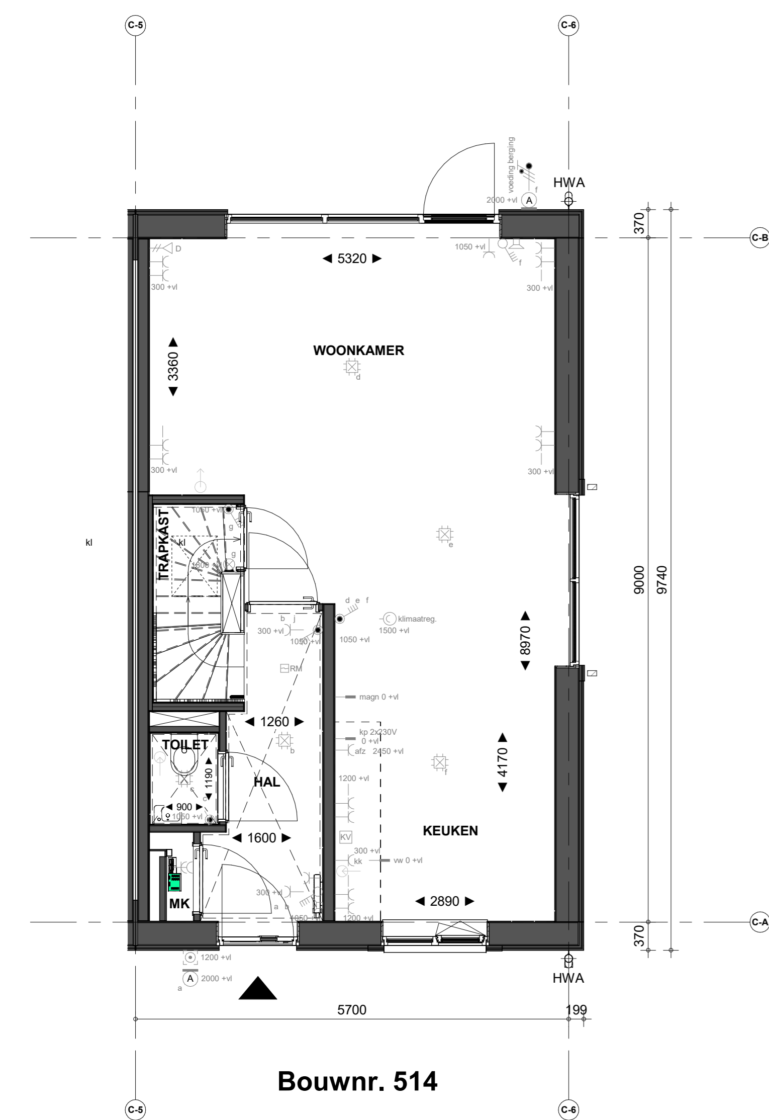
Begane grond
