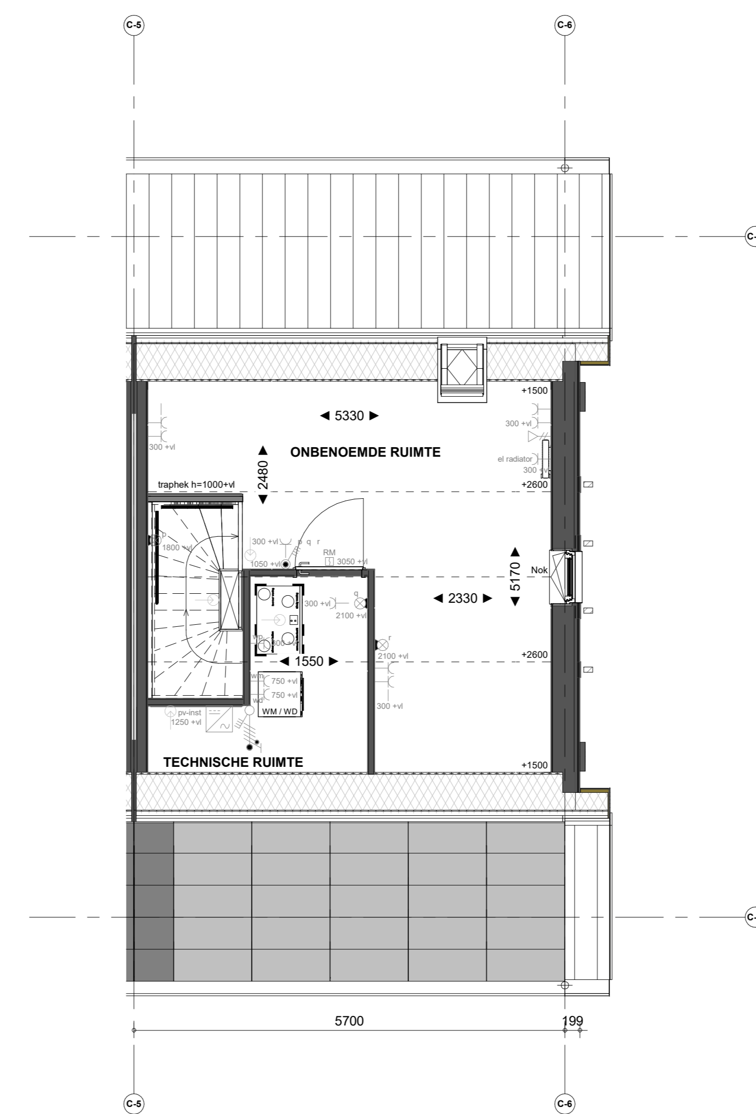
2e verdieping
