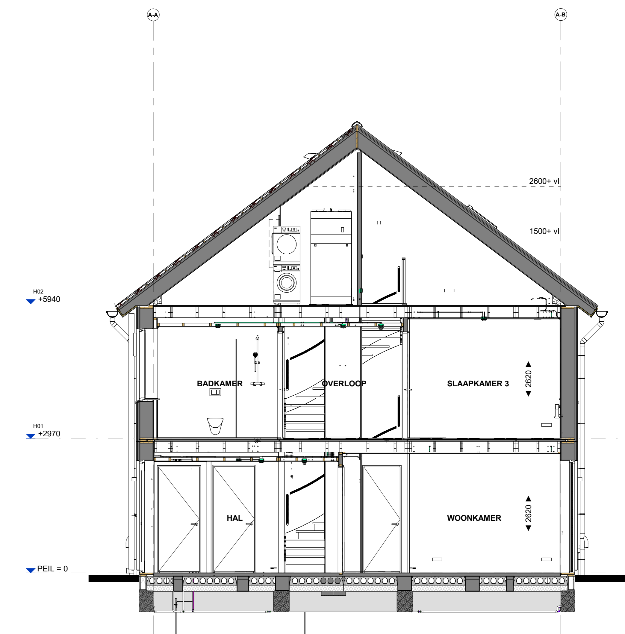
Doorsnede B514
