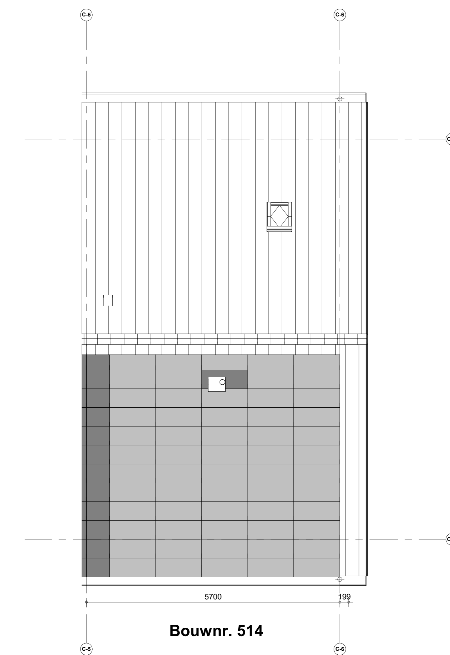
Dakaanzicht
