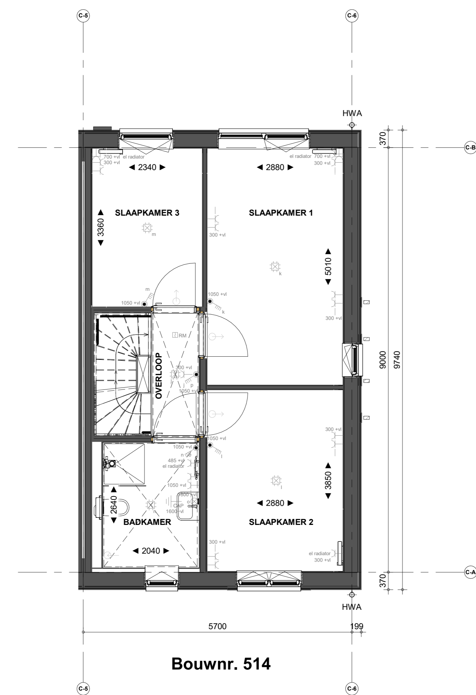
1e verdieping
