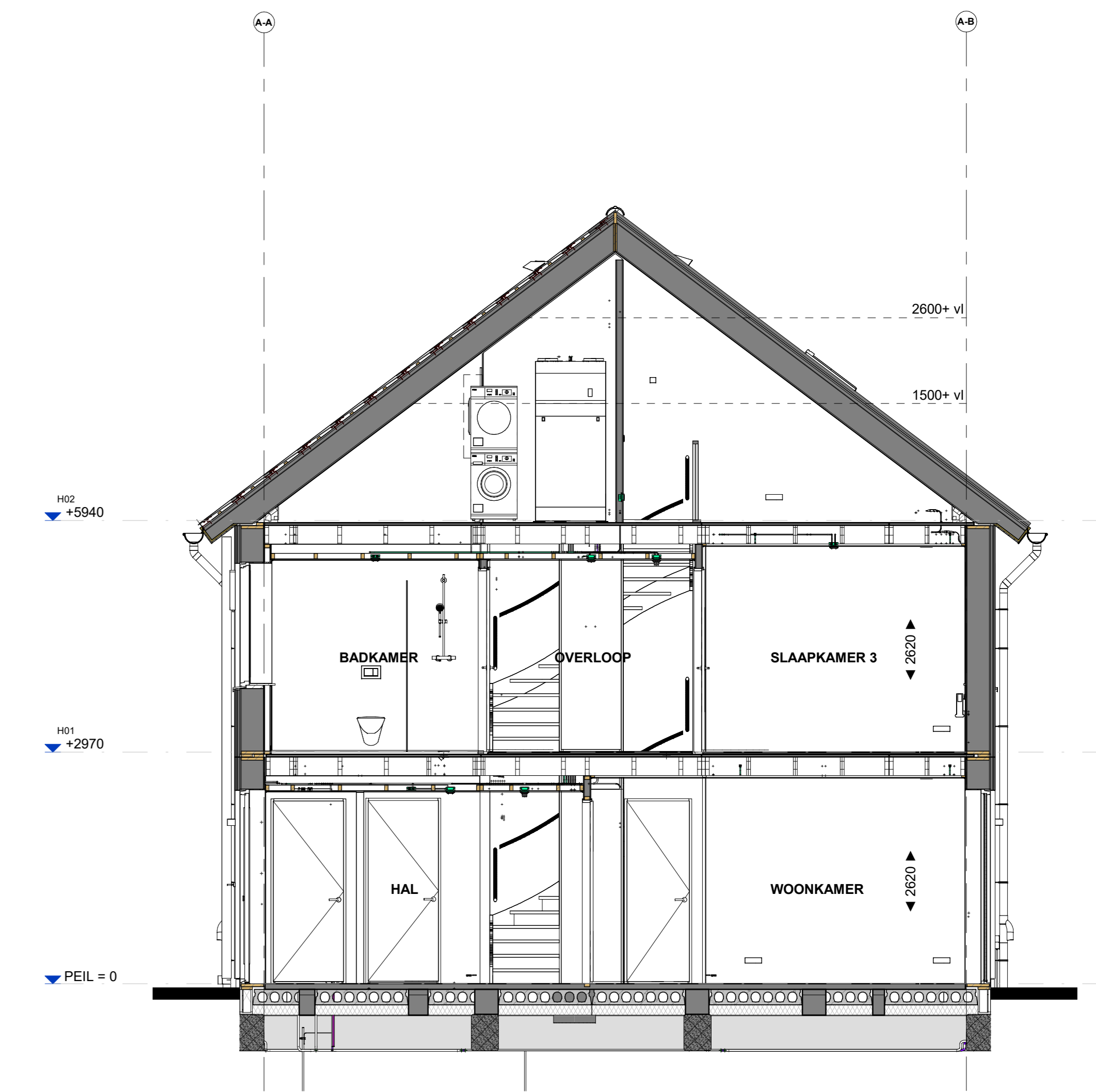
Doorsnede B515
