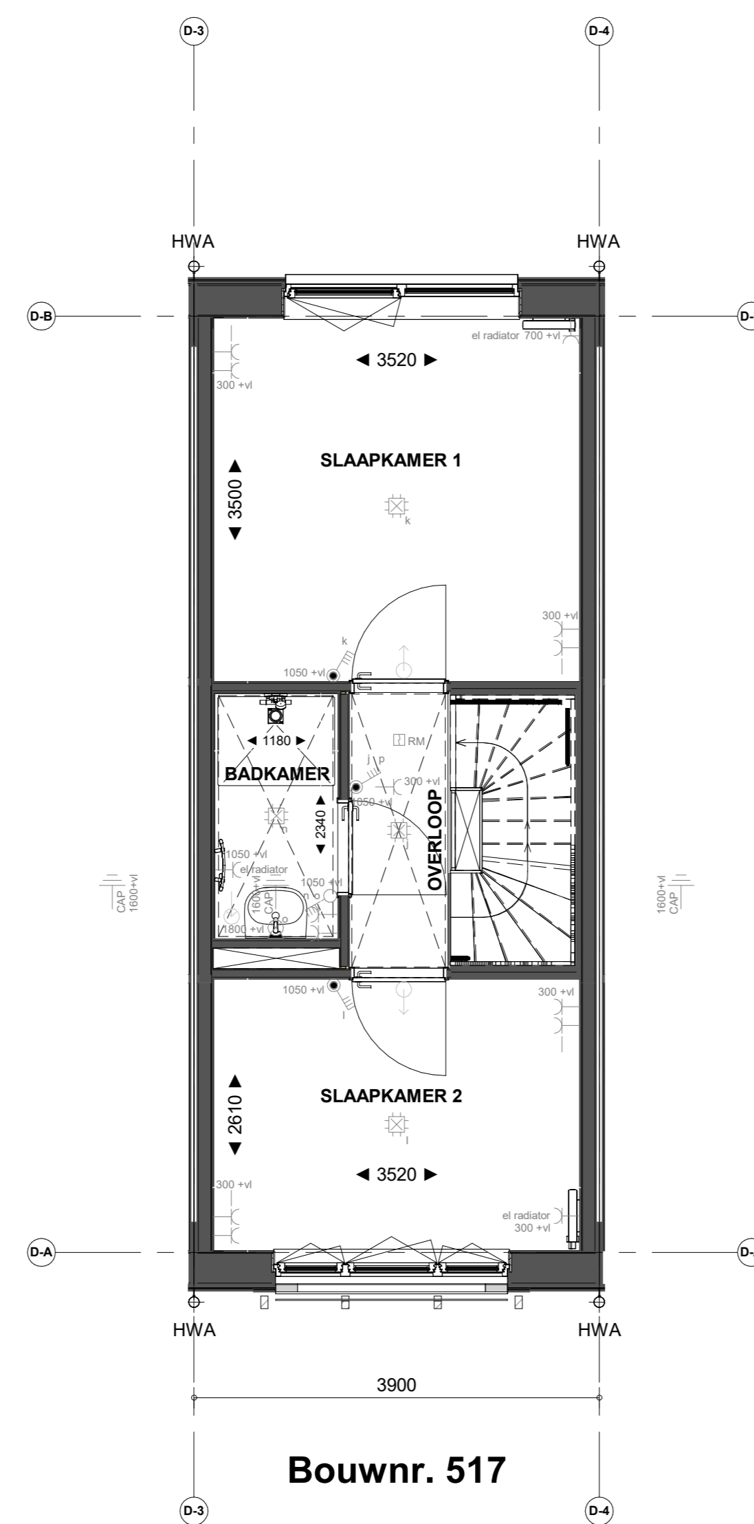
1e verdieping
