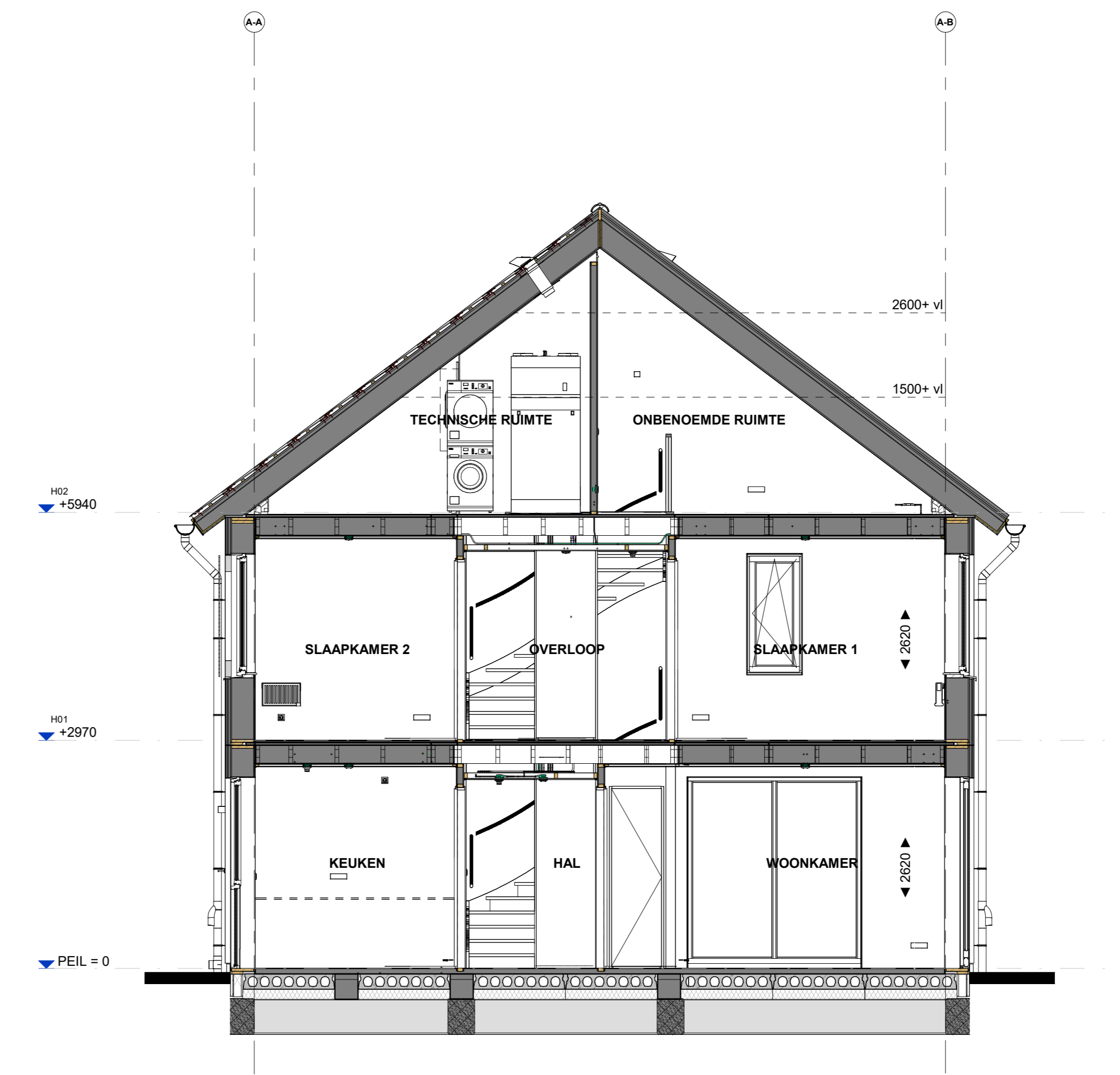
Doorsnede B517
