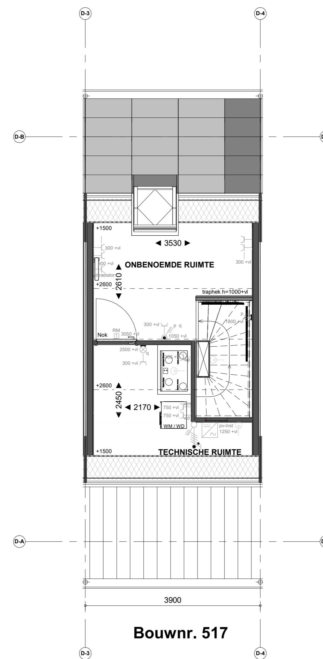
2e verdieping
