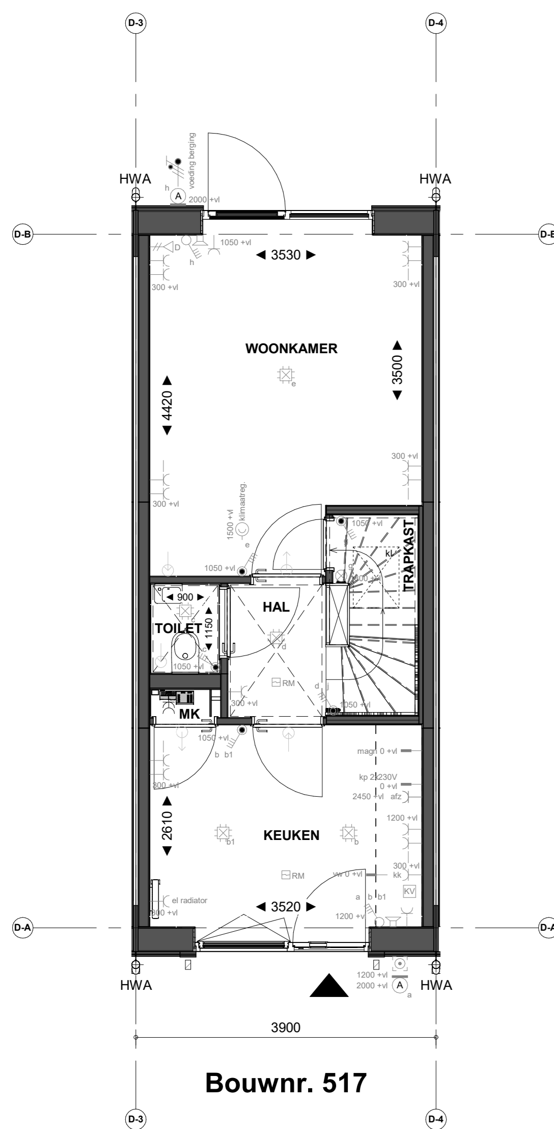
Begane grond
