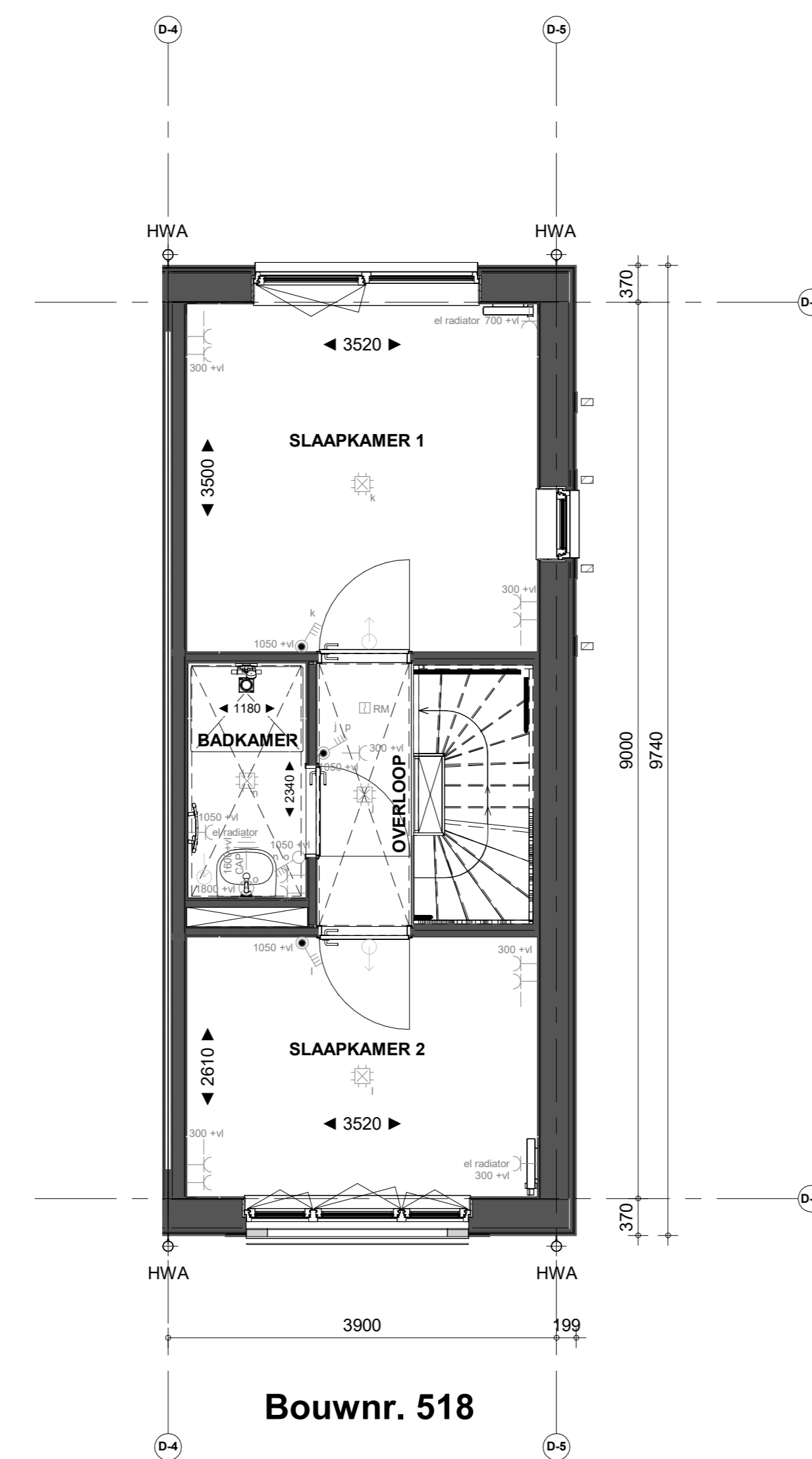
1e verdieping
