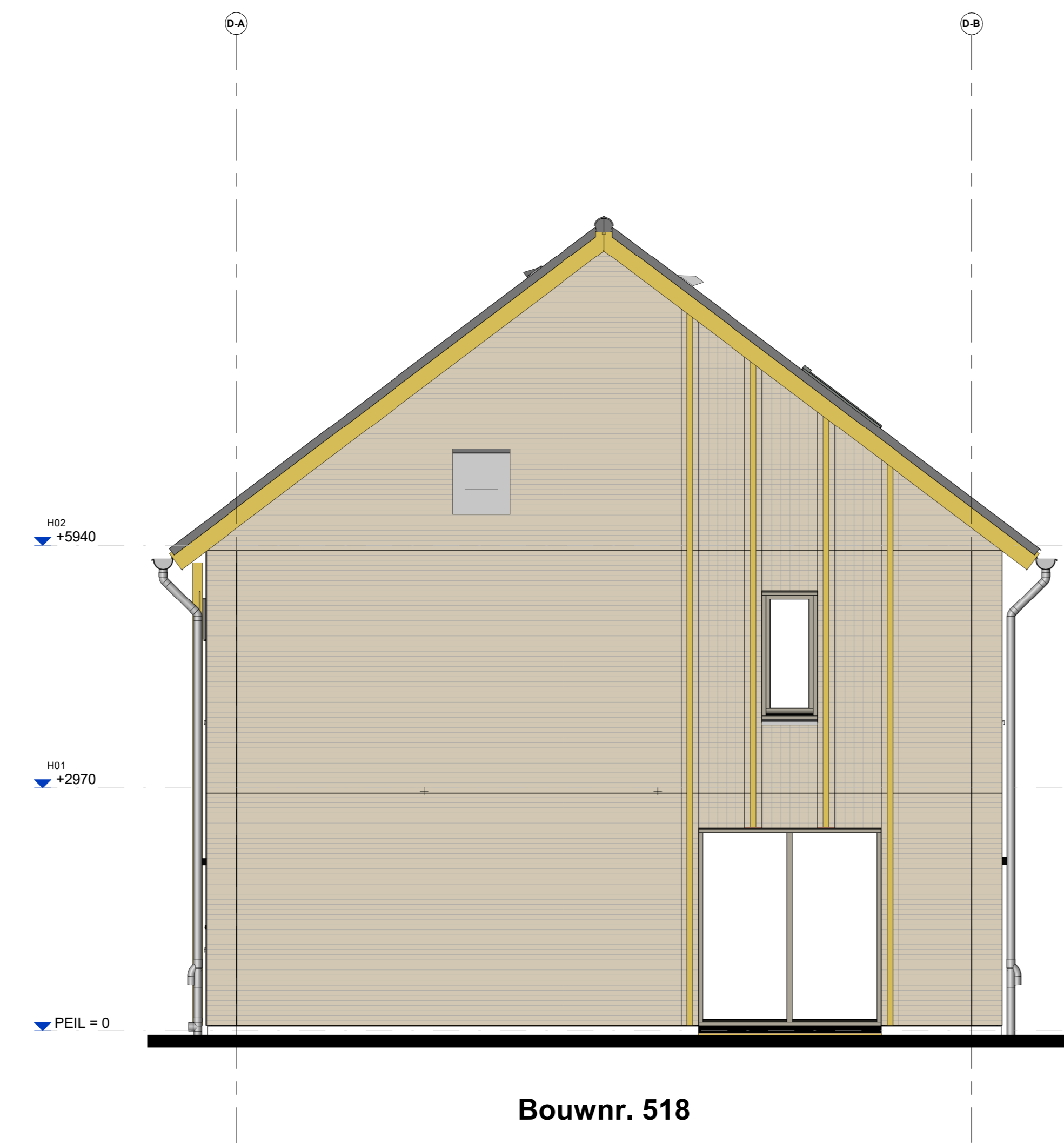
Rechter zijgevel
