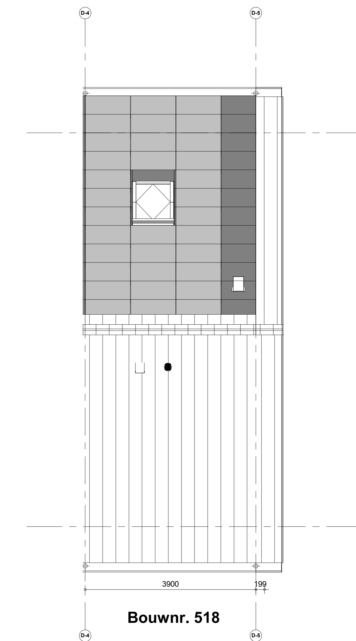
Dakaanzicht
