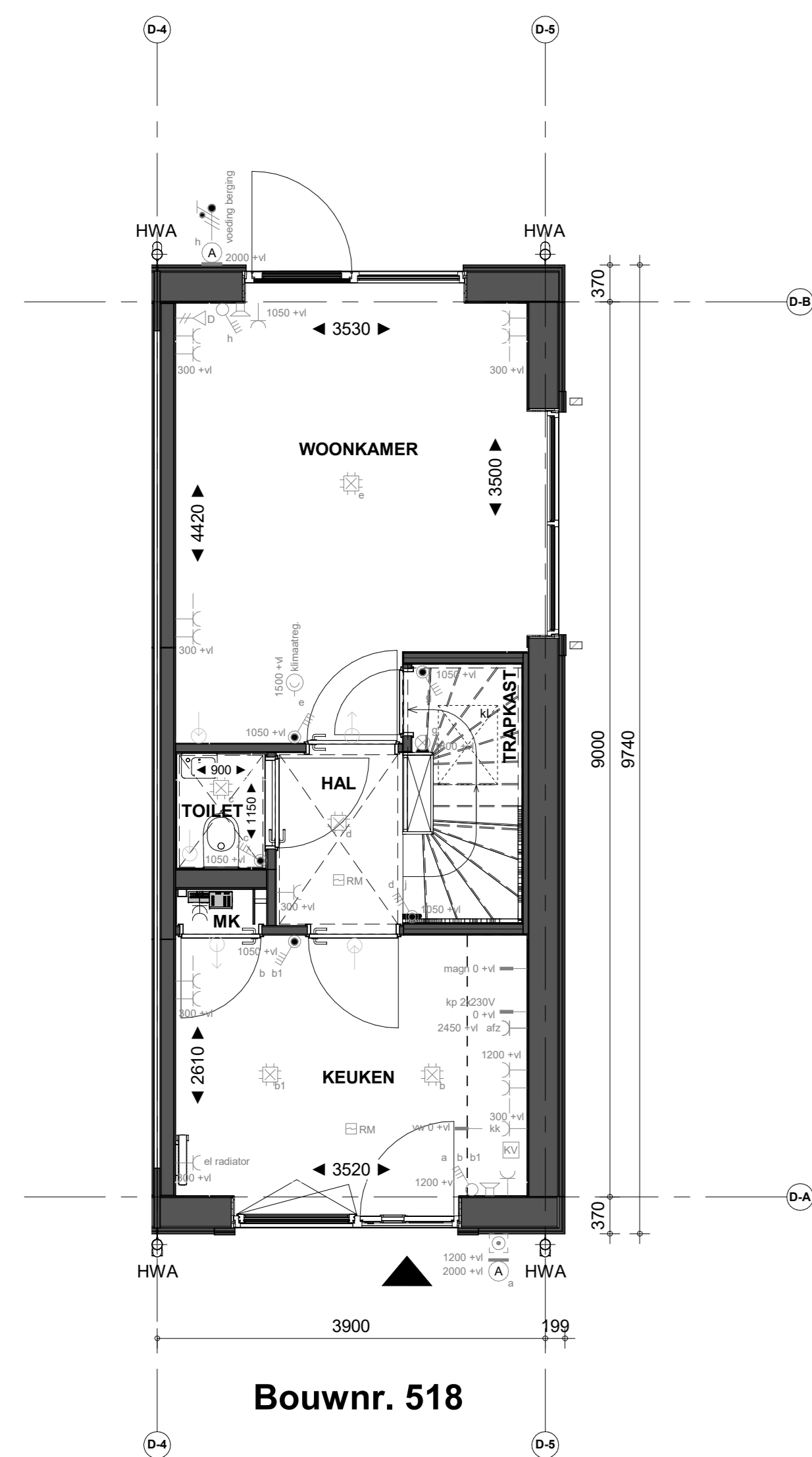
Begane grond
