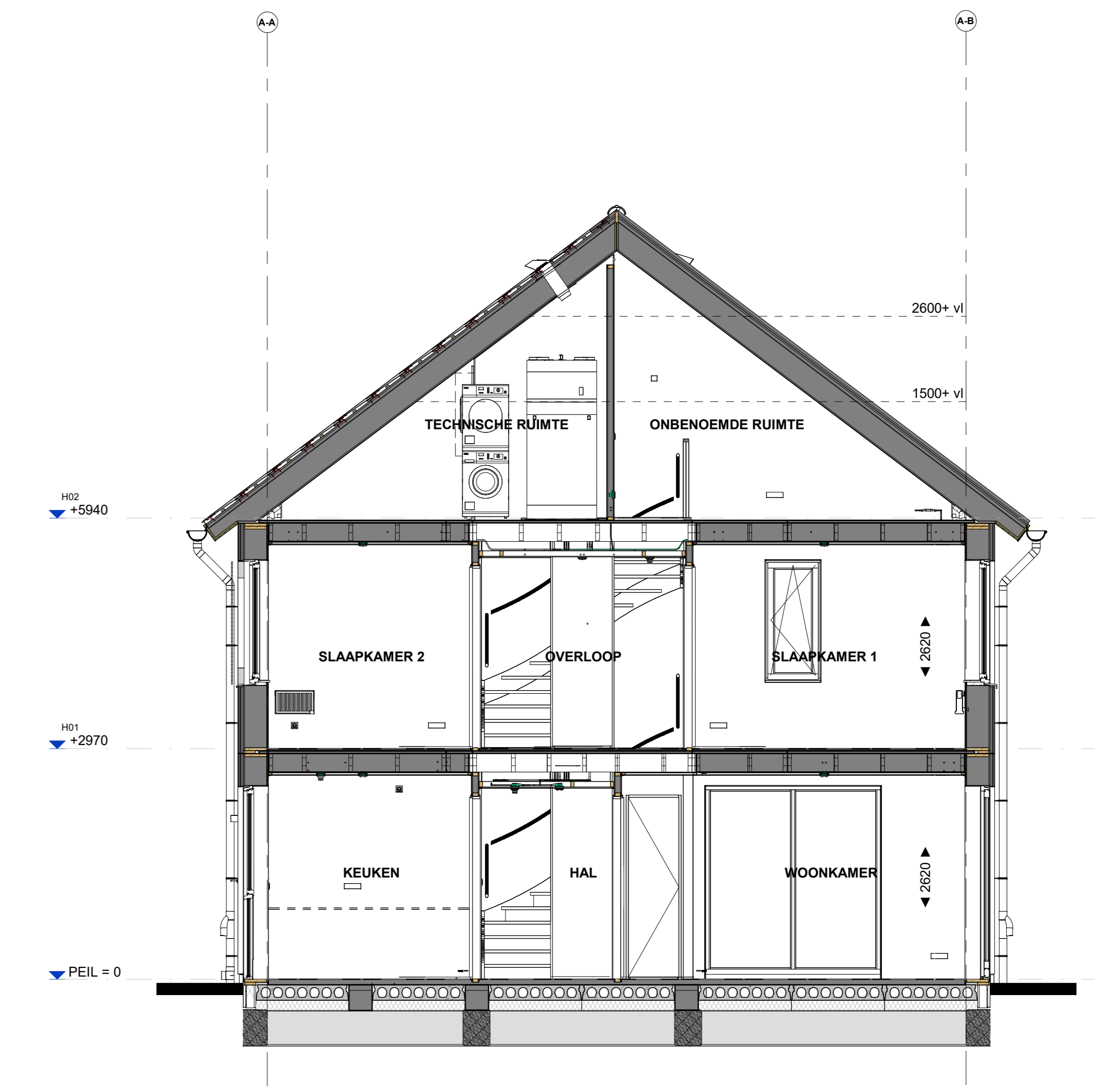
Doorsnede B518
