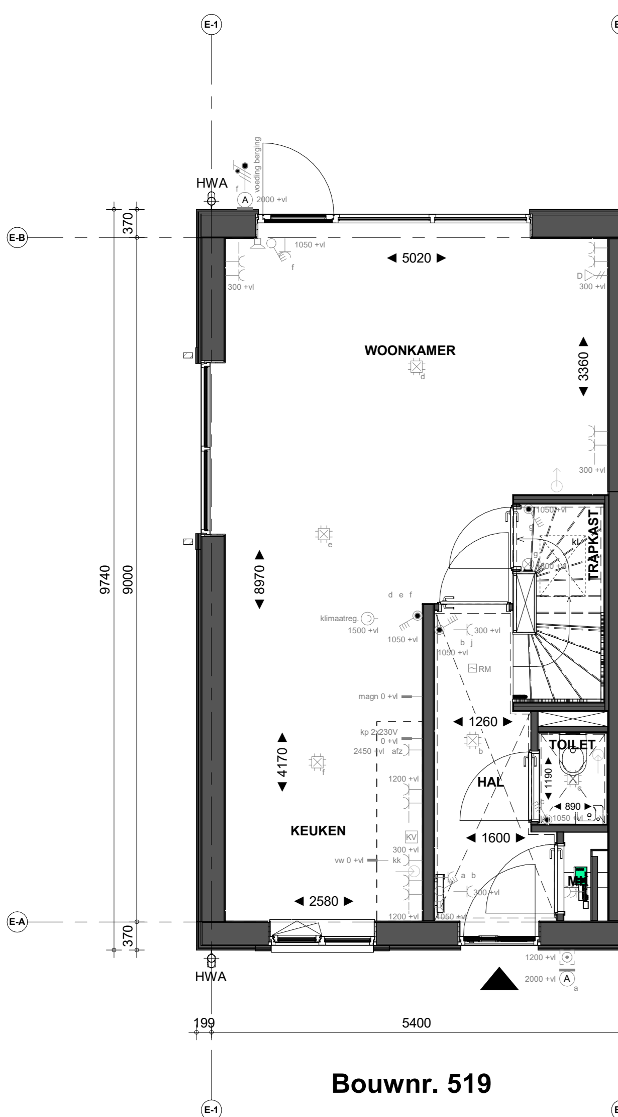
Begane grond
