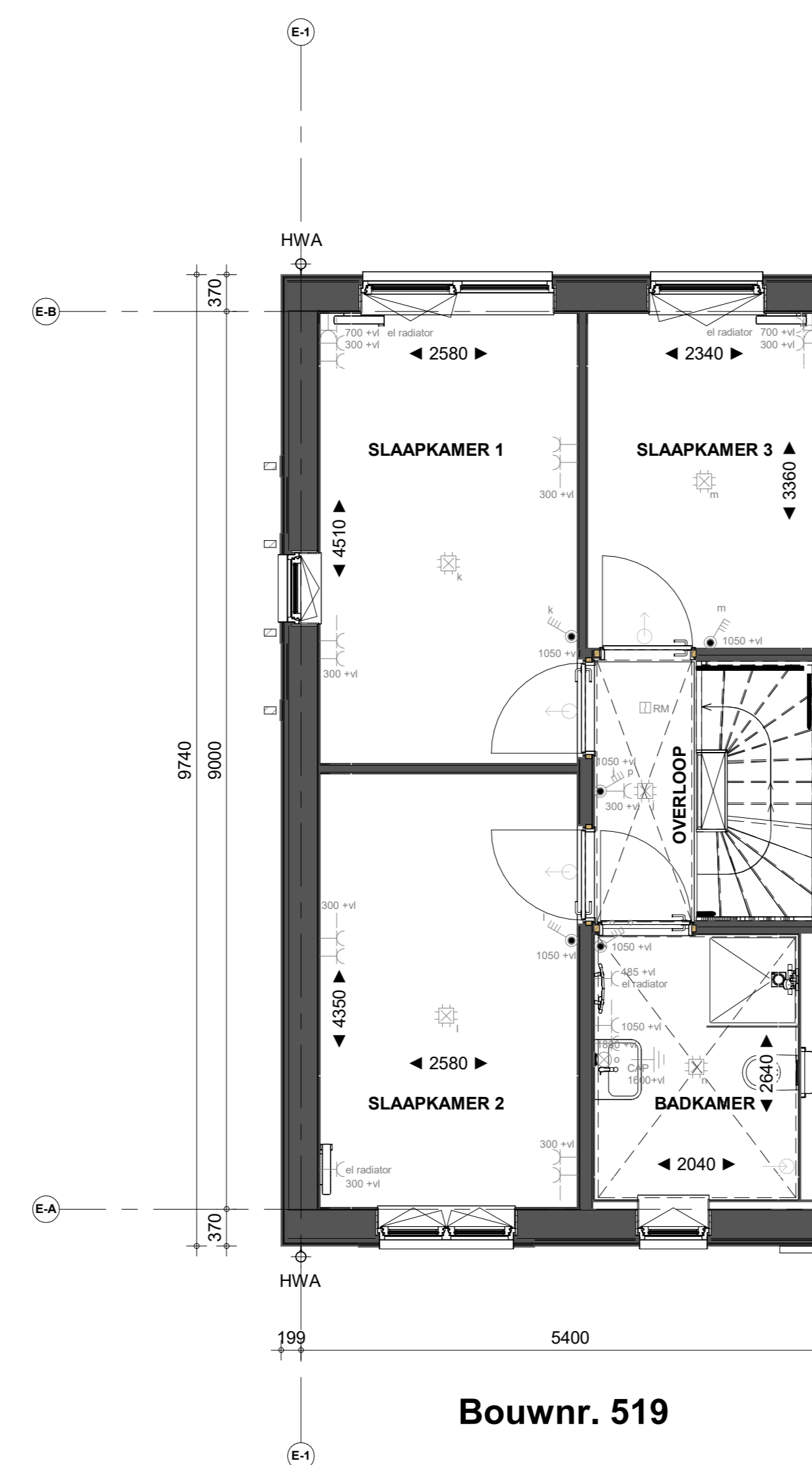
1e verdieping
