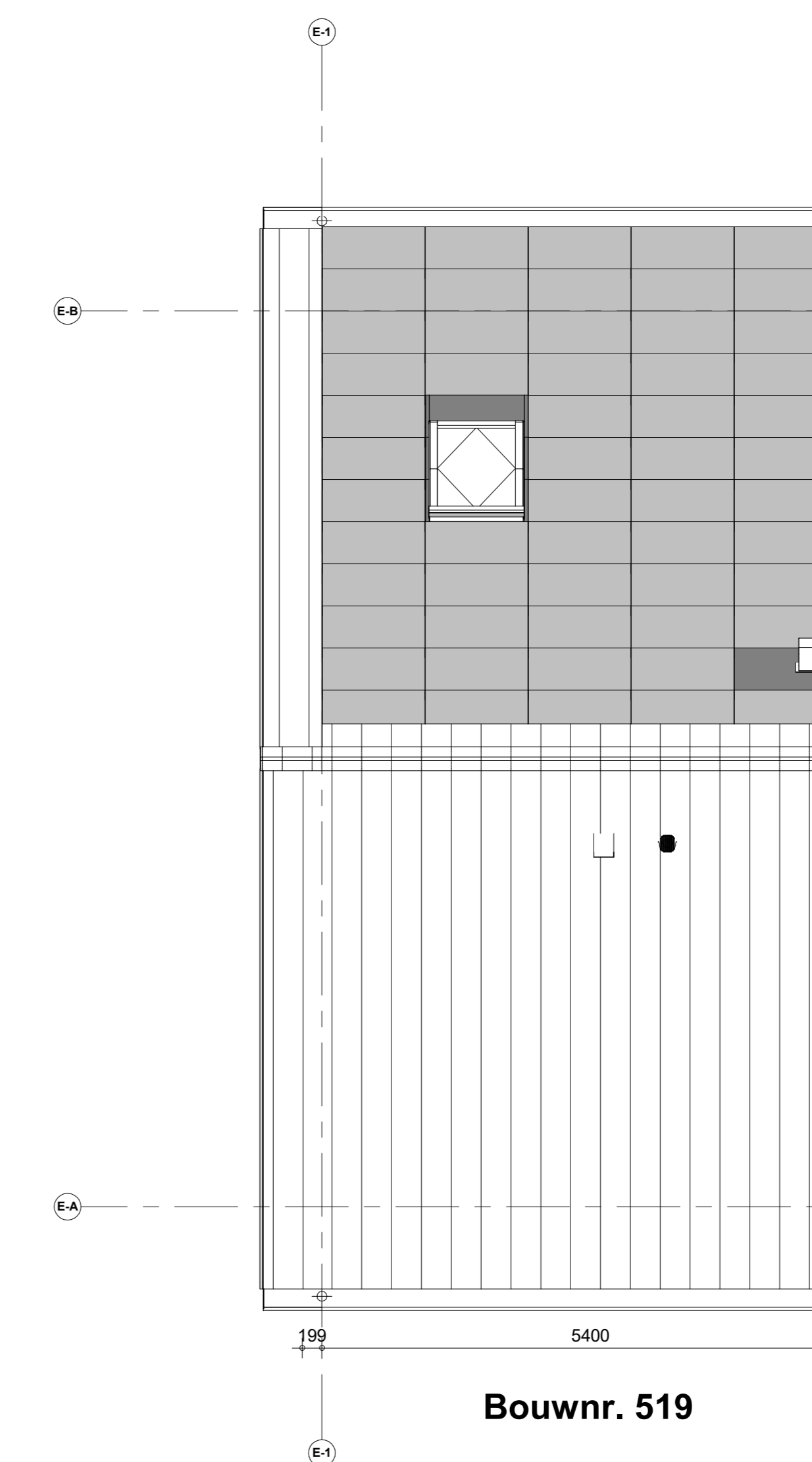
Dakaanzicht
