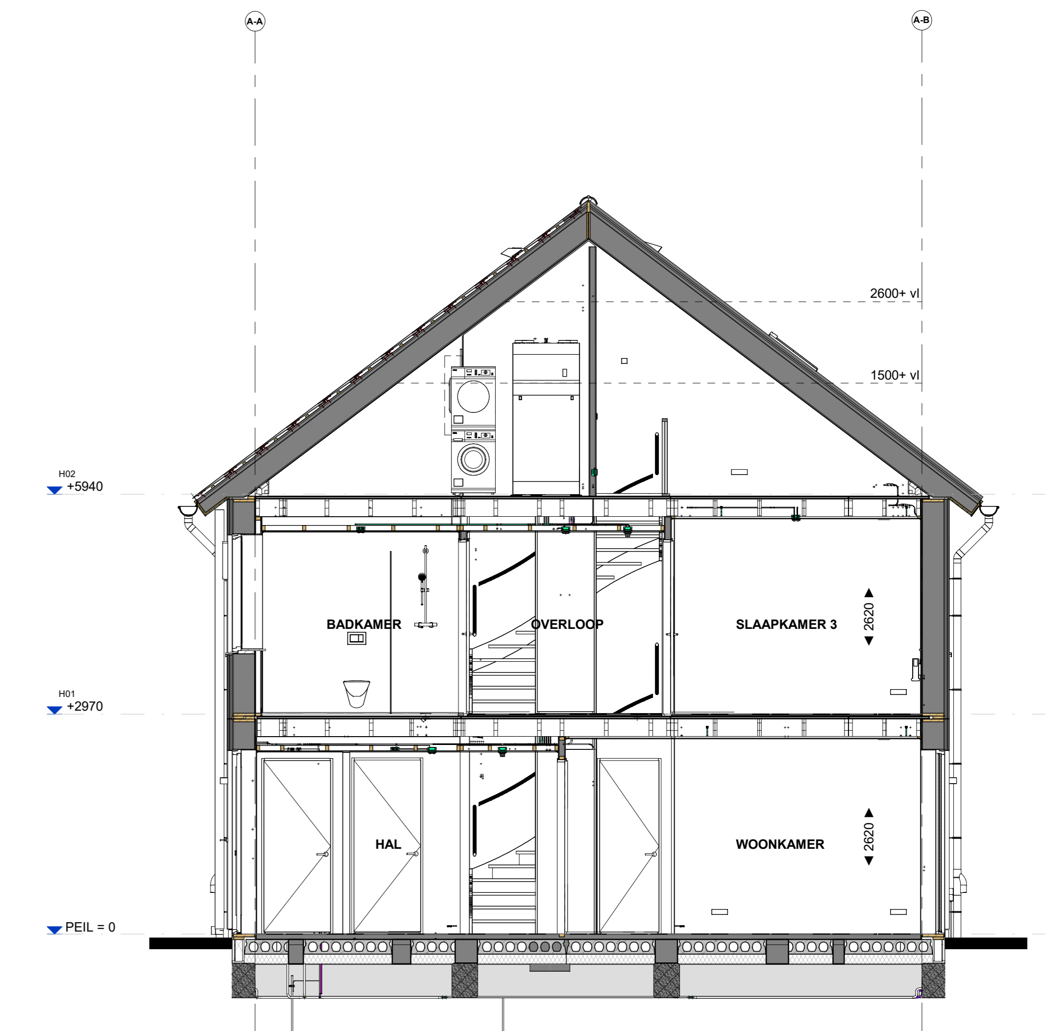
Doorsnede B519
