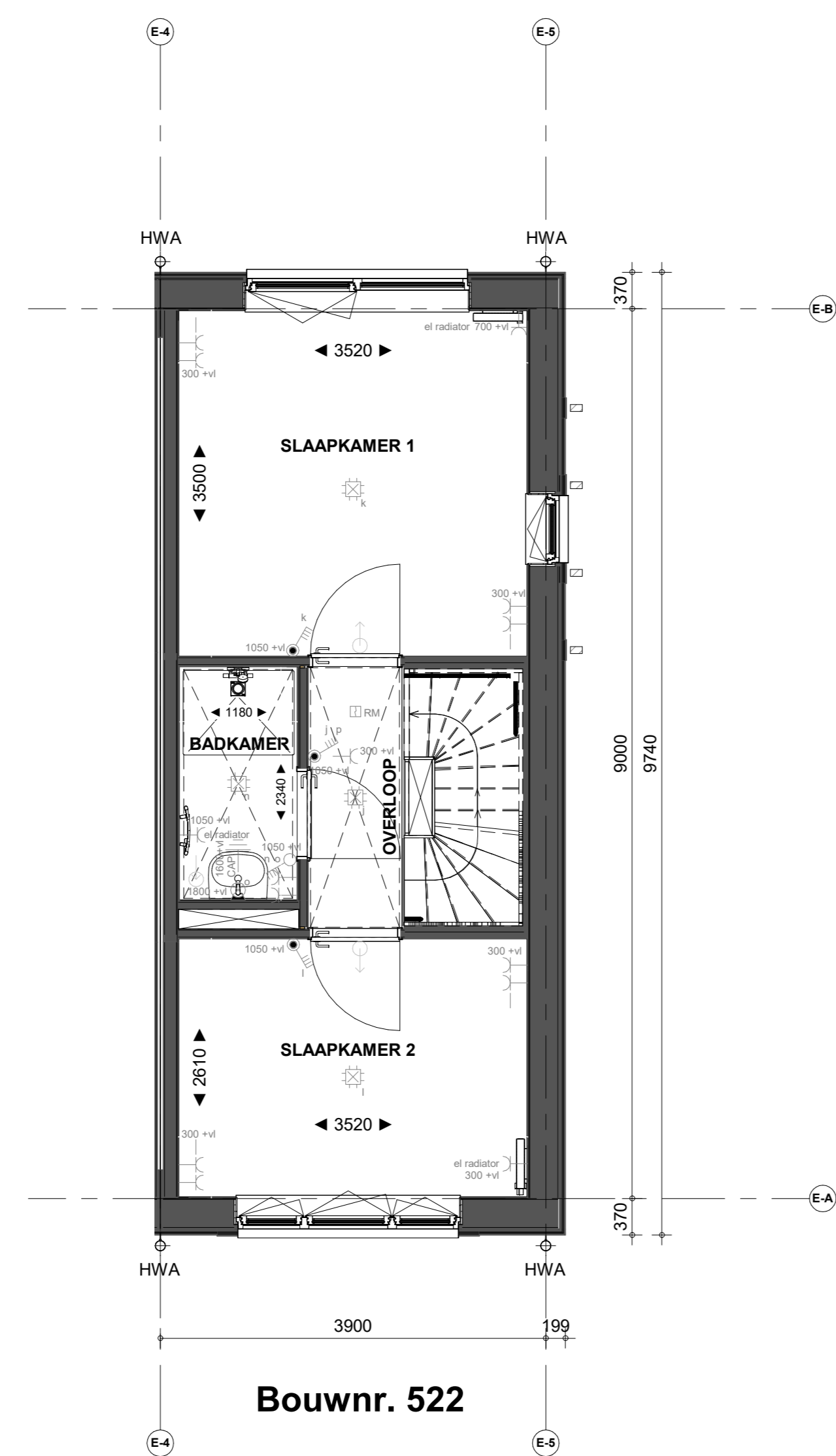
1e verdieping
