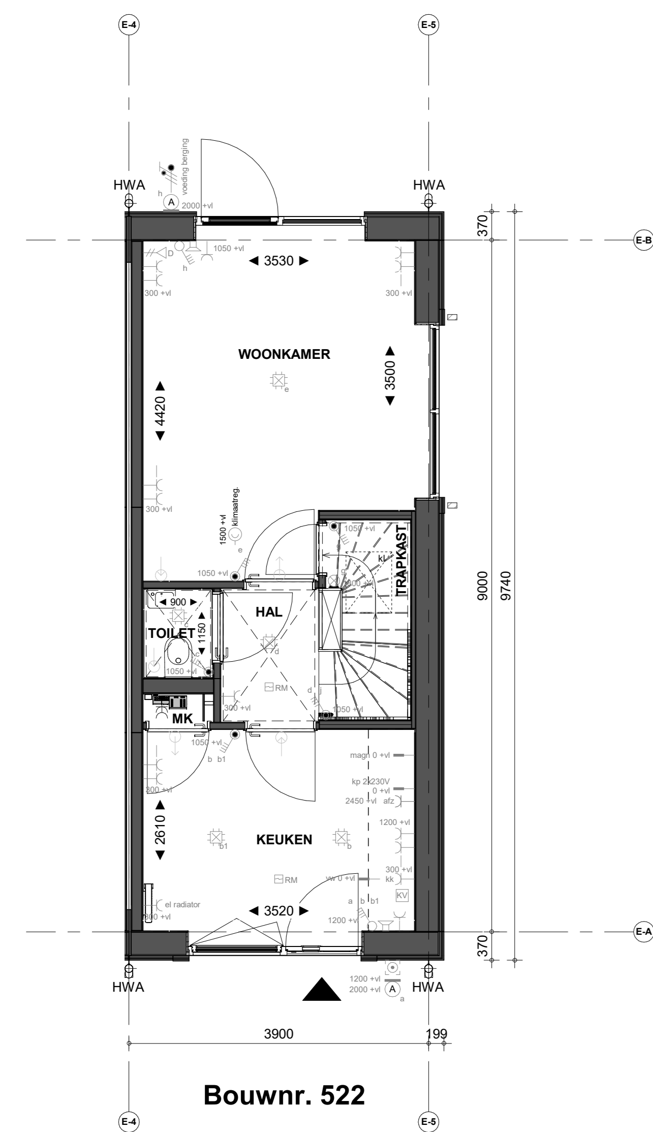
Begane grond
