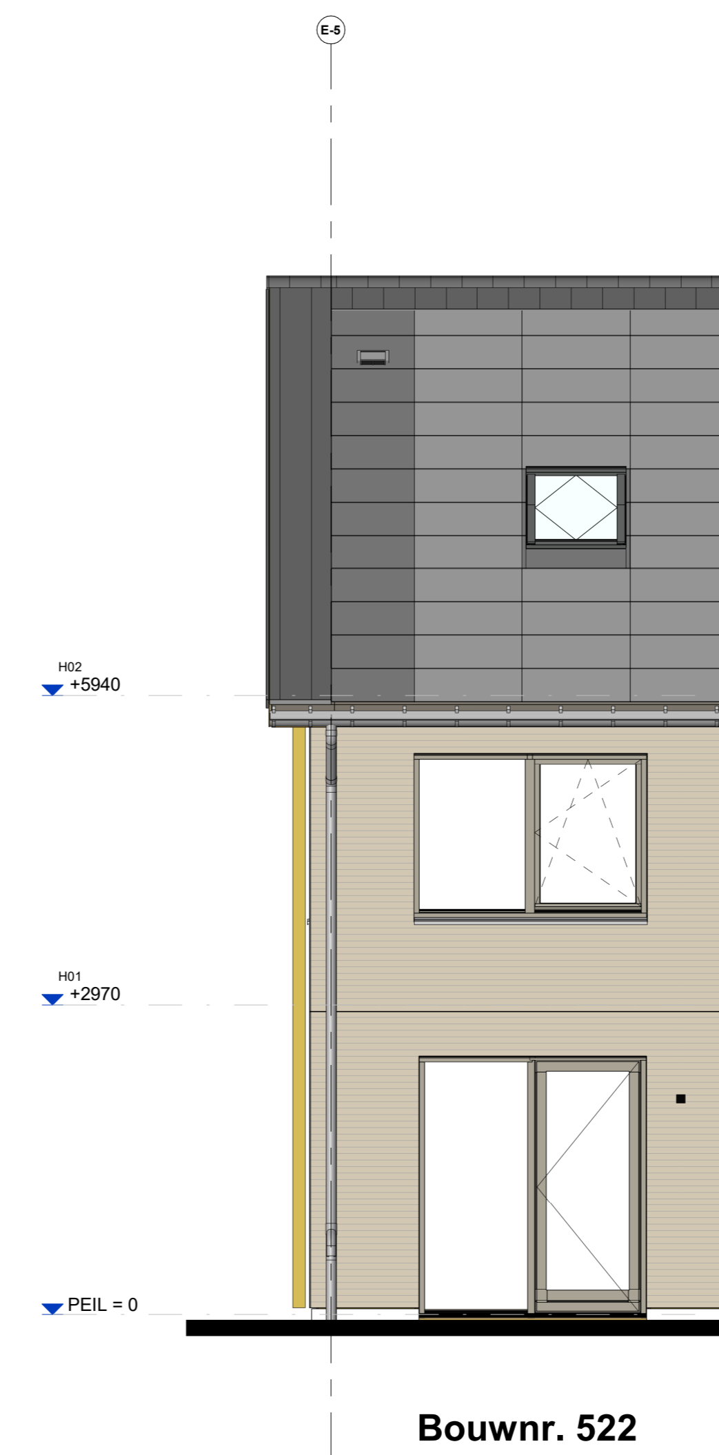
Achtergevel
