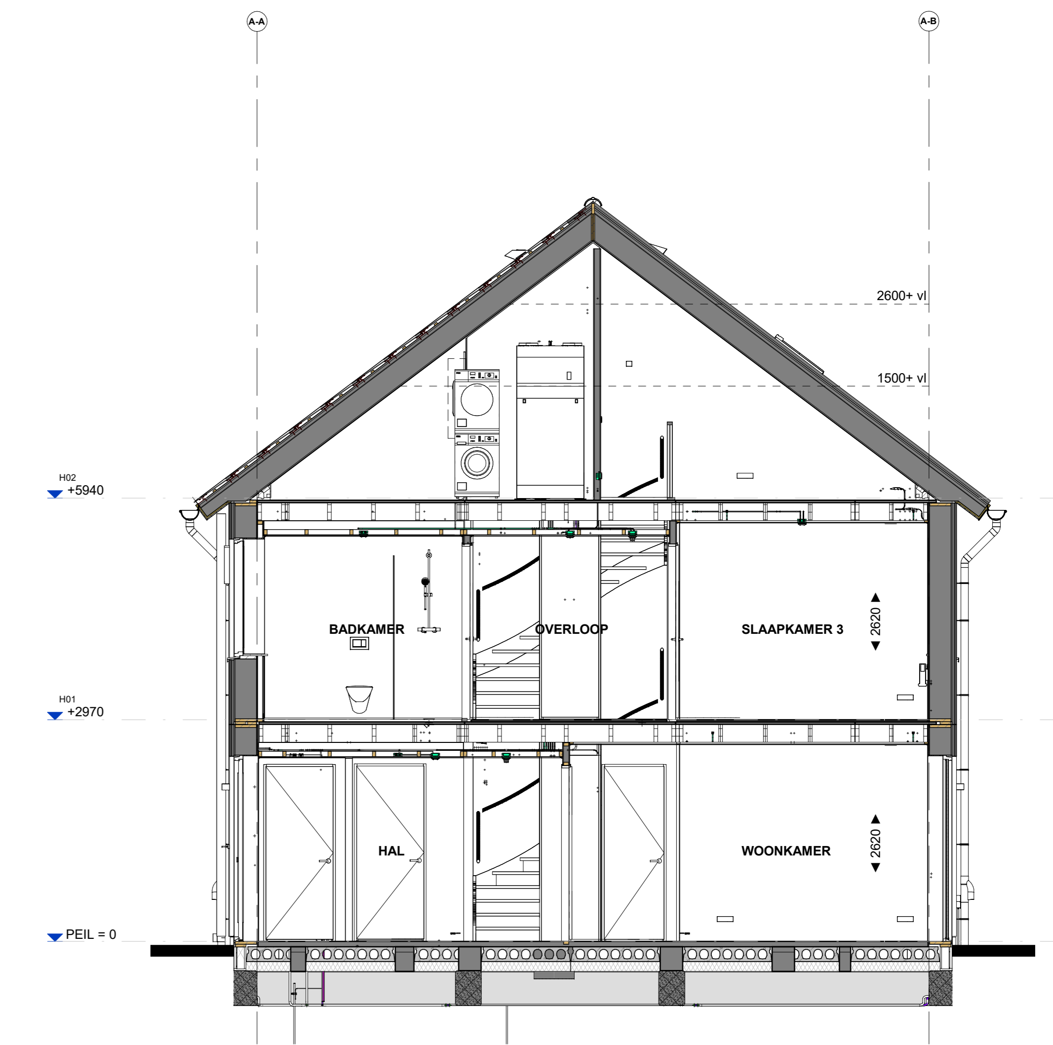
Doorsnede B523
