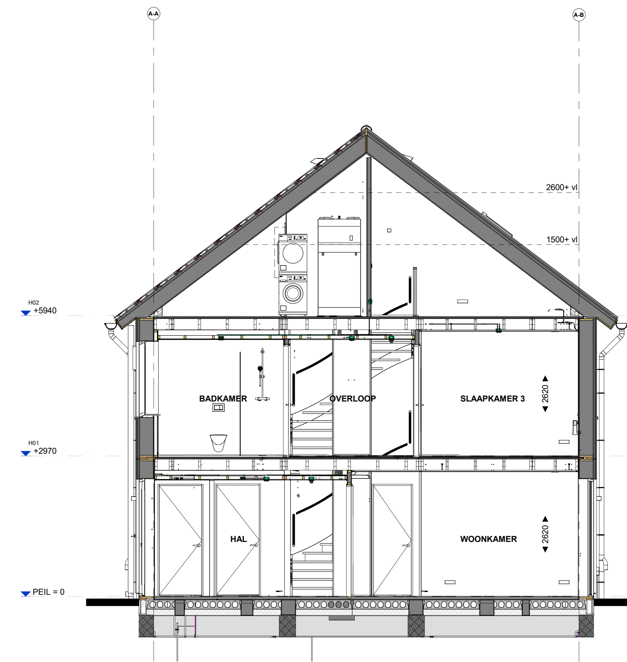
Doorsnede B524
