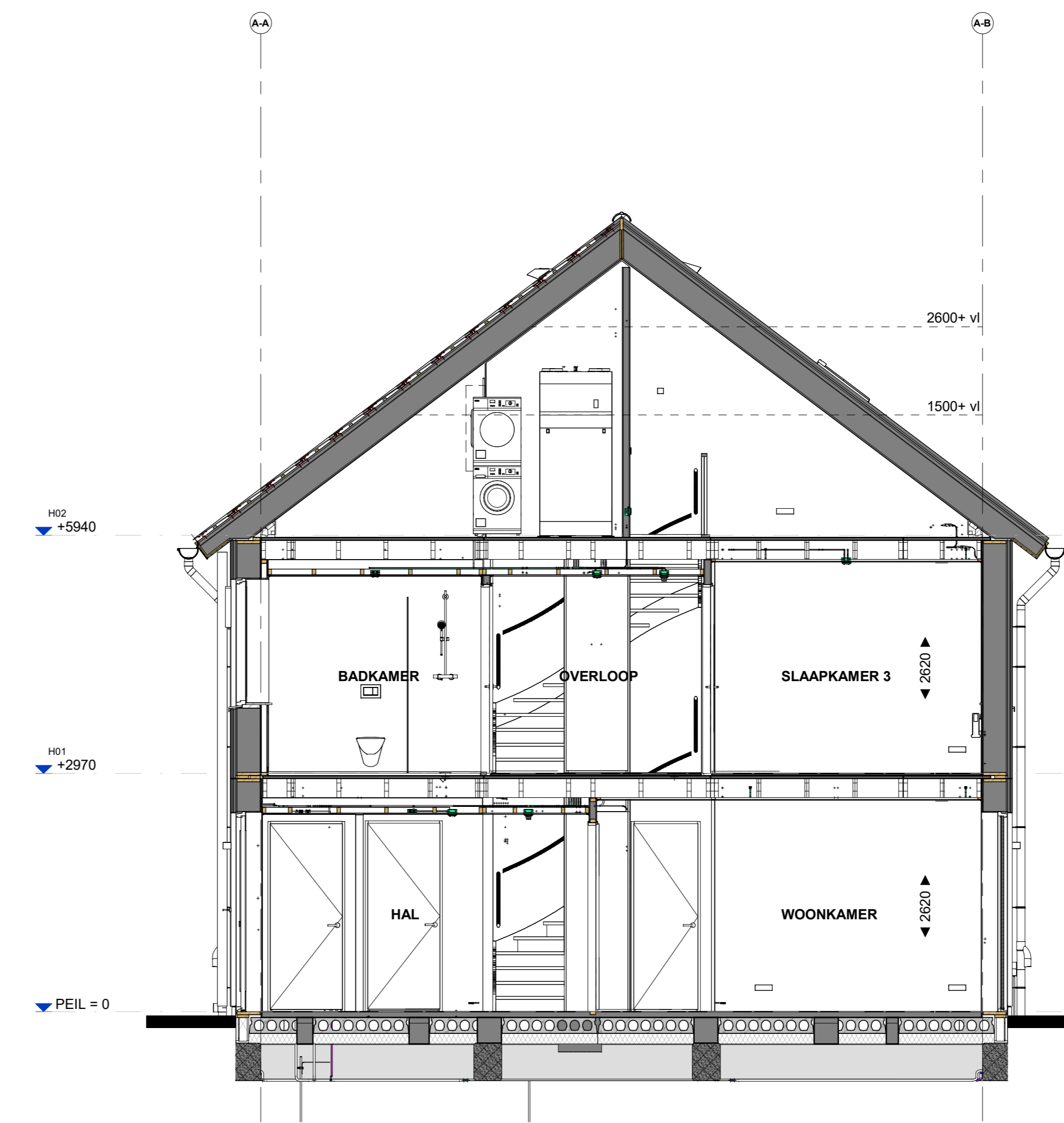
Doorsnede B525
