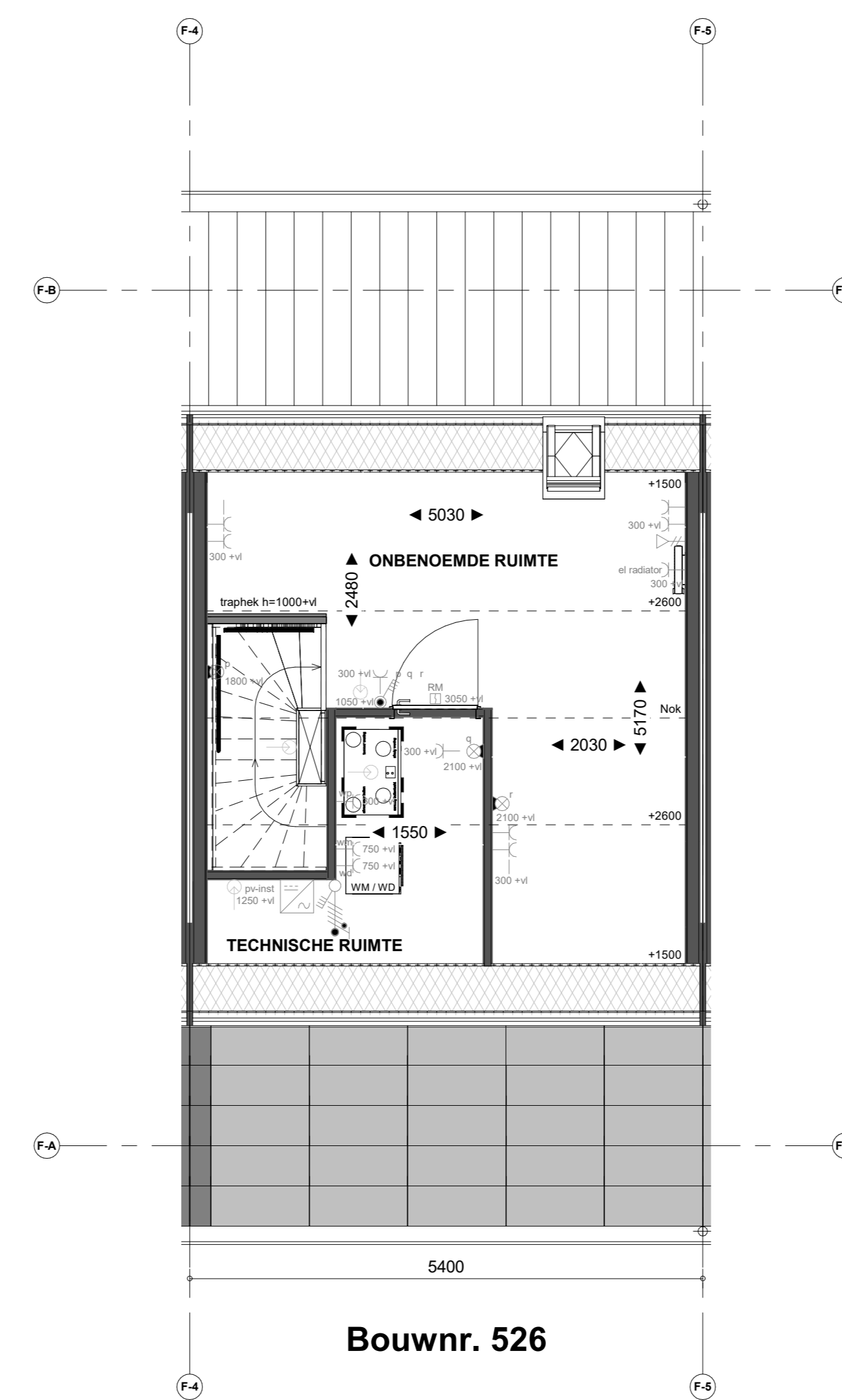
2e verdieping
