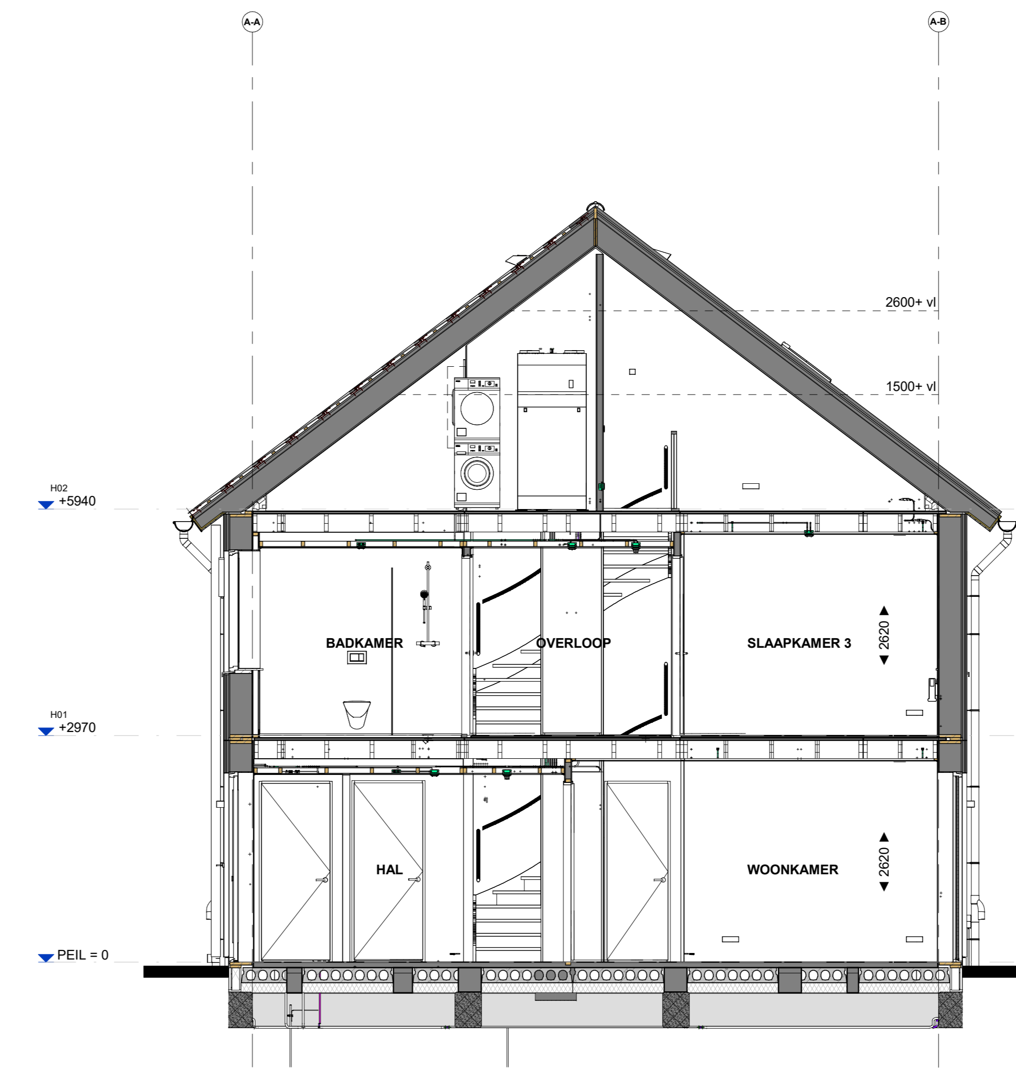
Doorsnede B526
