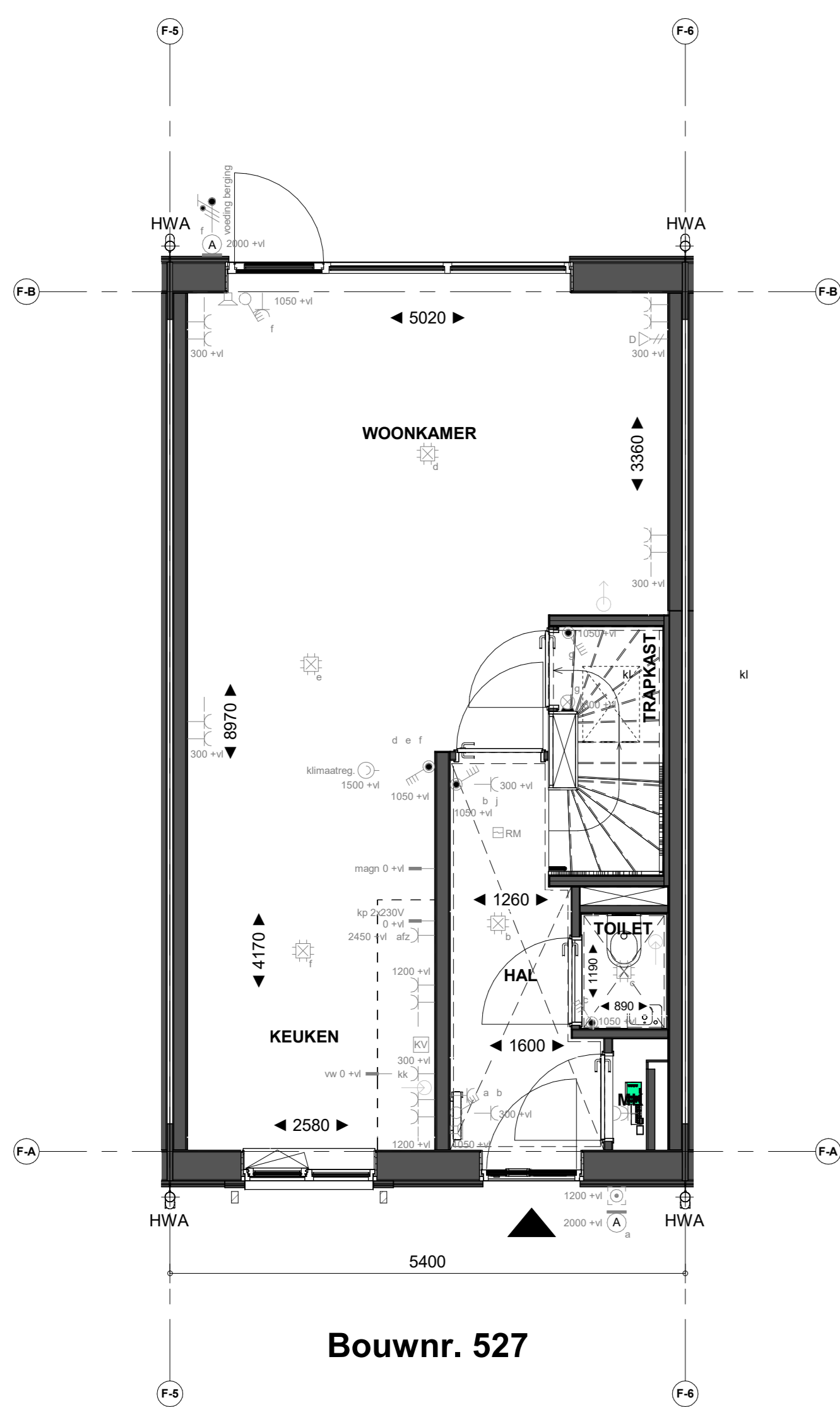
Begane grond
