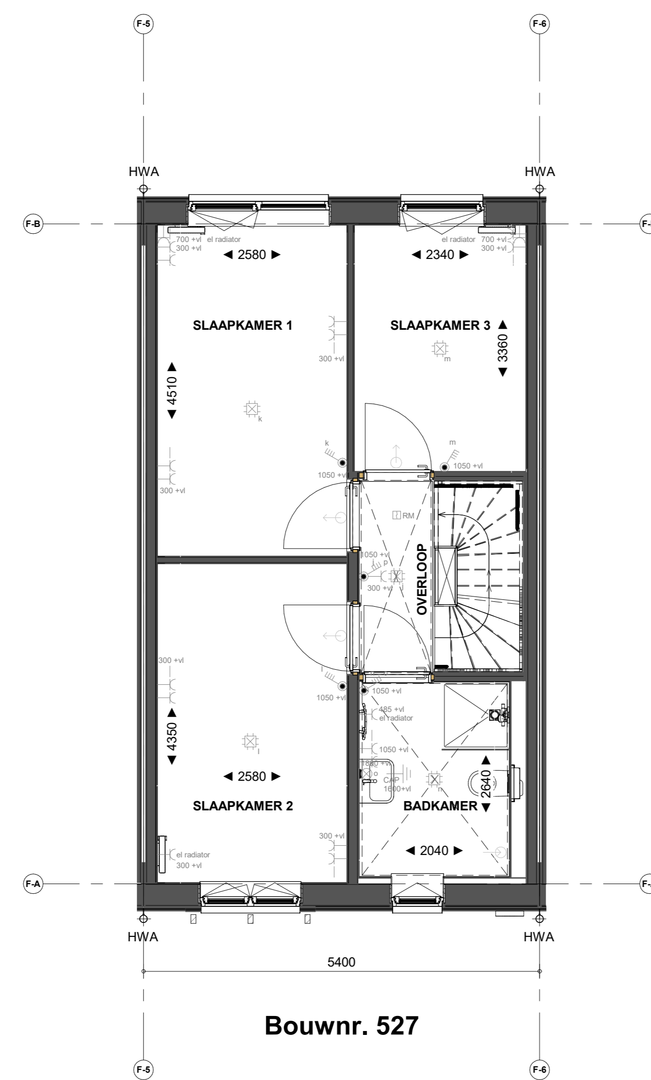
1e verdieping
