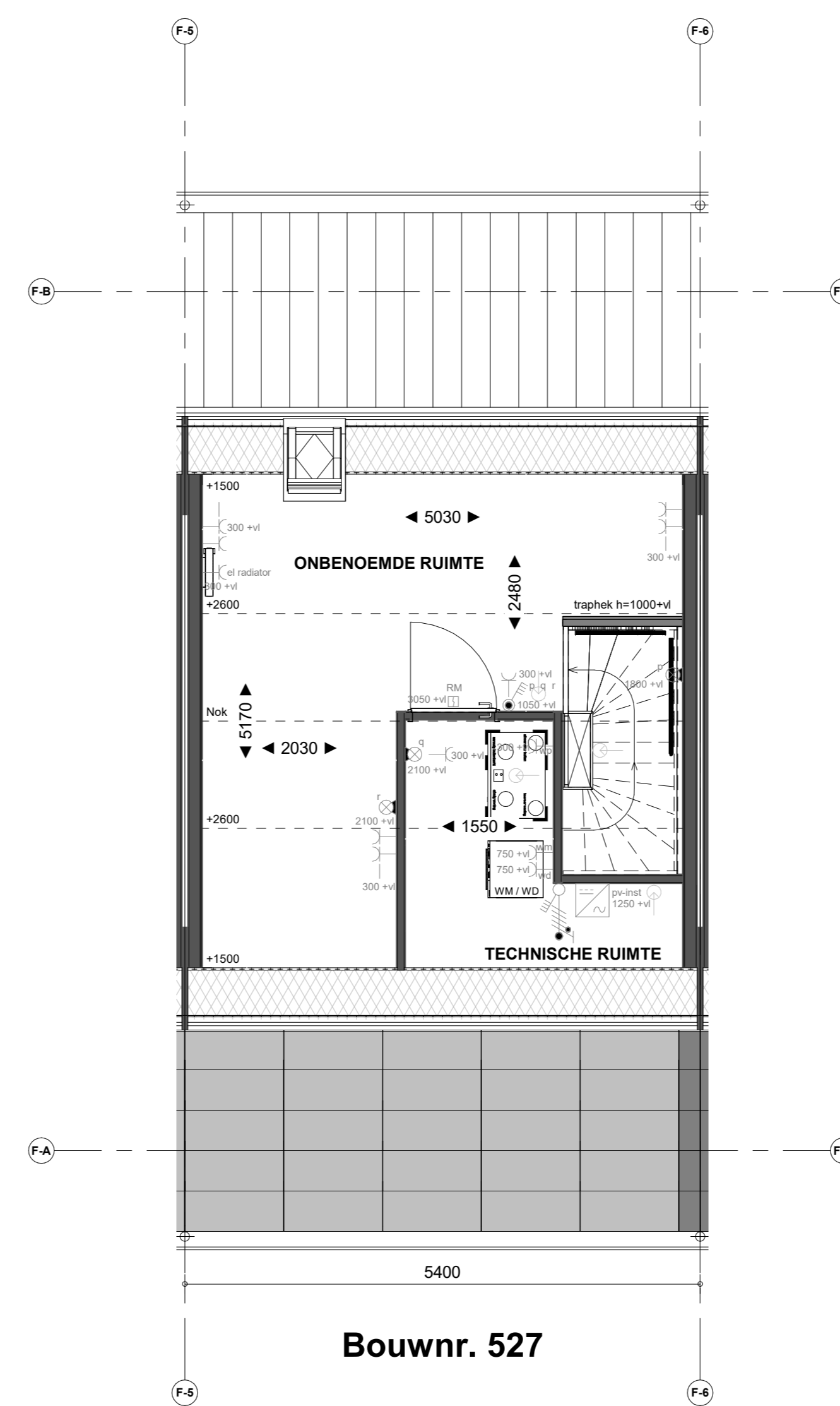
2e verdieping
