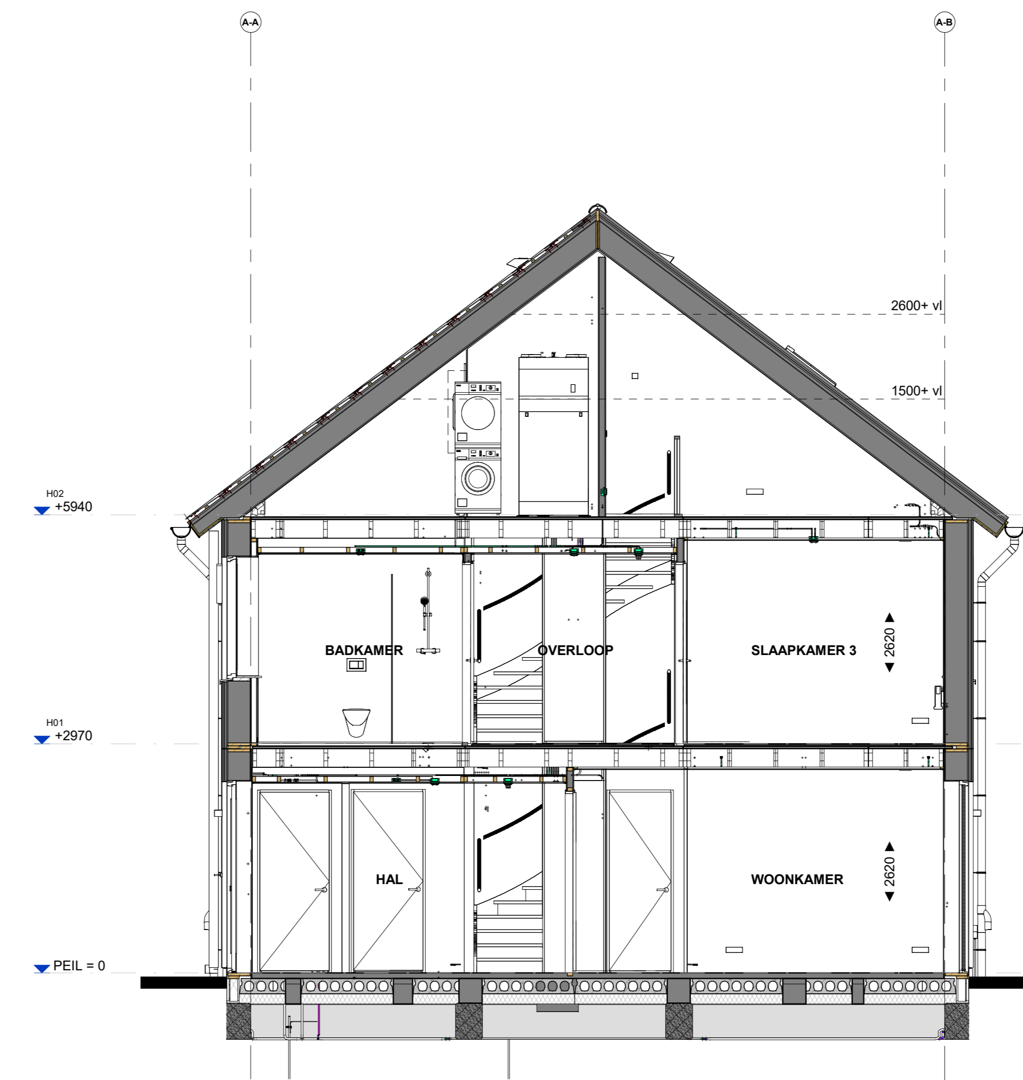
Doorsnede B527
