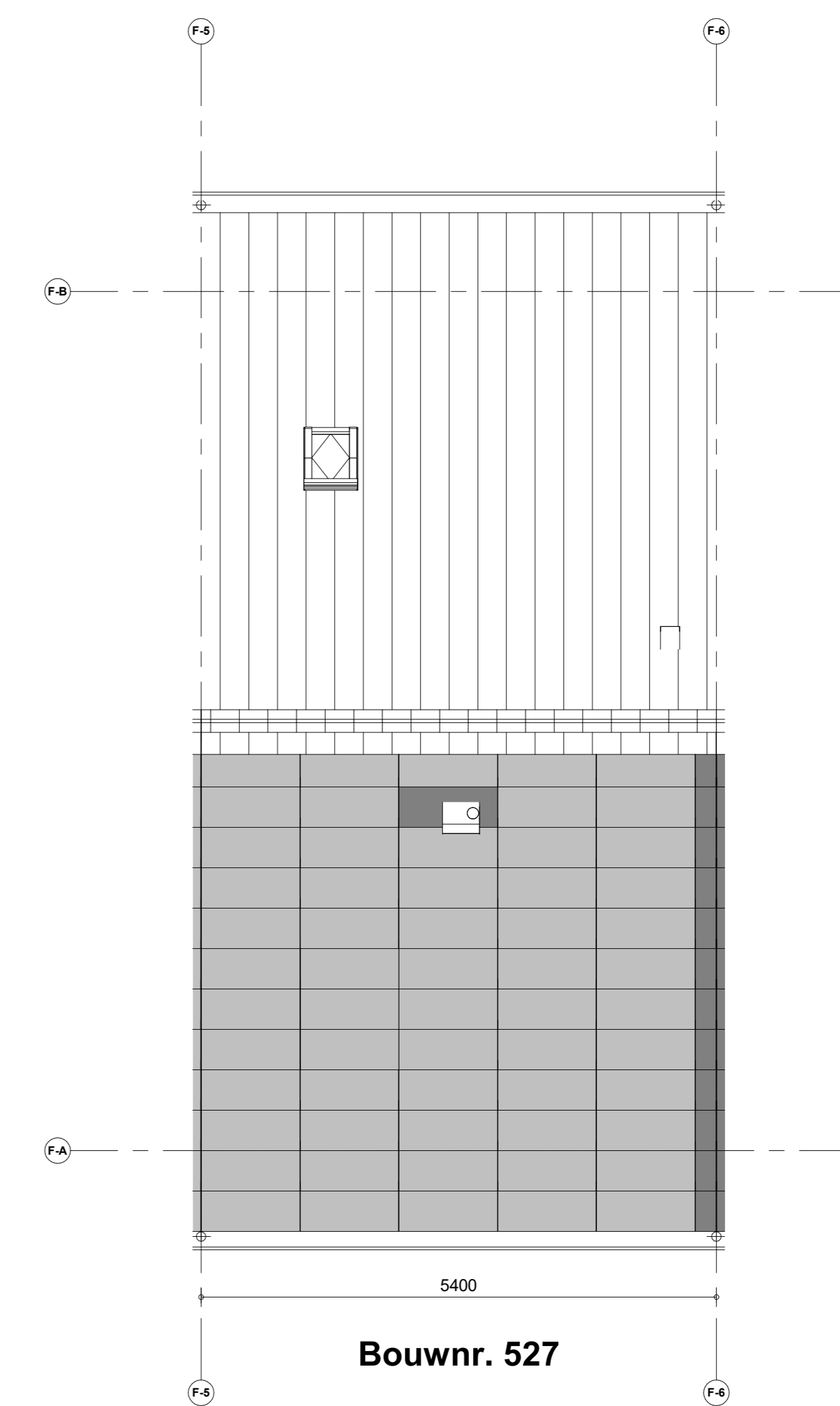
Dakaanzicht
