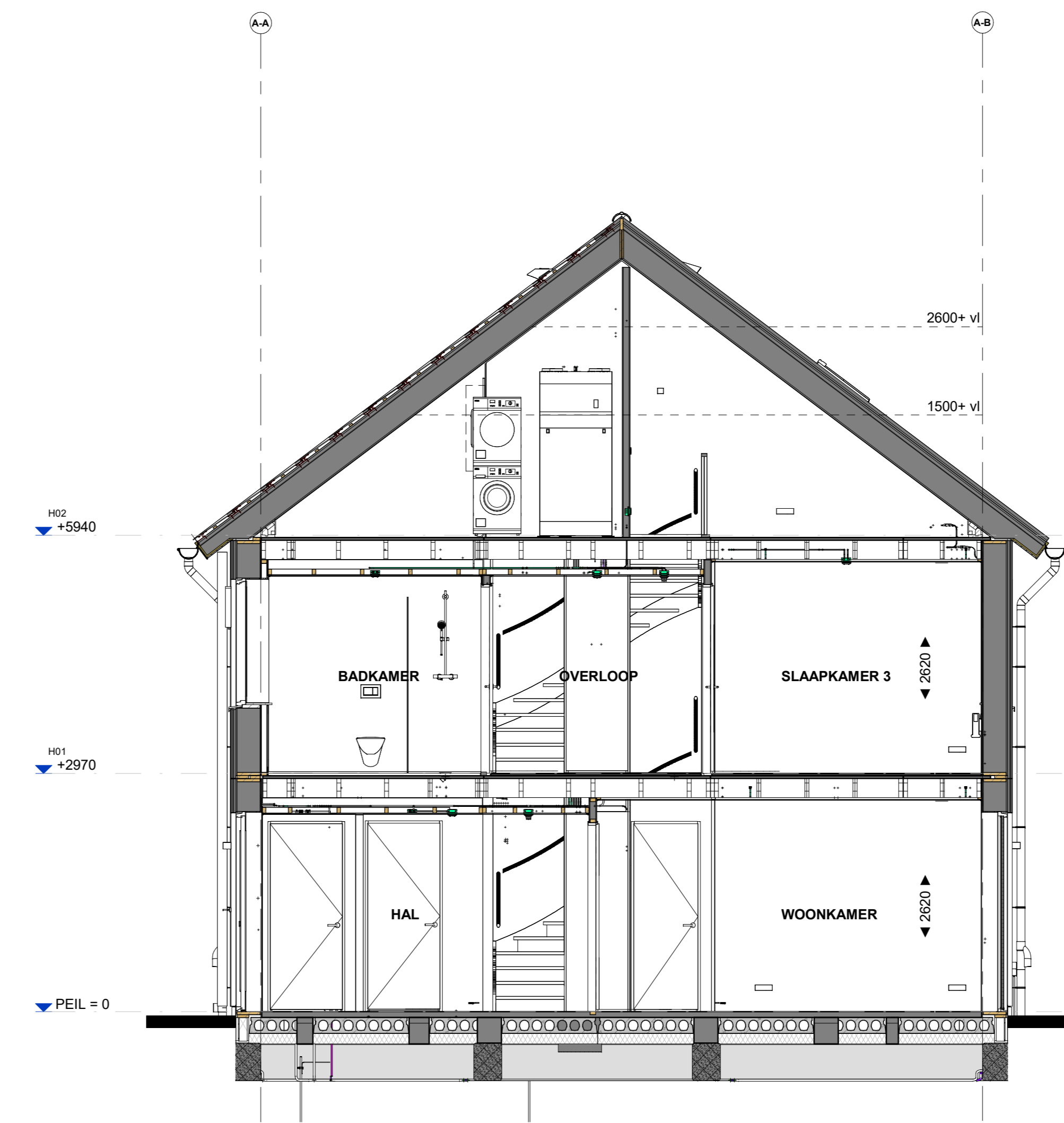
Doorsnede B528
