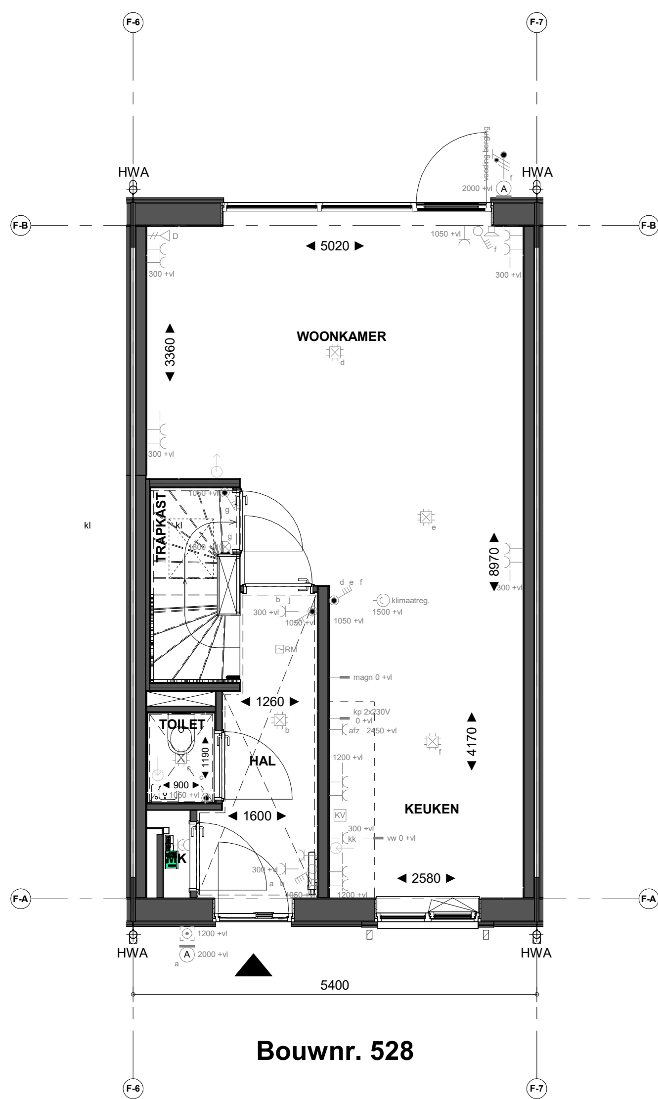
Begane grond
