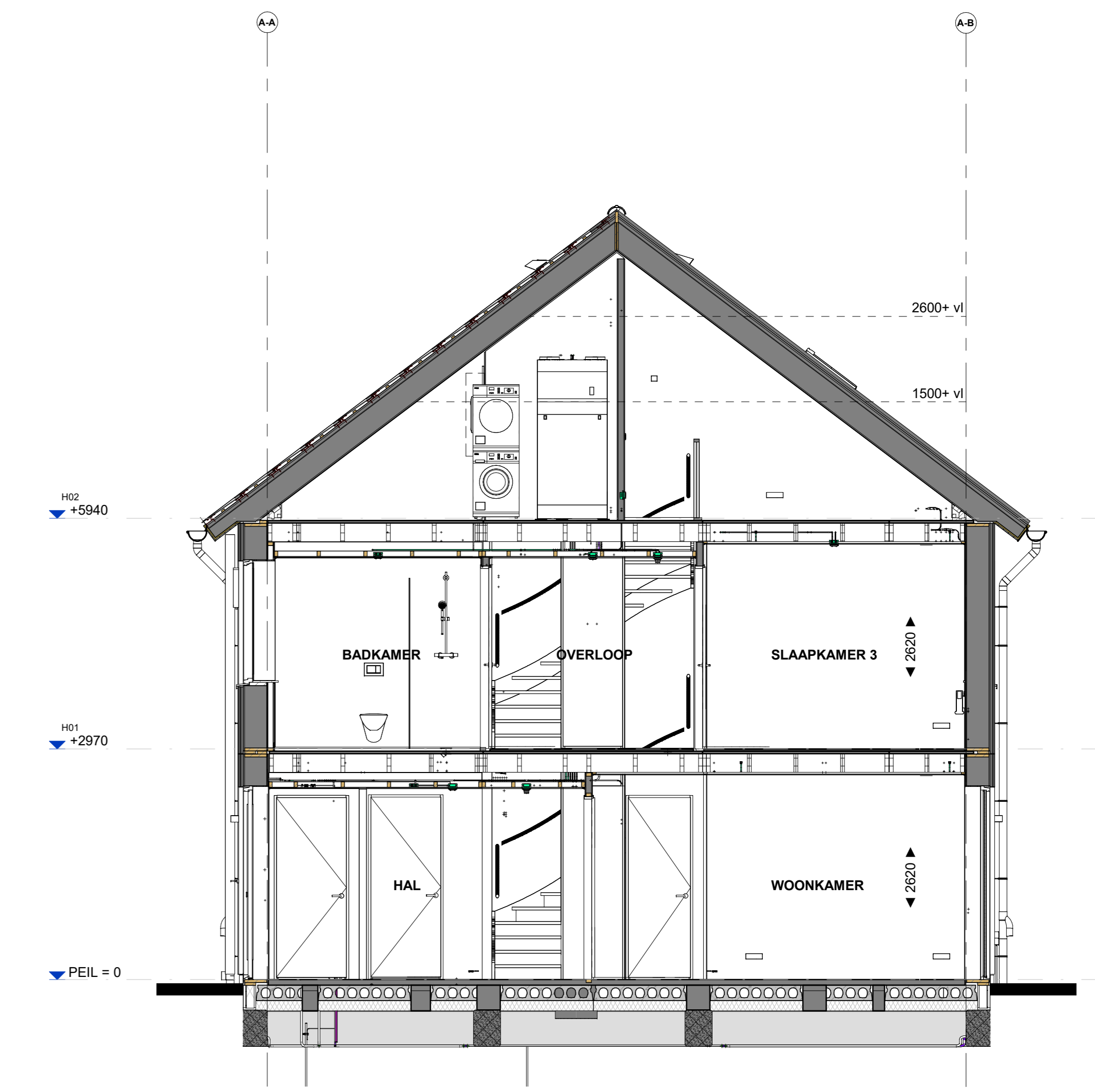
Doorsnede B530
