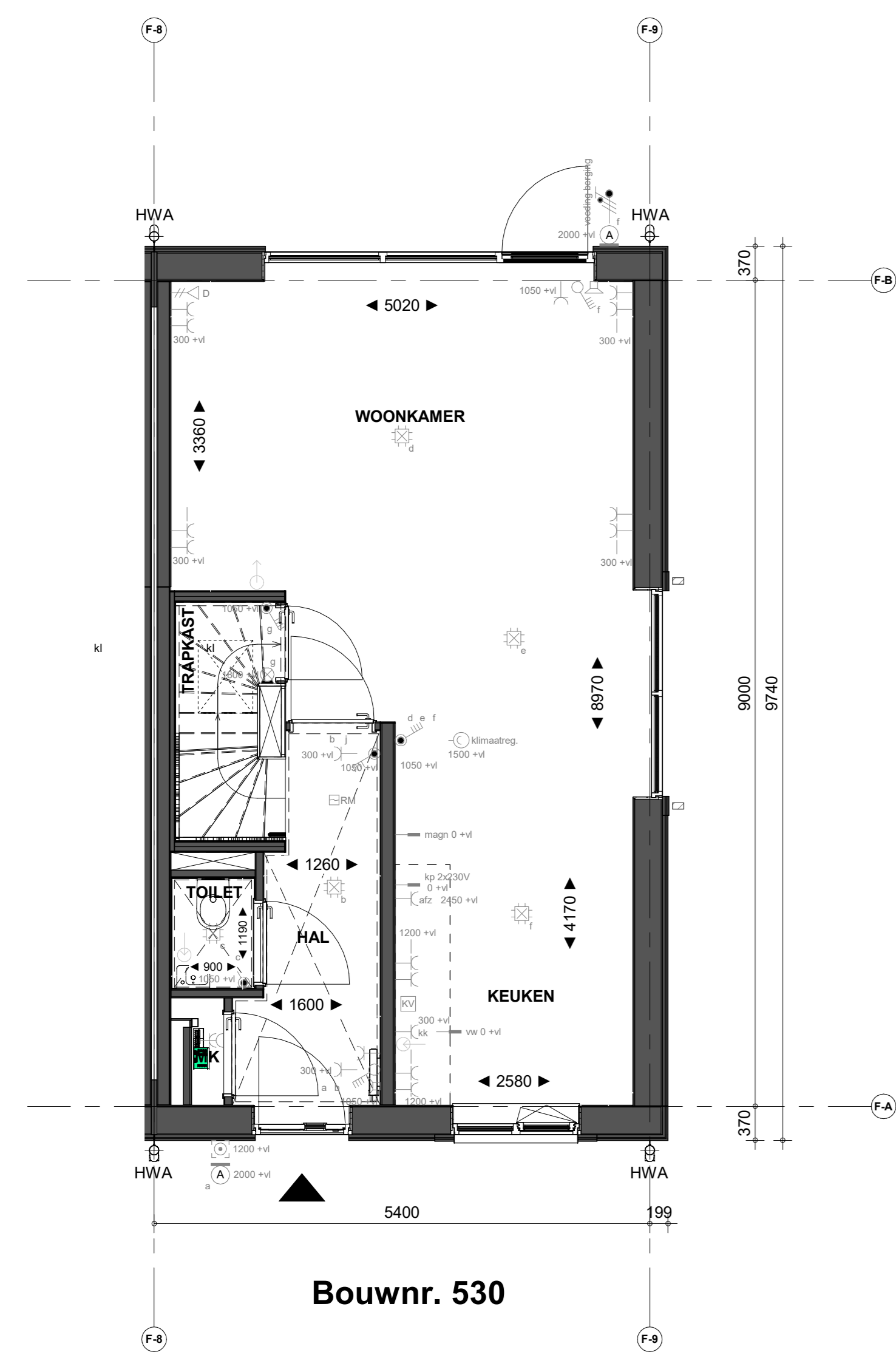
Begane grond
