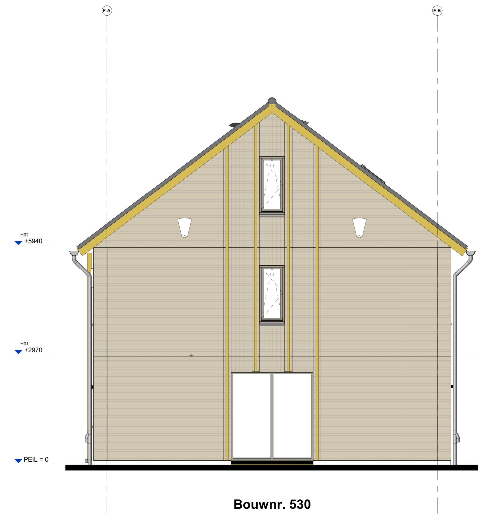
Rechter zijgevel
