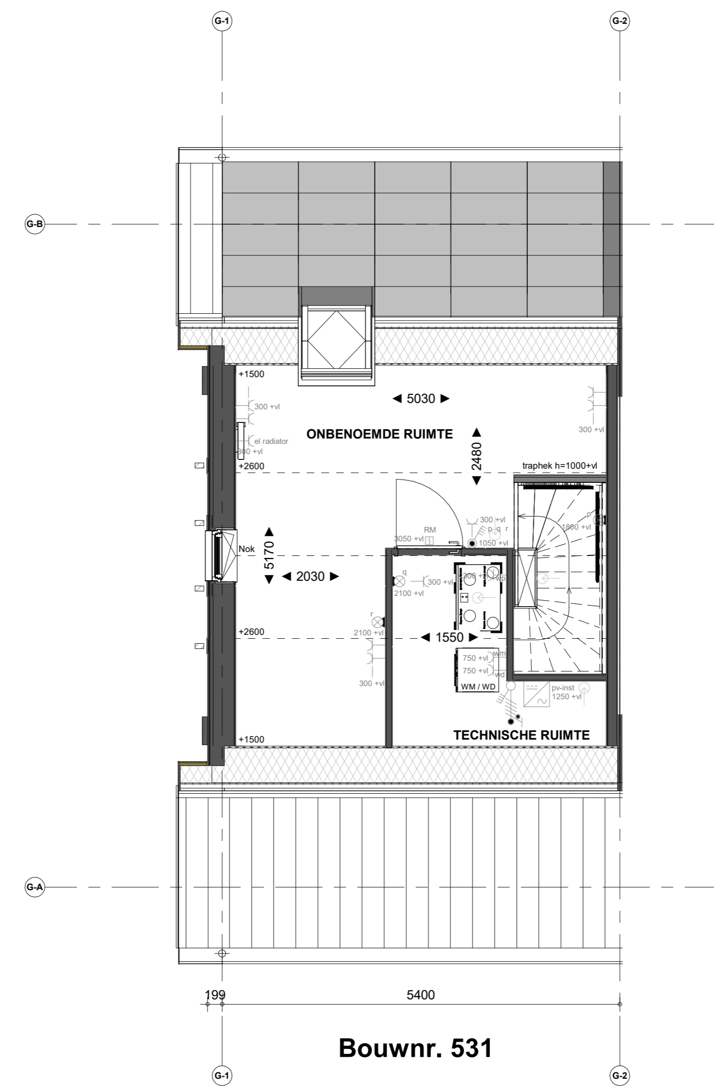
2e verdieping
