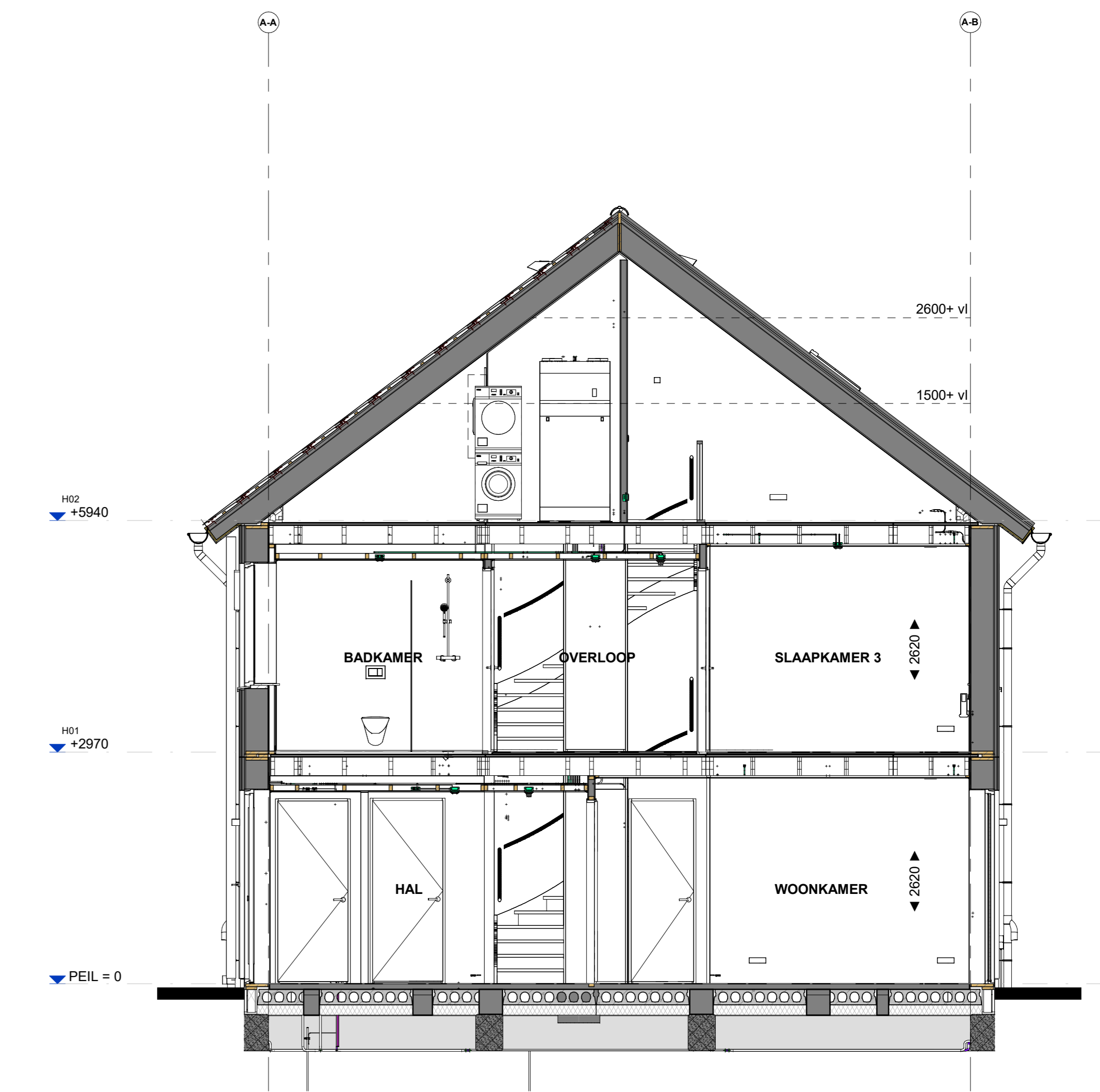
Doorsnede B531
