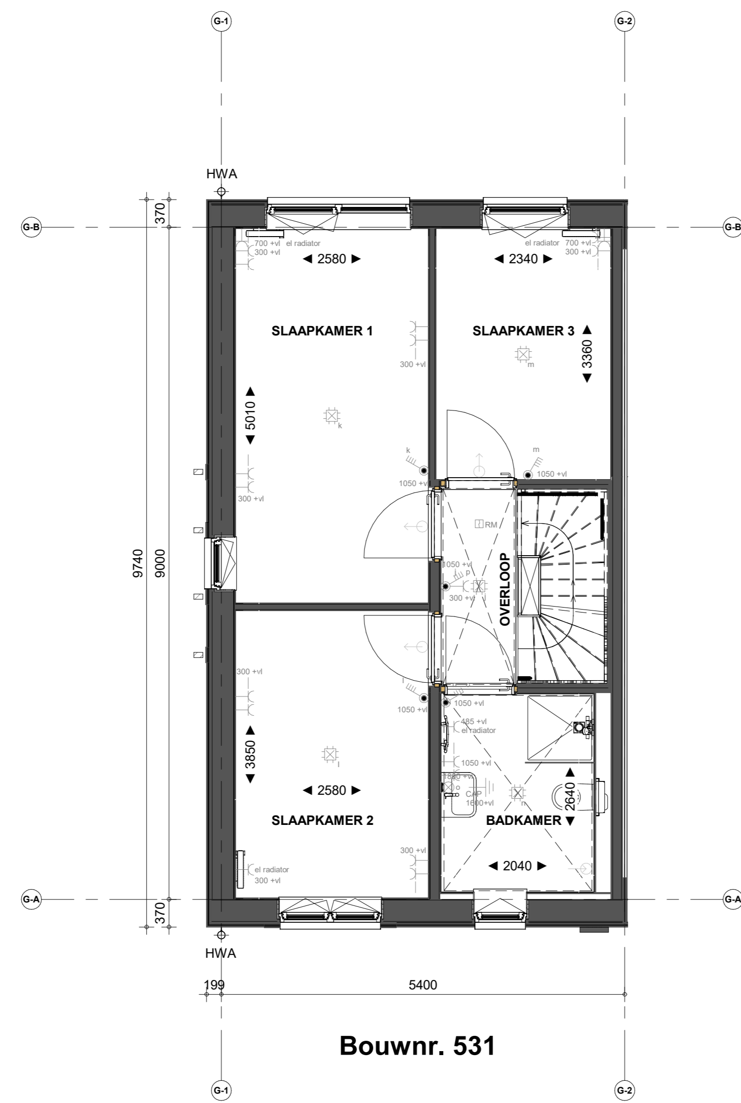
1e verdieping
