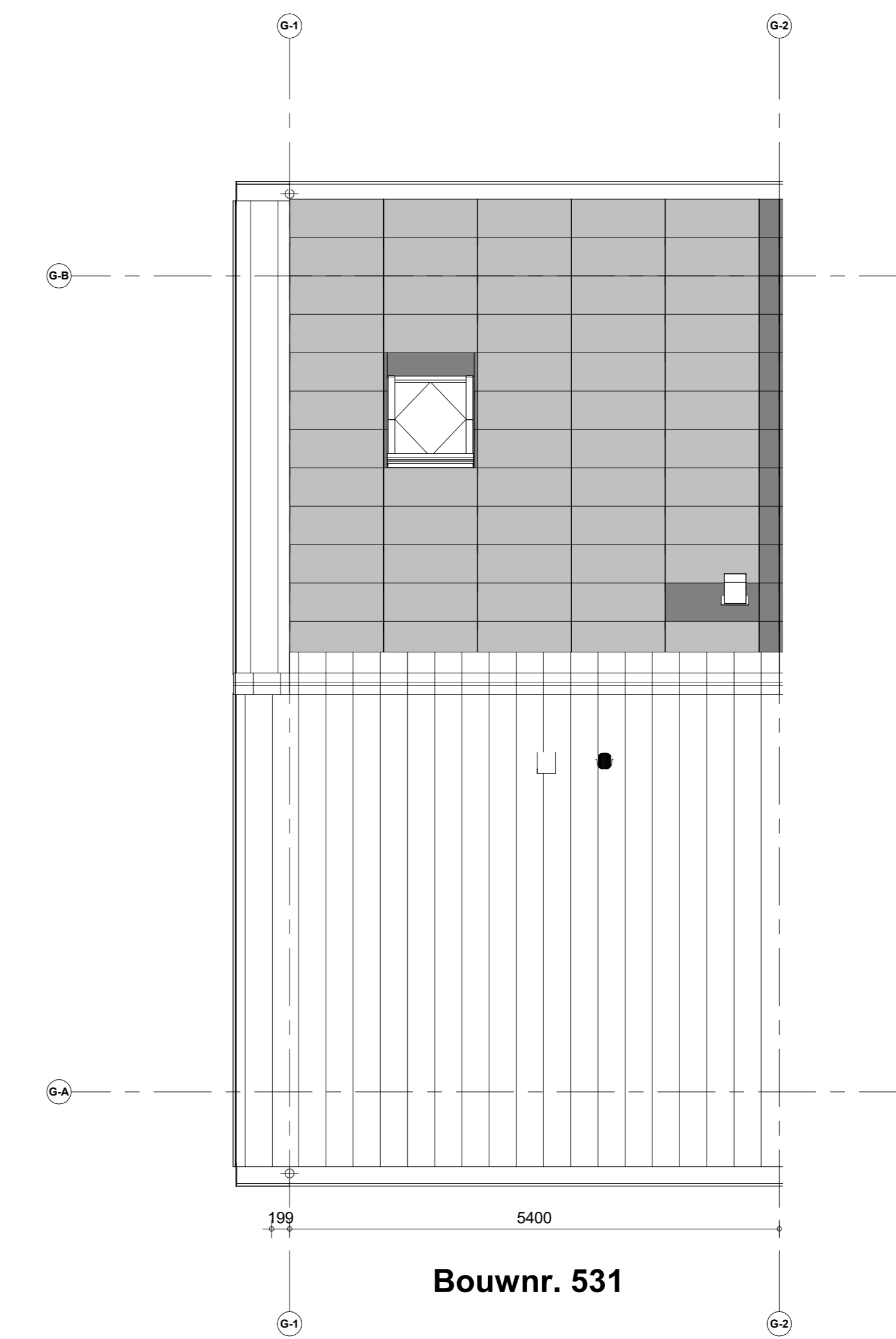
Dakaanzicht
