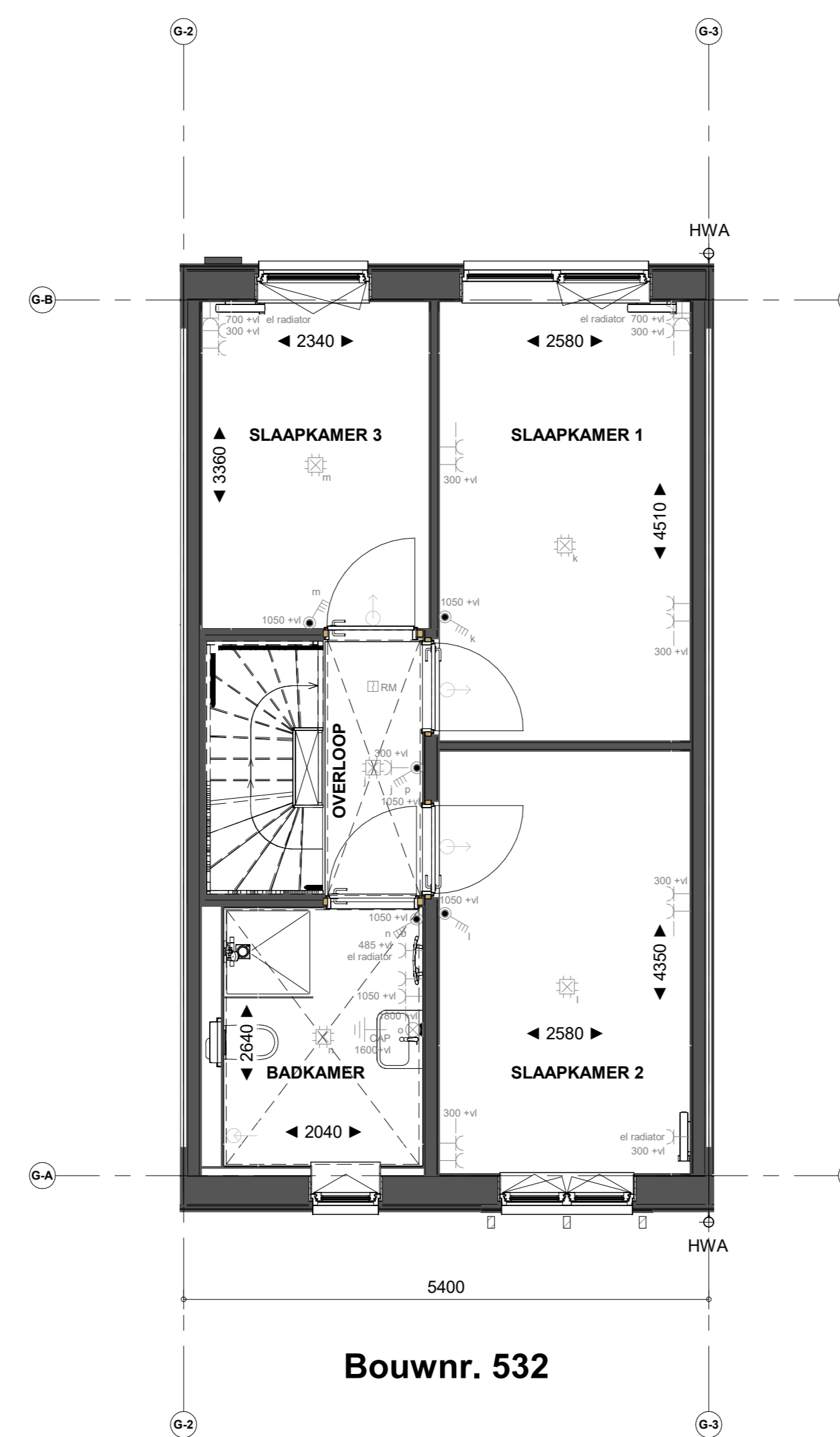
1e verdieping
