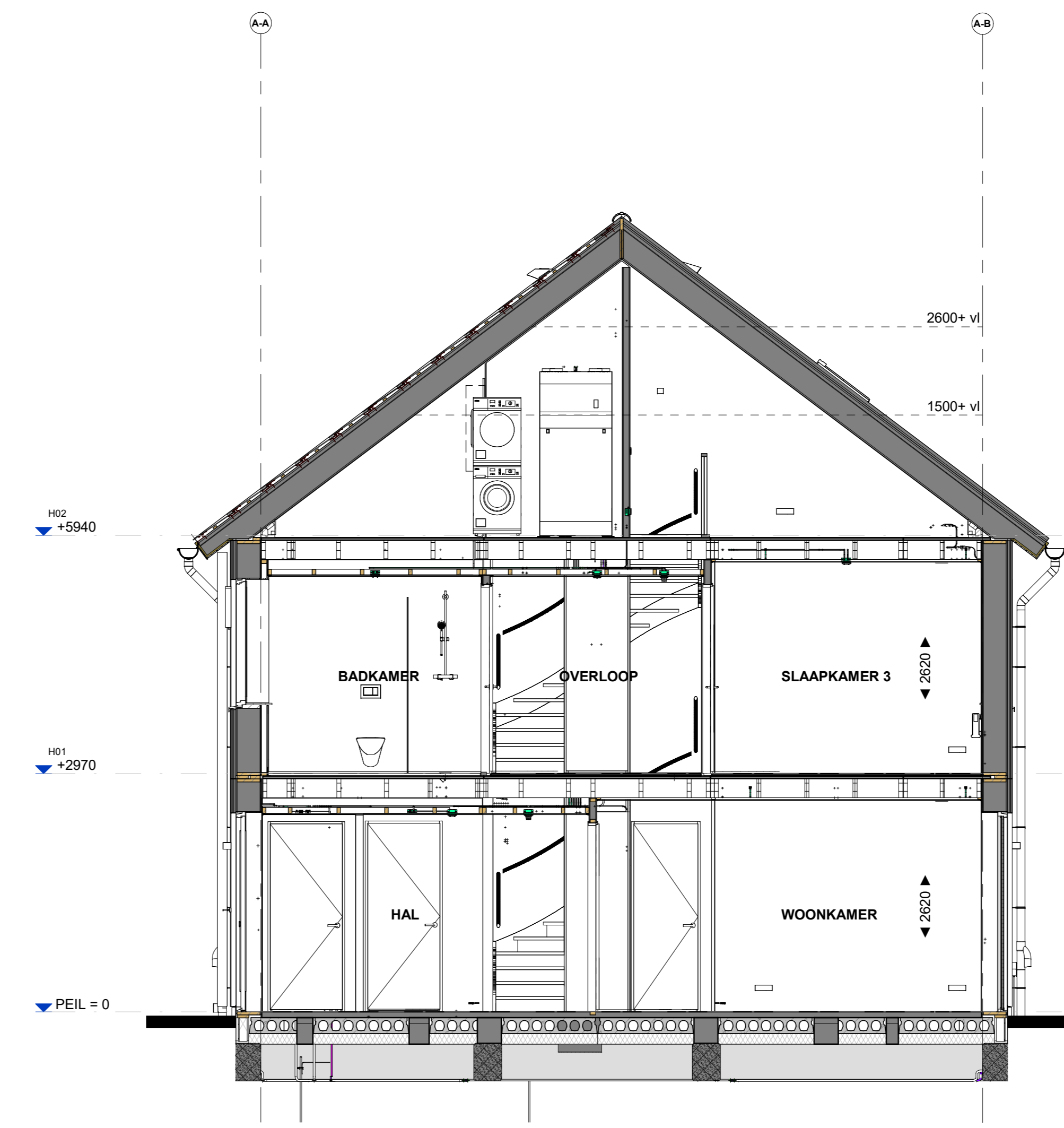
Doorsnede B532
