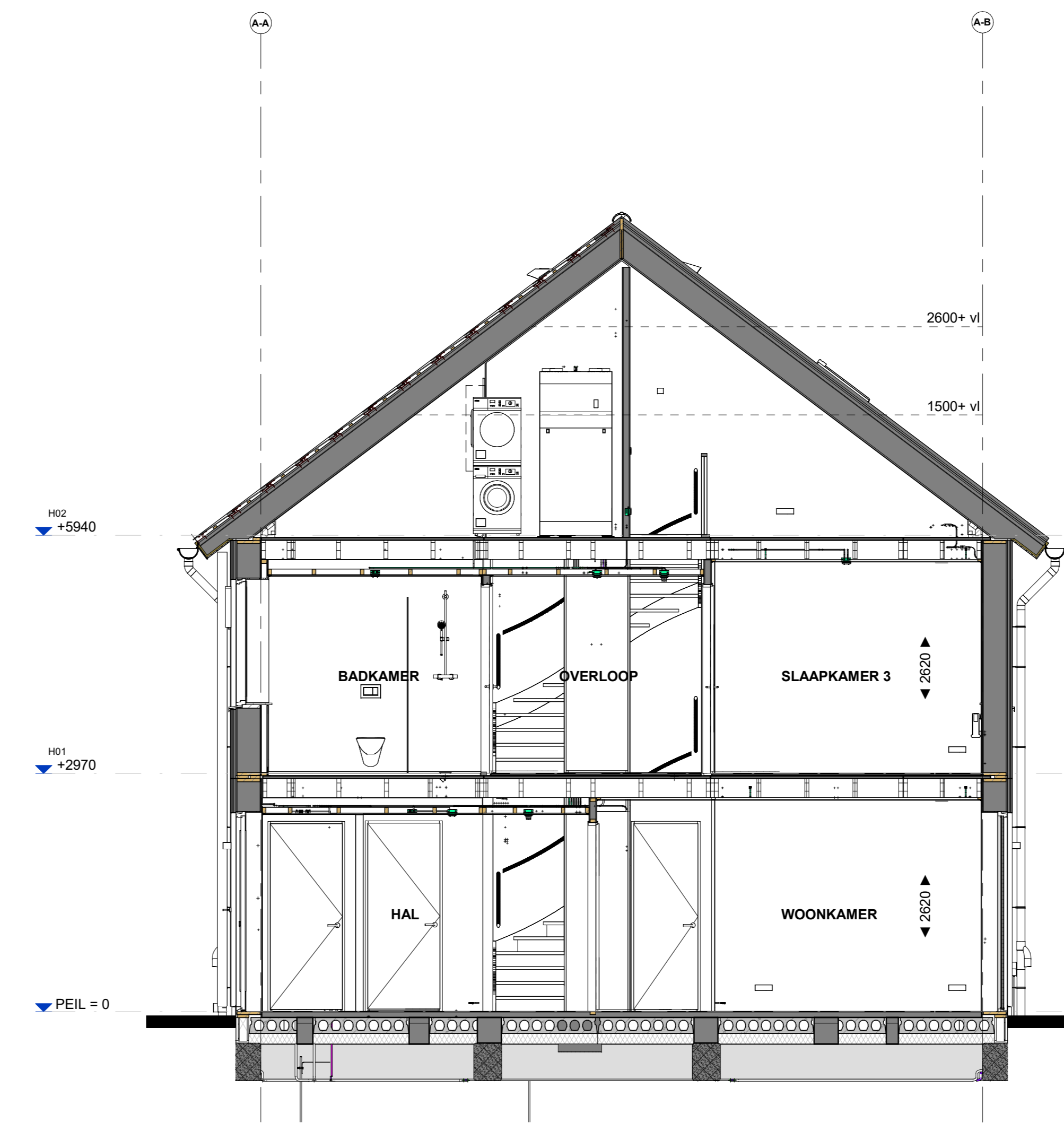
Doorsnede B533
