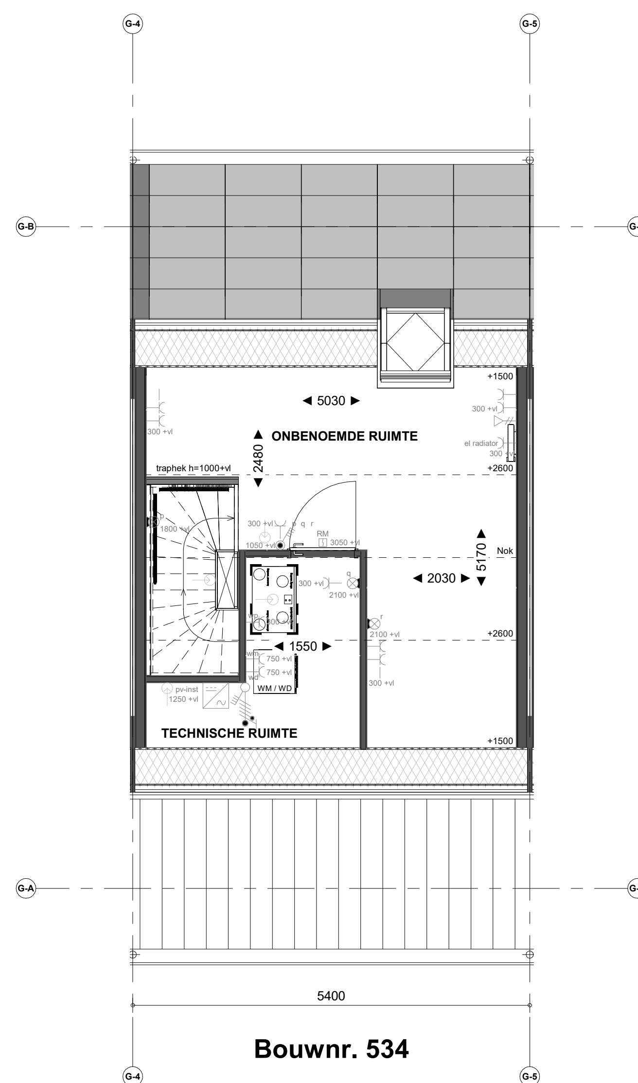
2e verdieping
