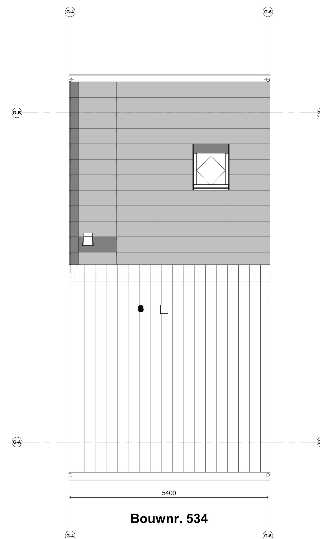
Dakaanzicht
