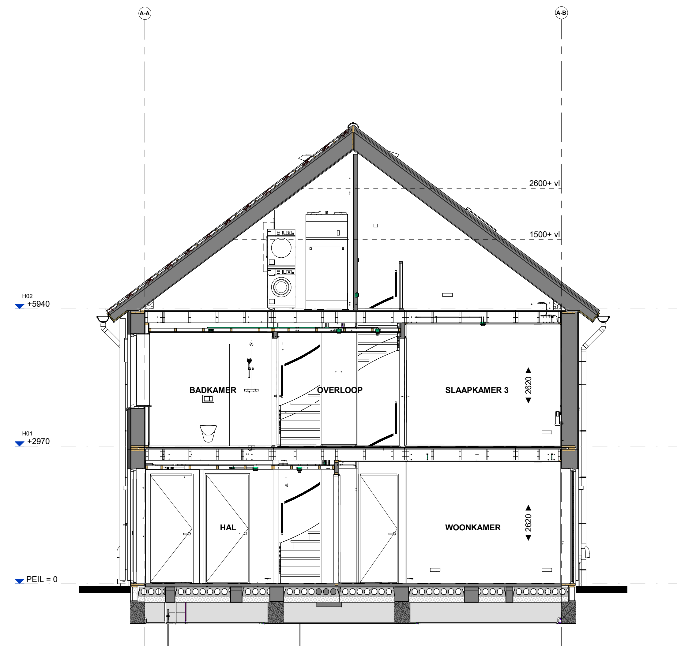
Doorsnede B534
