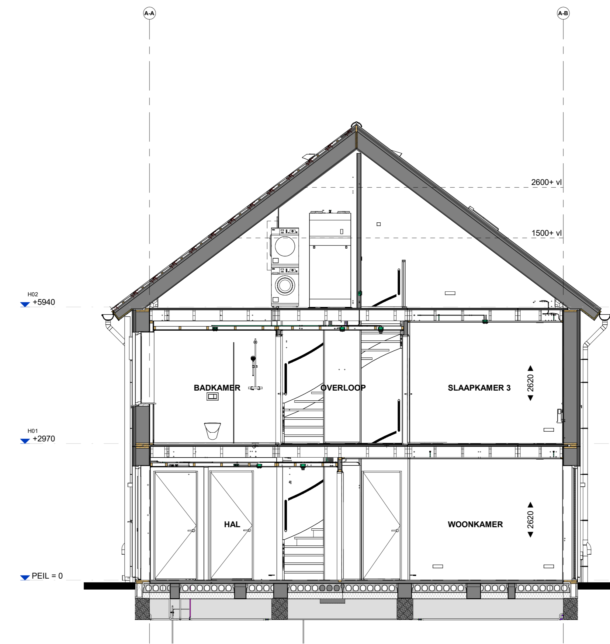
Doorsnede B535
