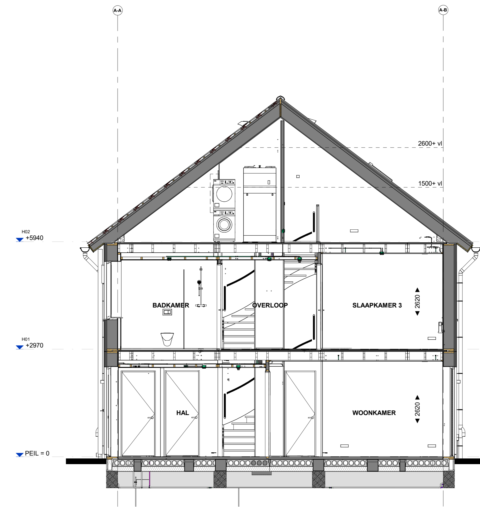
Doorsnede B536
