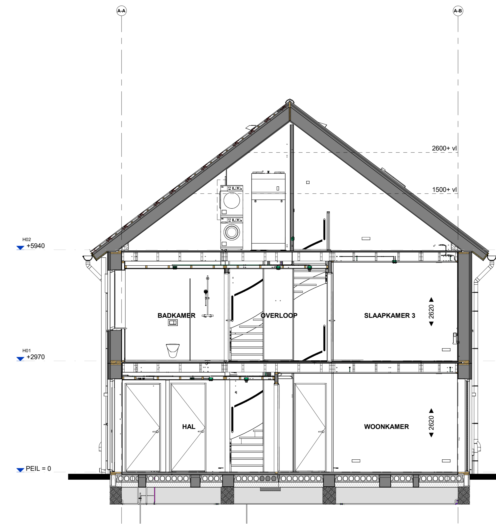
Doorsnede B537
