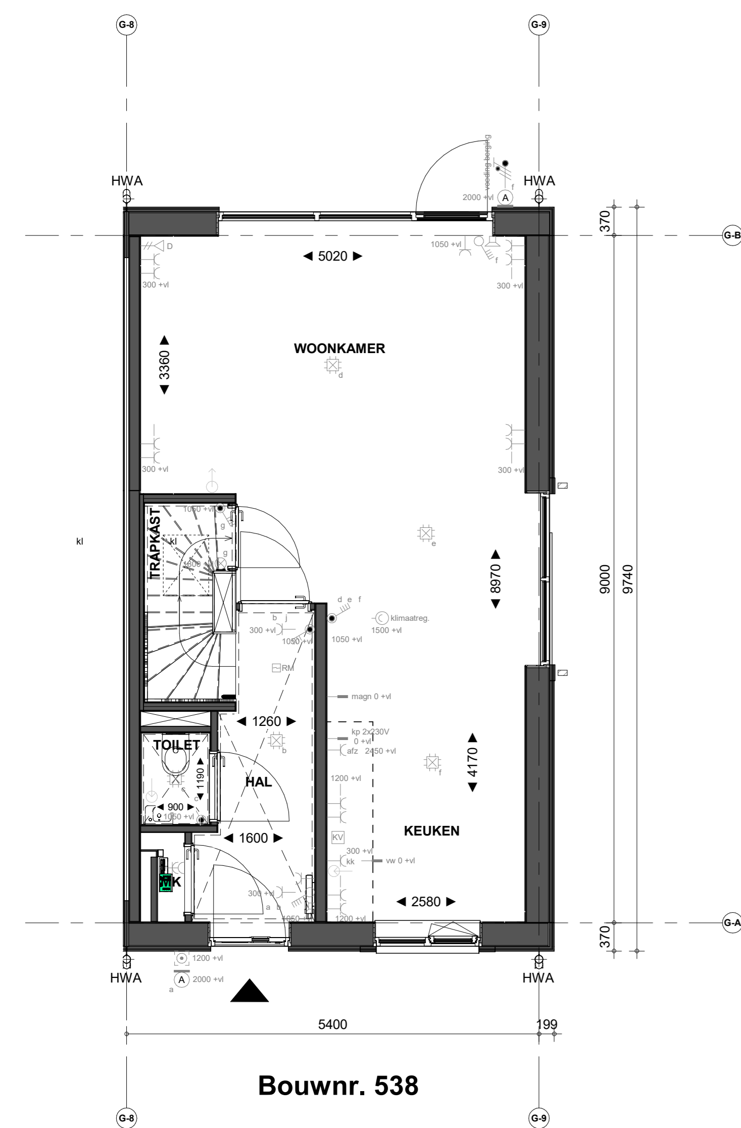
Begane grond
