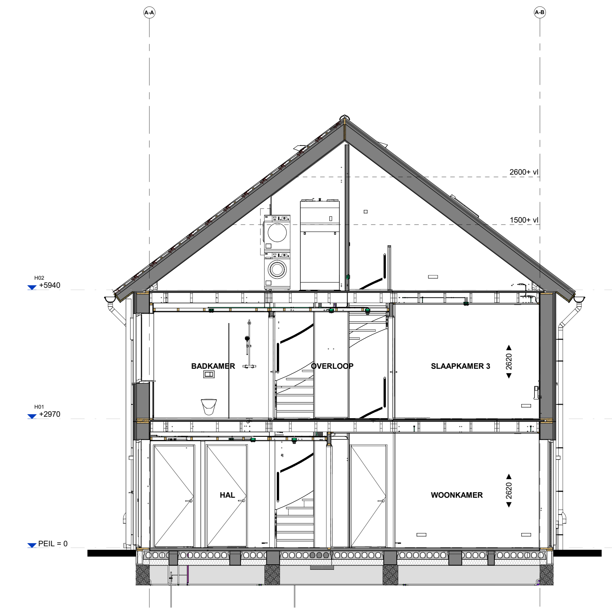
Doorsnede B538
