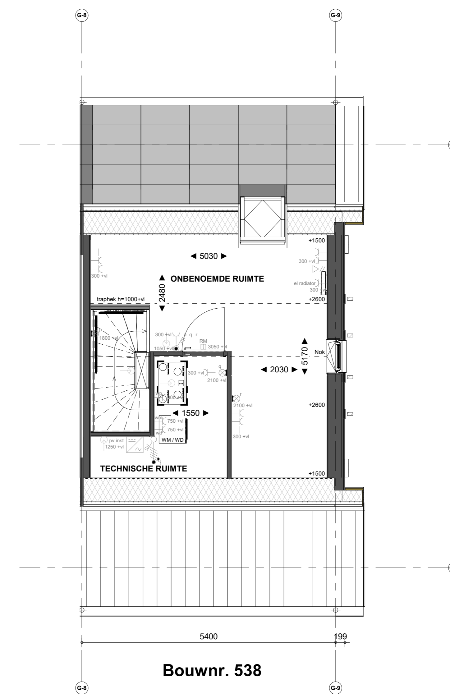
2e verdieping
