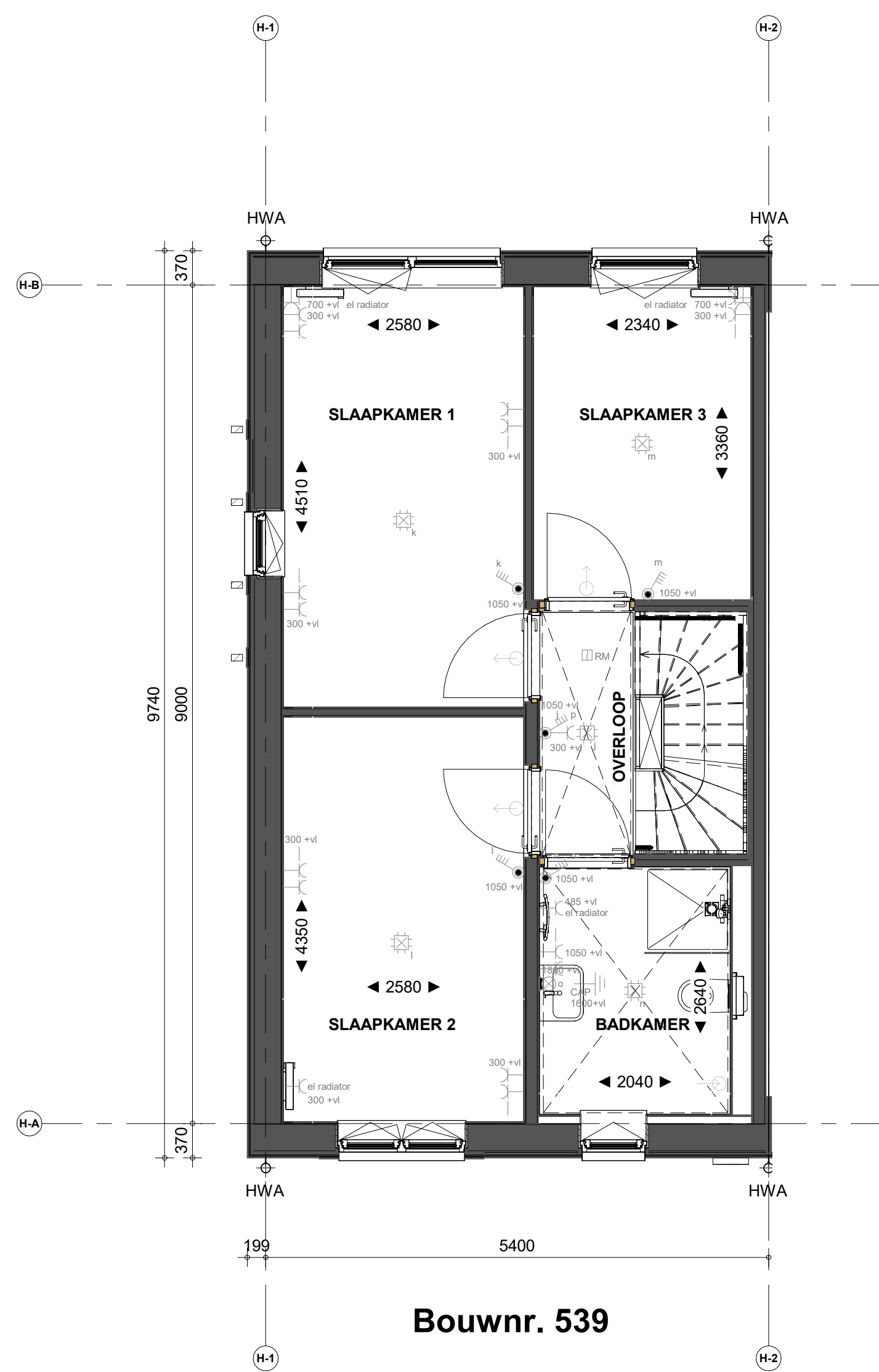
1e verdieping
