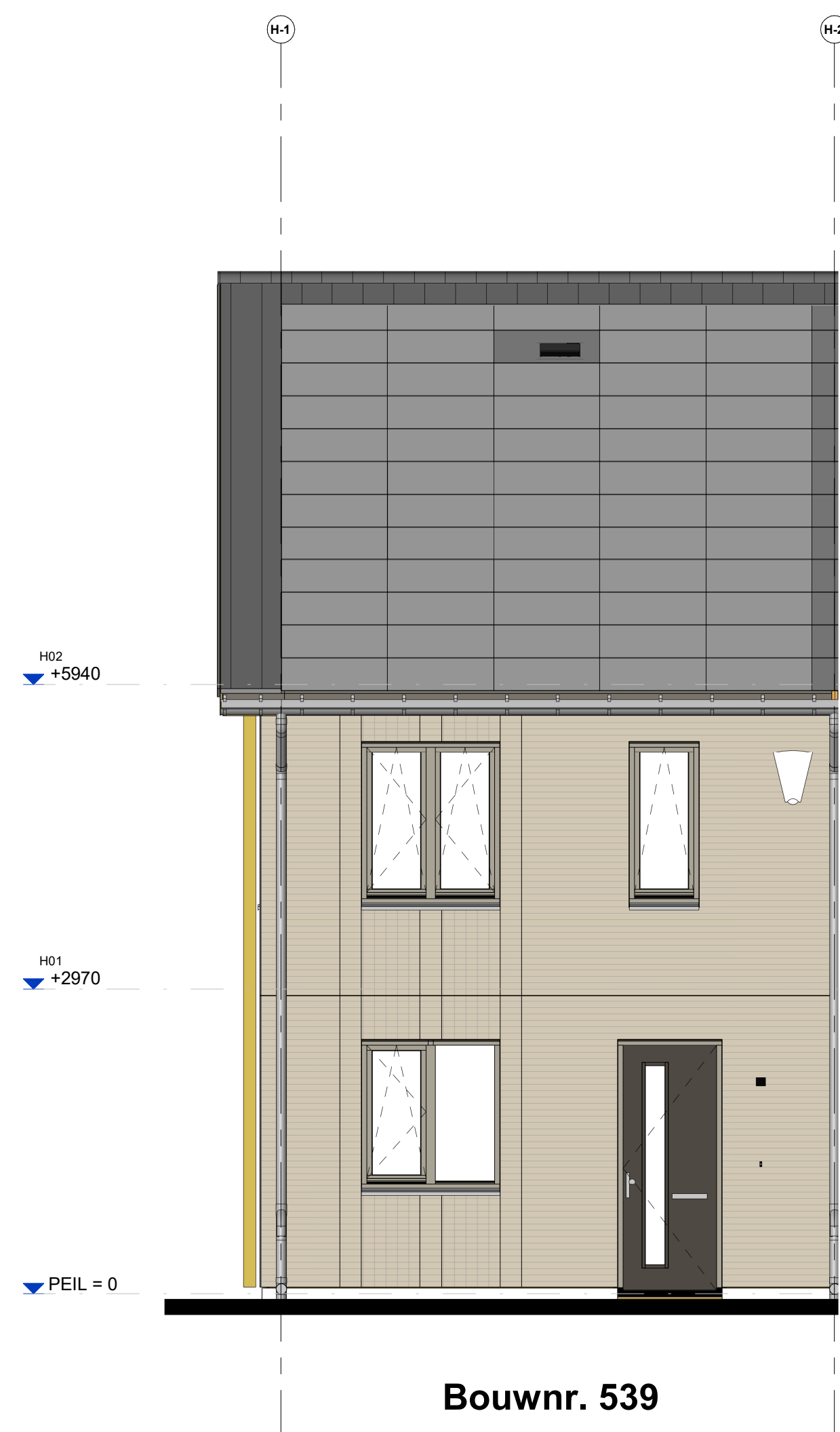
Voorgevel
