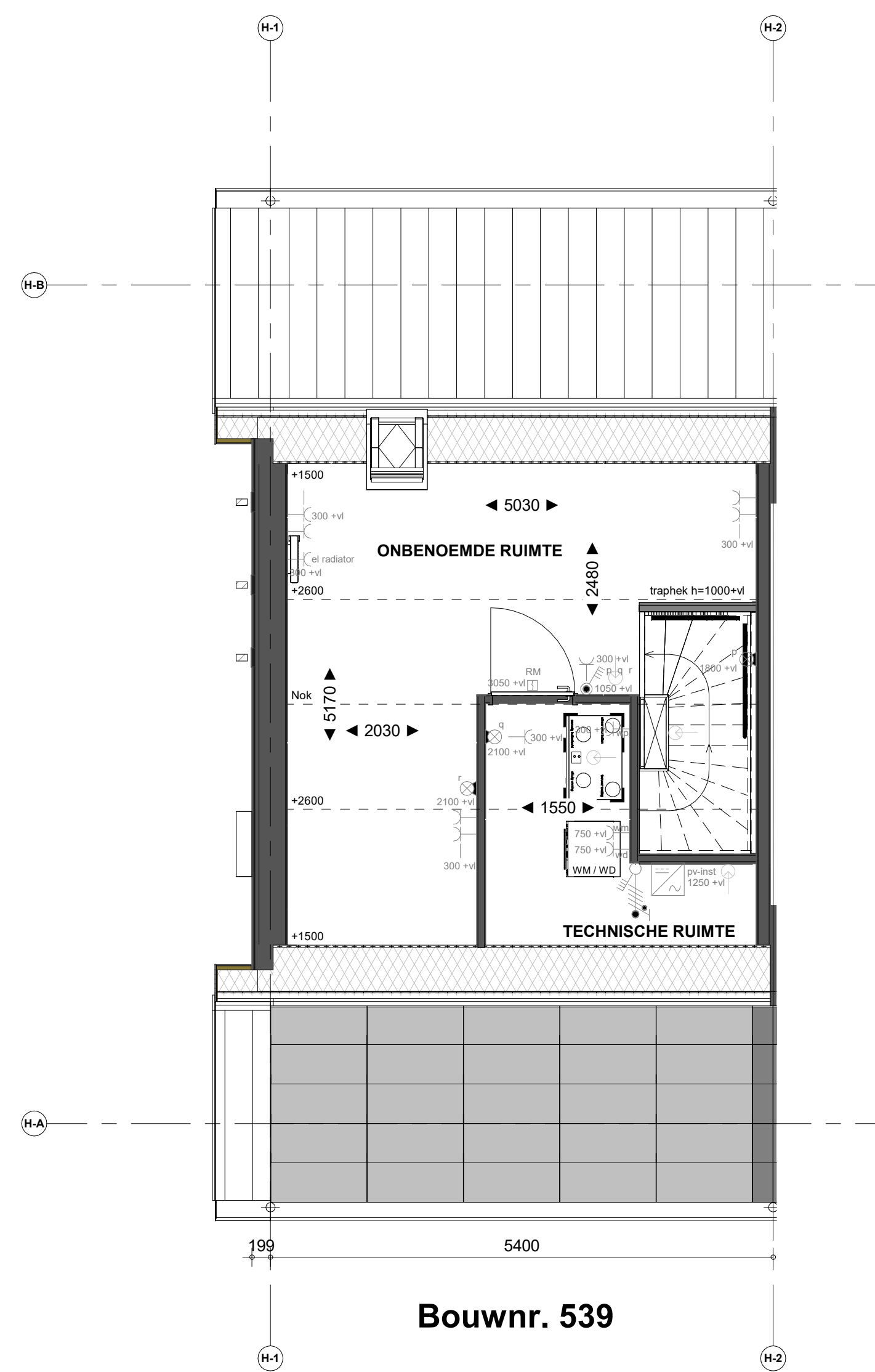
2e verdieping
