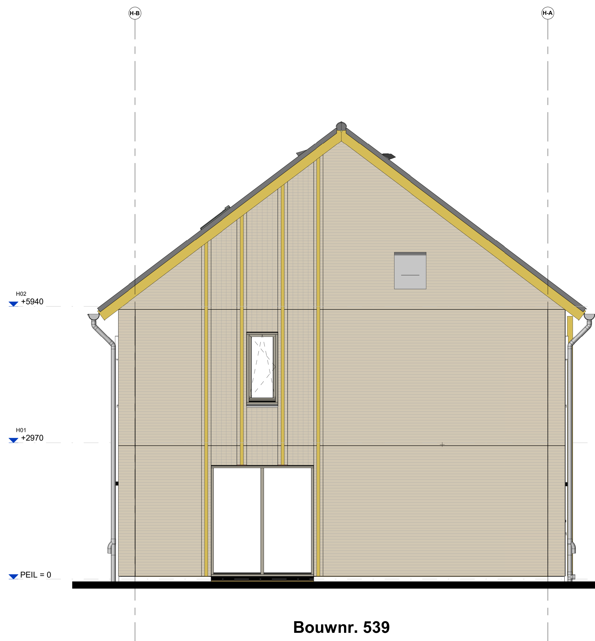
Linker zijgevel
