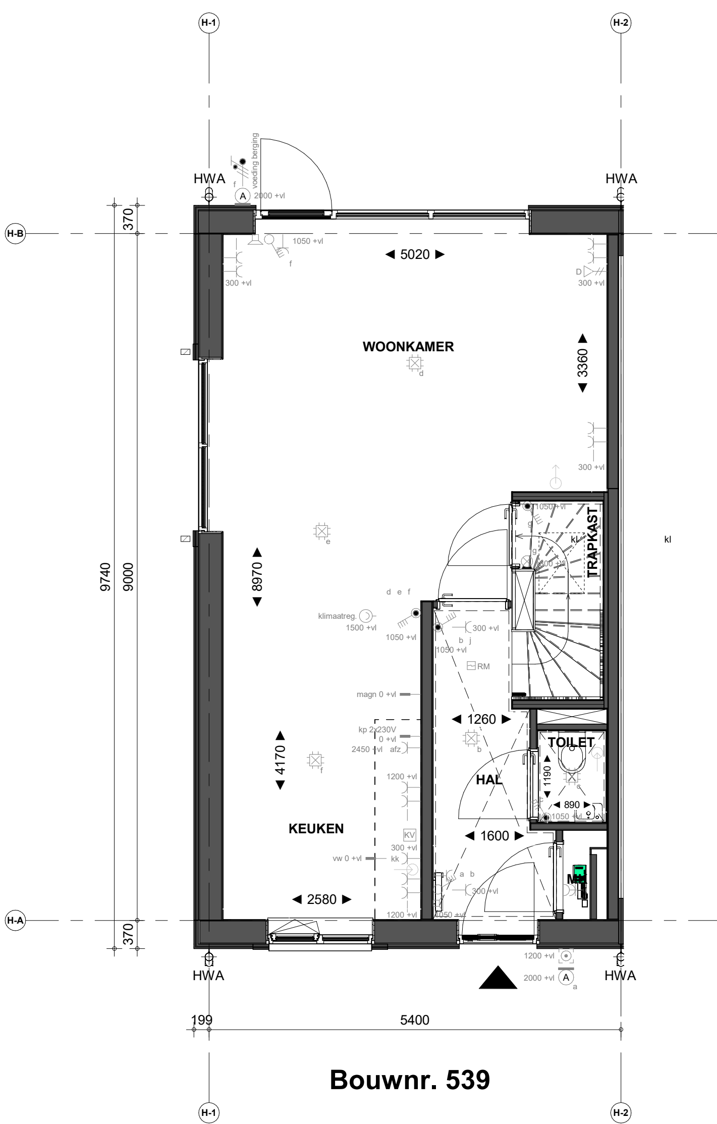
Begane grond
