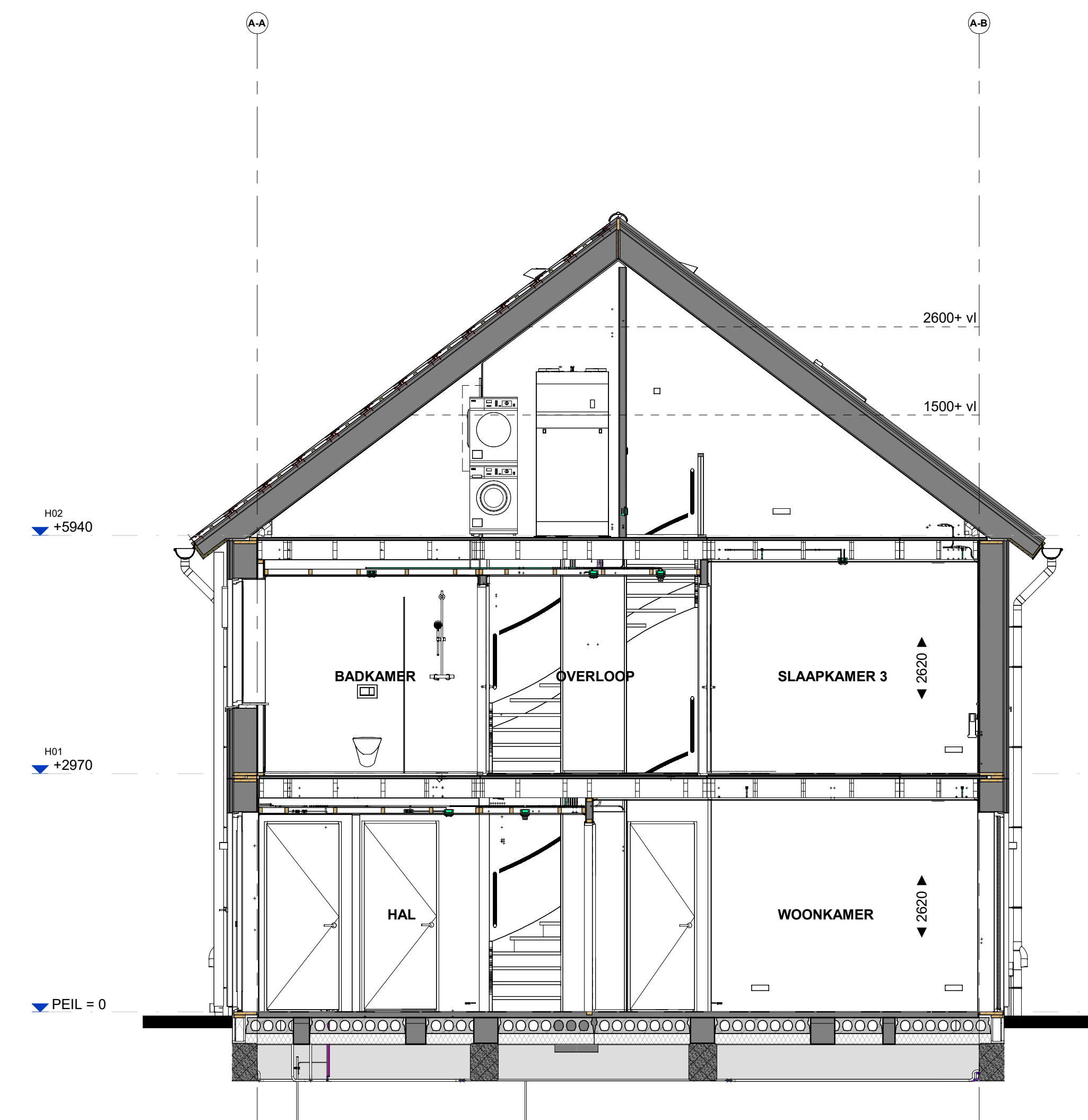
Doorsnede B539
