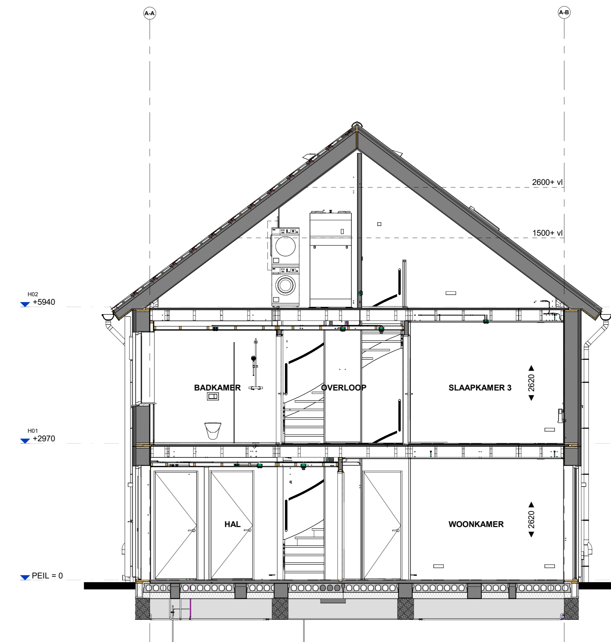
Doorsnede B540
