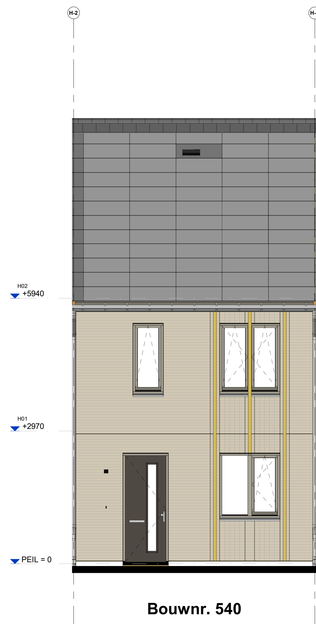
Voorgevel
