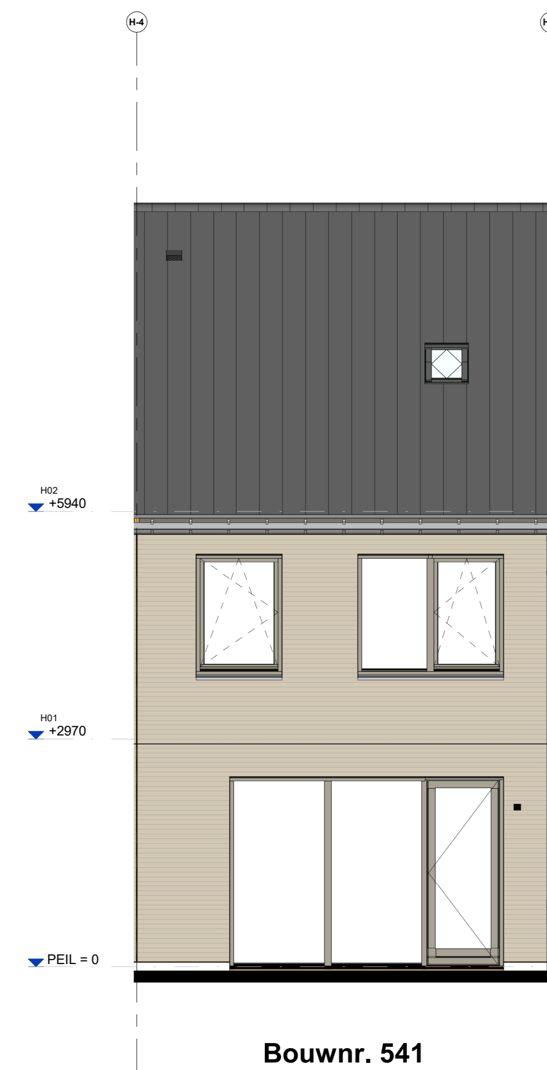
Achtergevel
