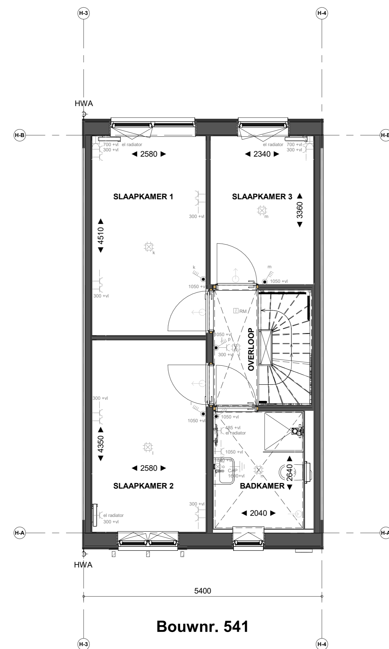
1e verdieping
