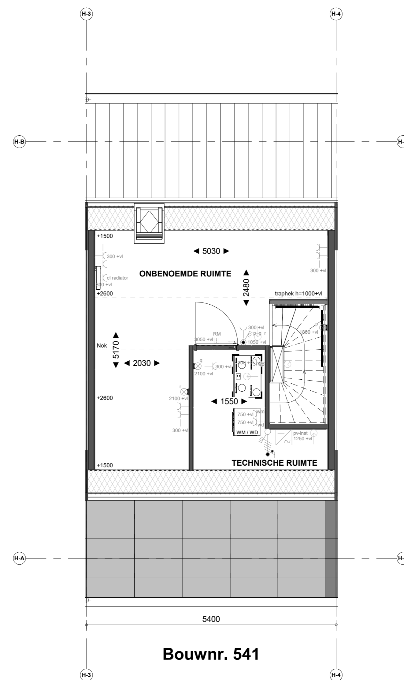
2e verdieping
