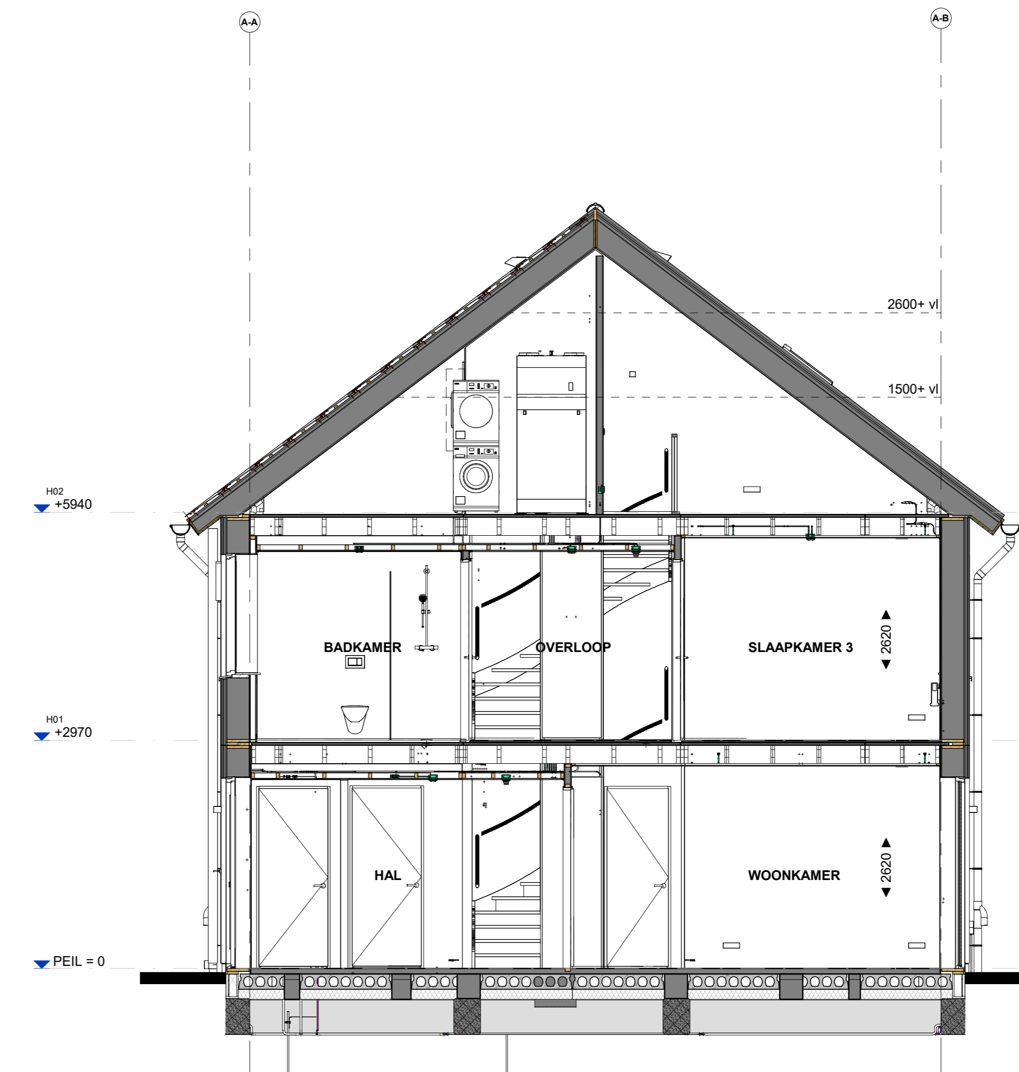
Doorsnede B541
