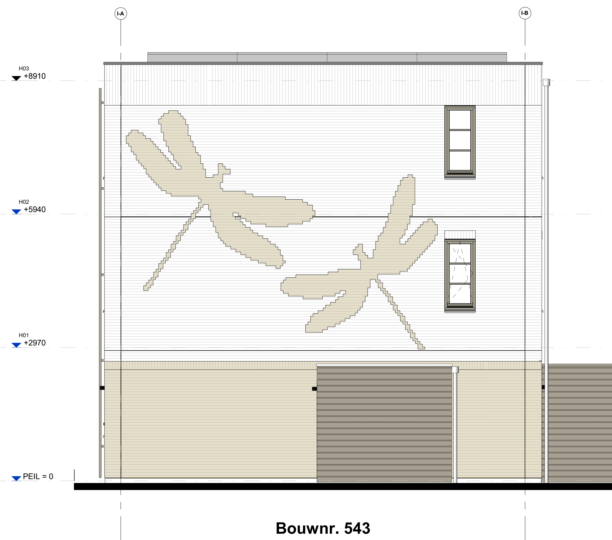
Rechter zijgevel
