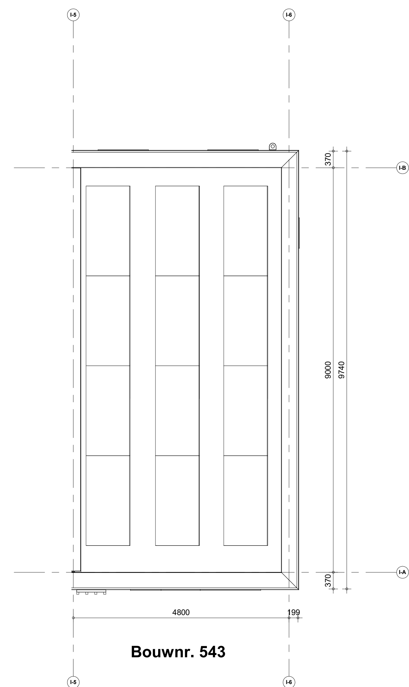
Dakaanzicht
