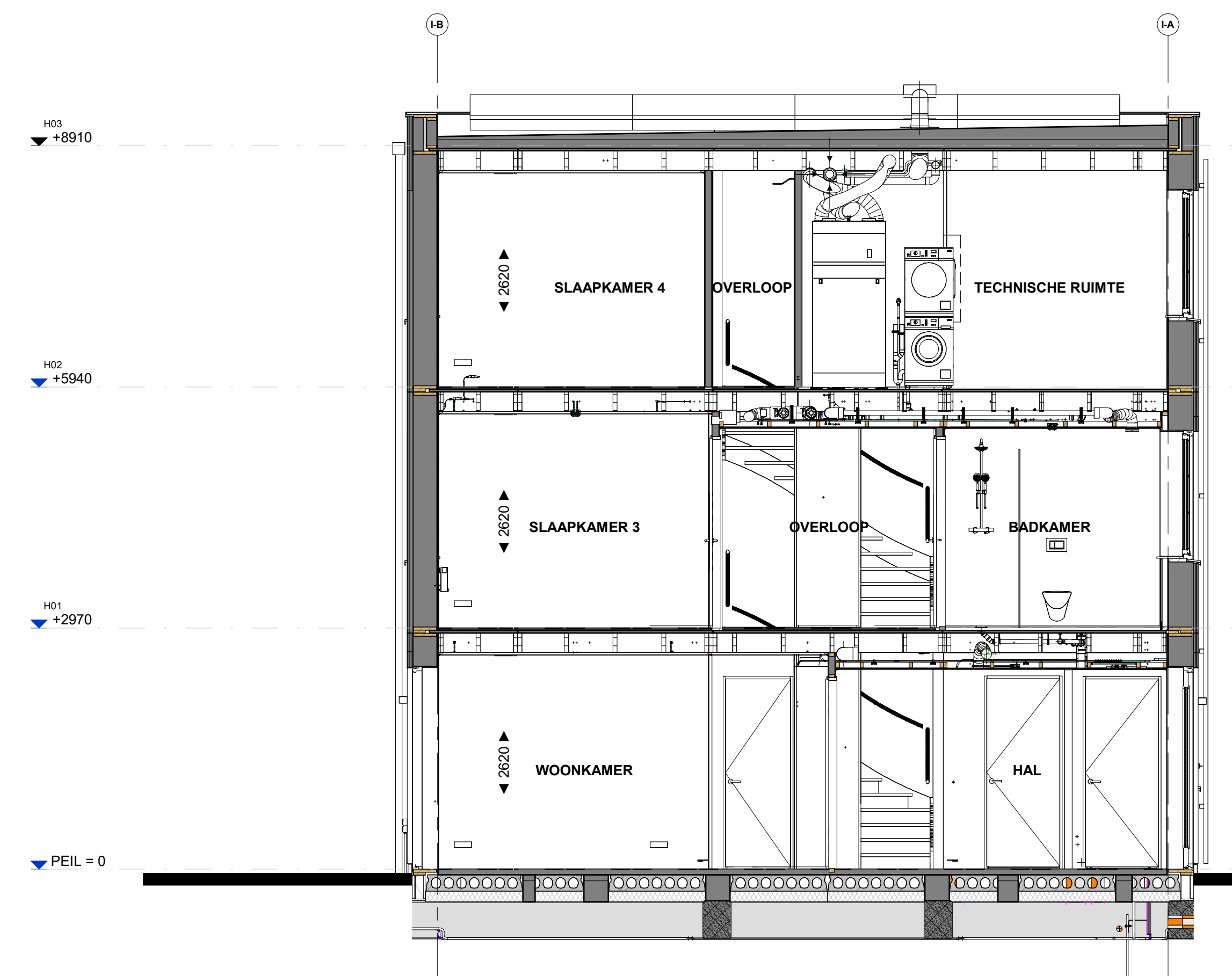
Doorsnede B543
