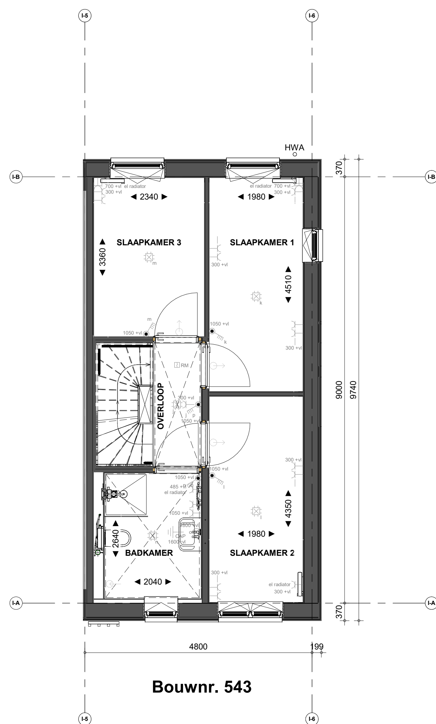
1e verdieping
