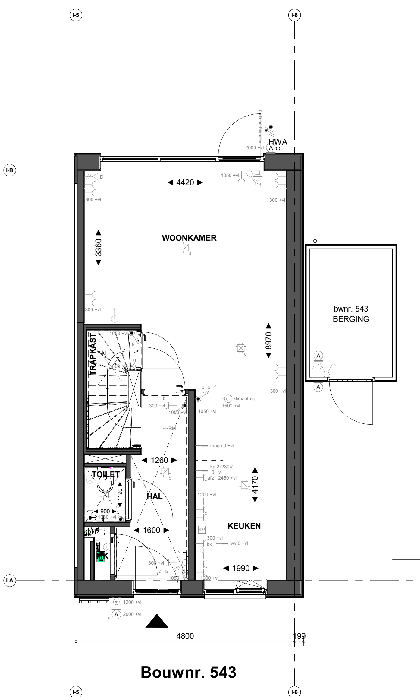
Begane grond
