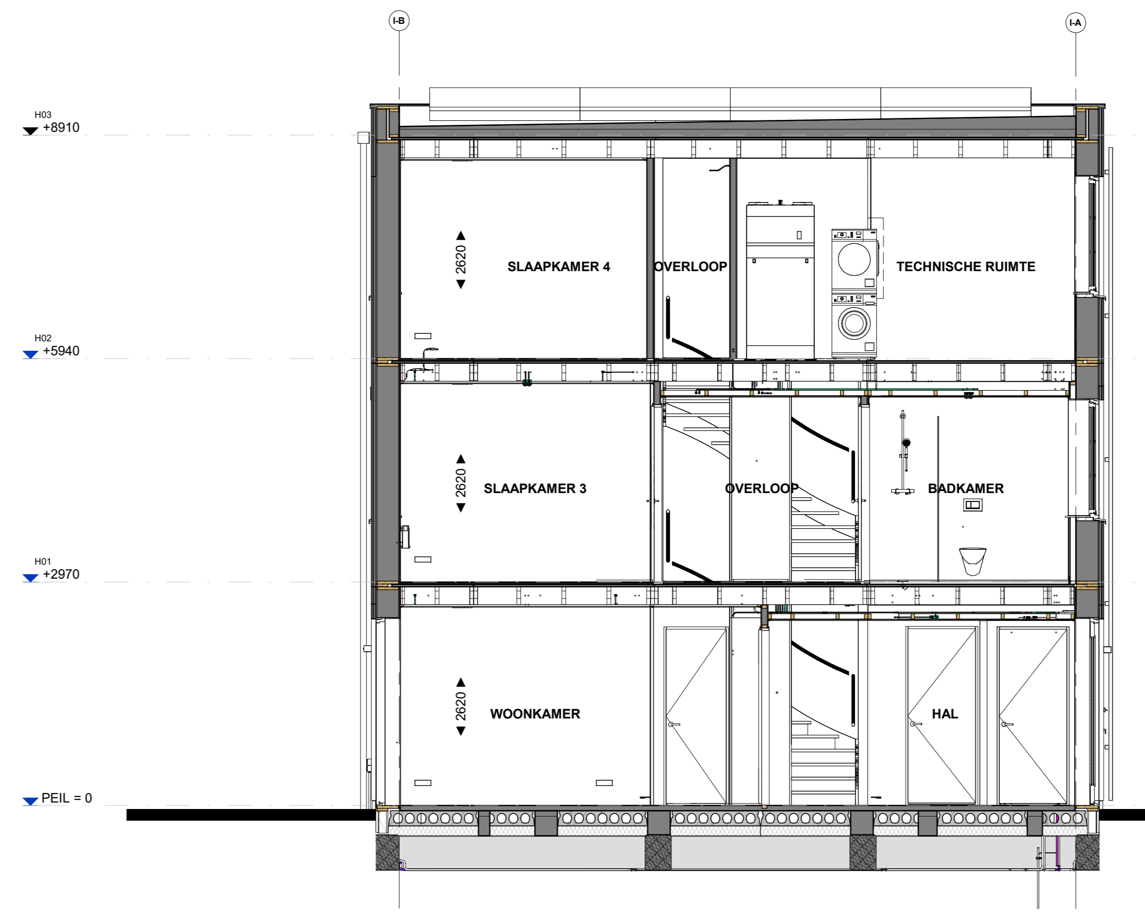
Doorsnede B544
