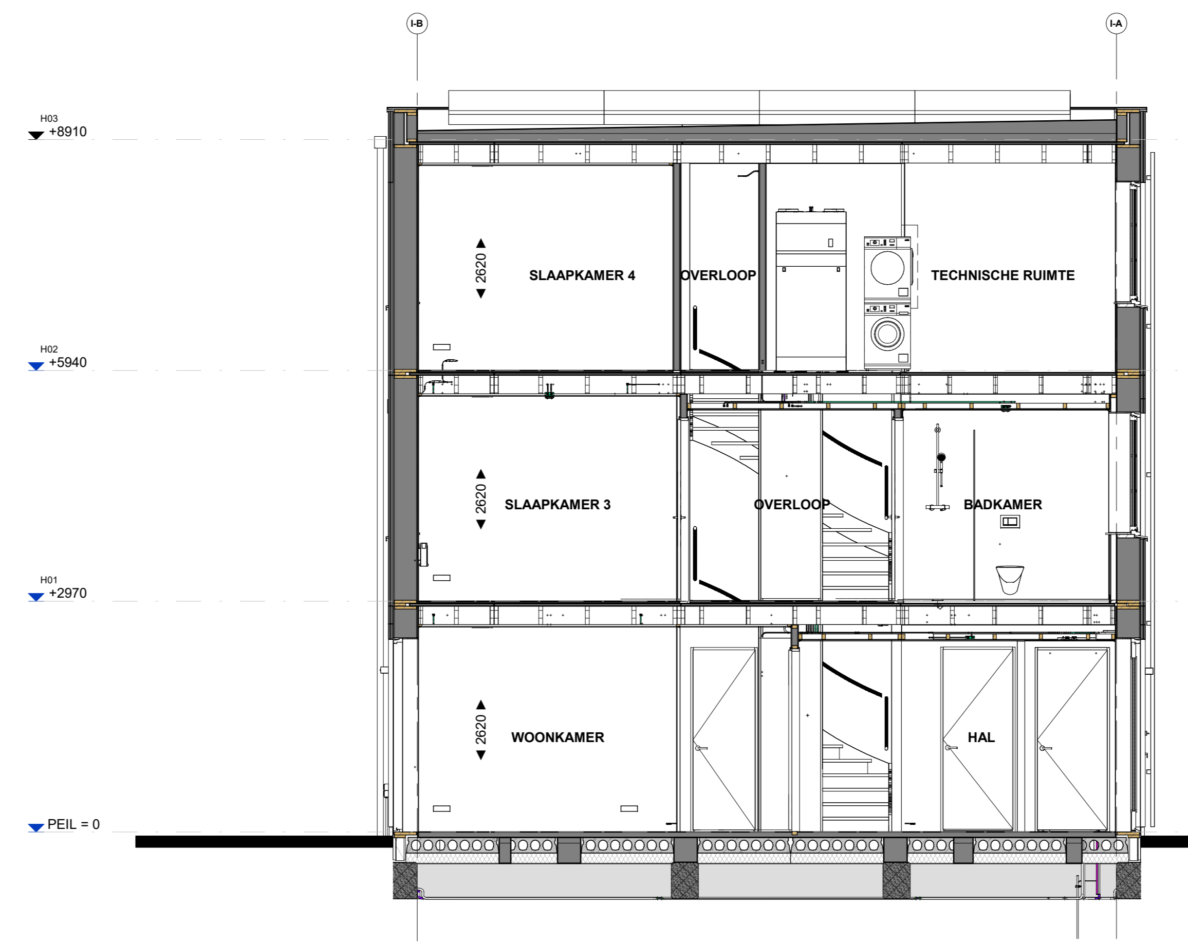
Doorsnede B545
