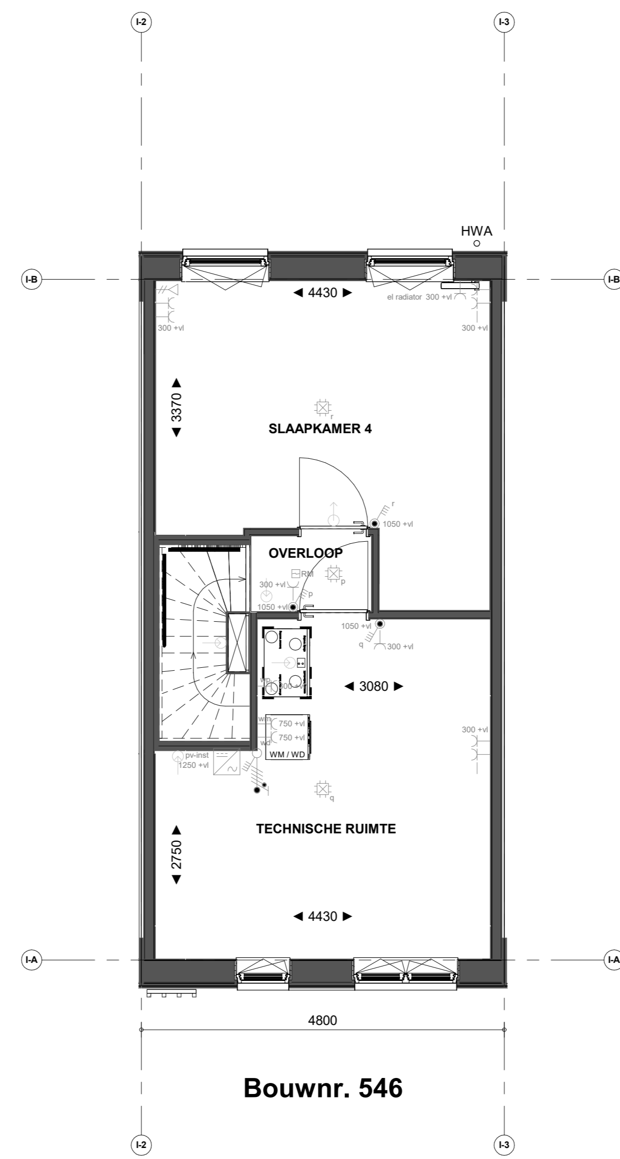
2e verdieping
