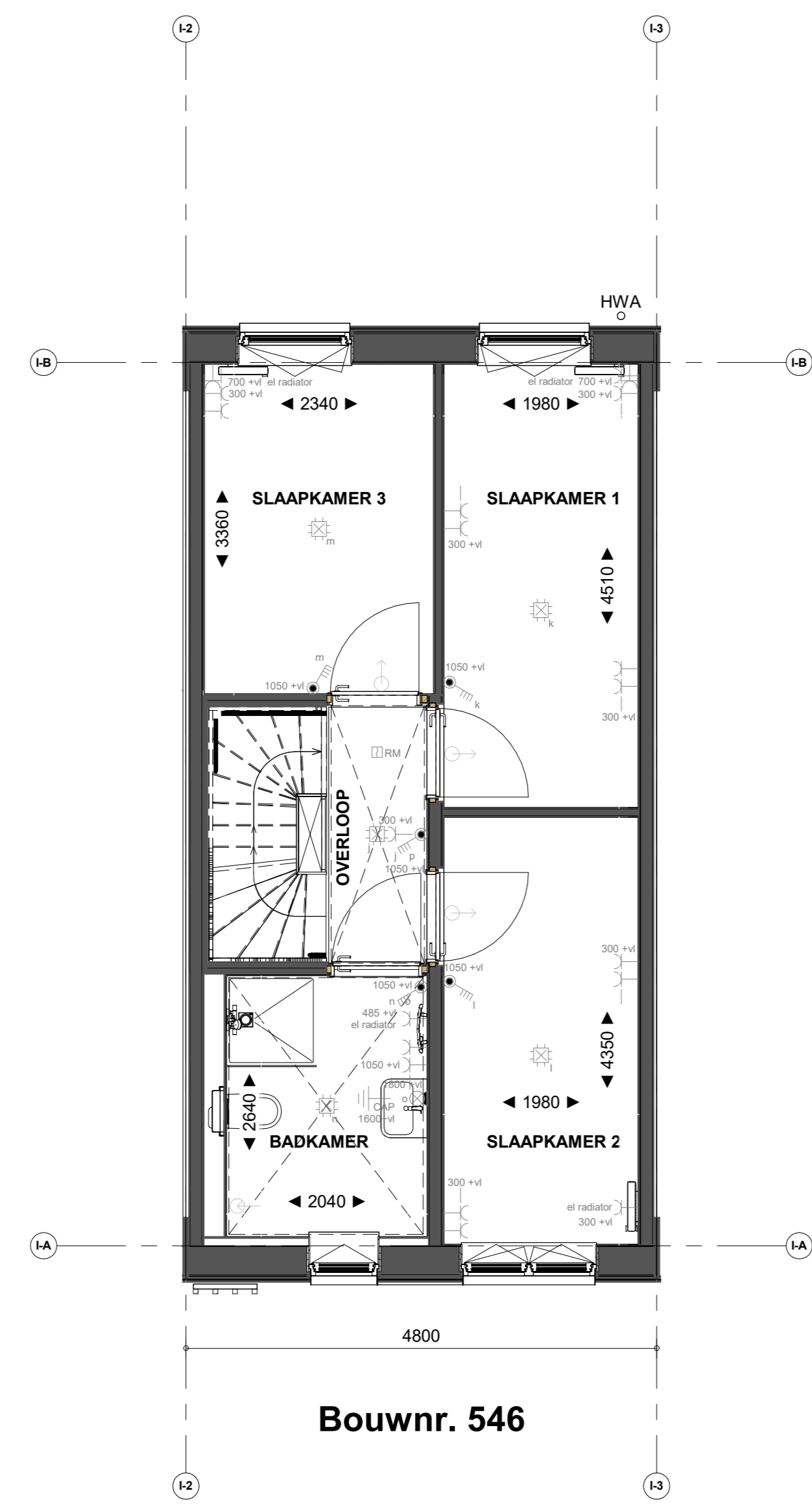
1e verdieping
