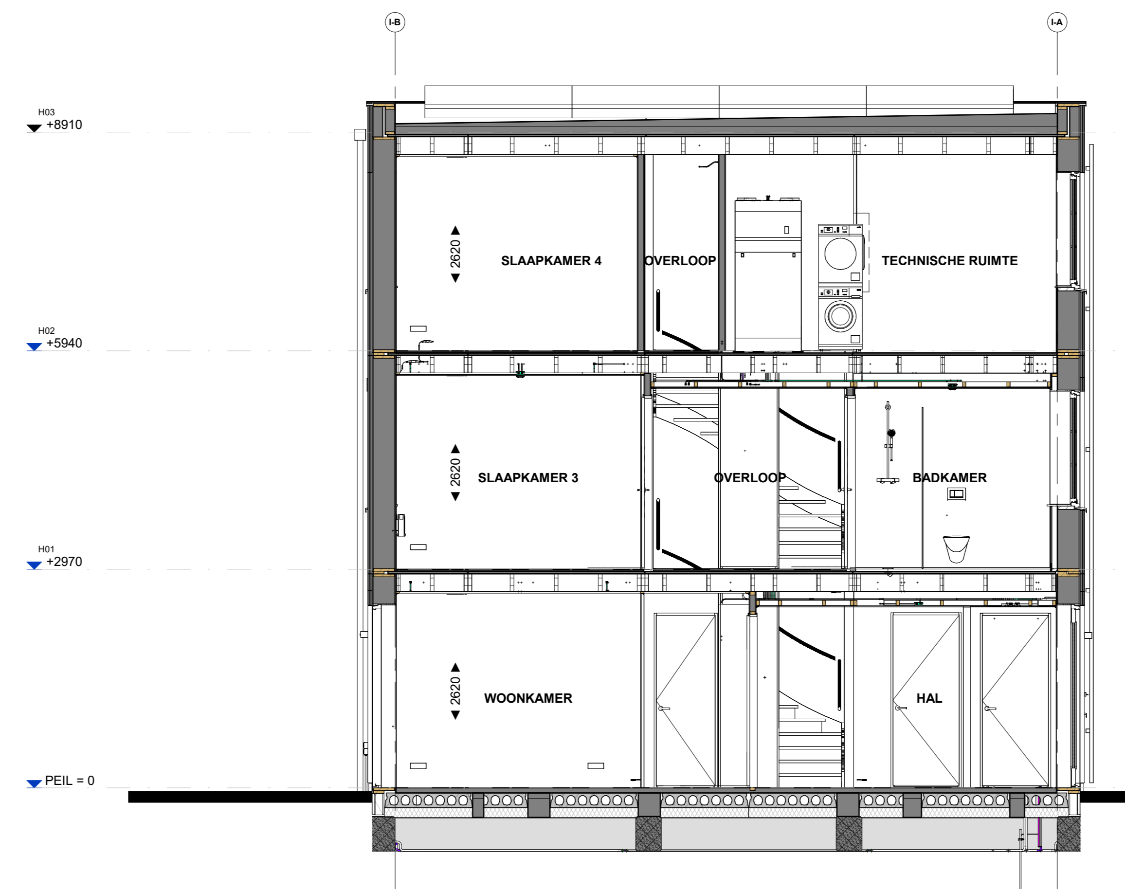
Doorsnede B546
