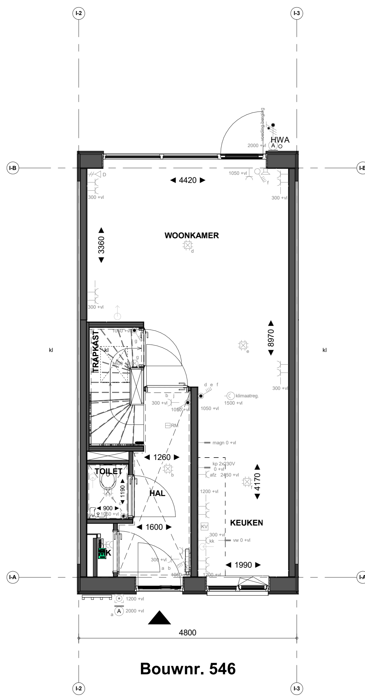
Begane grond
