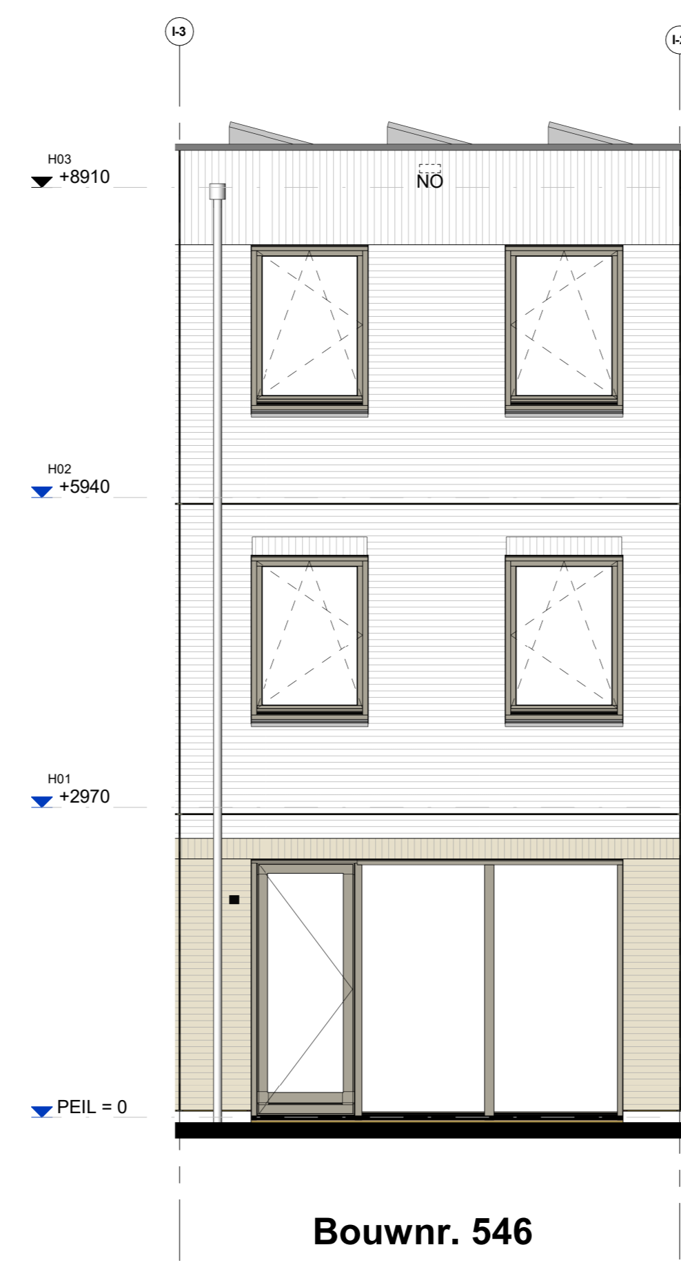
Achtergevel
