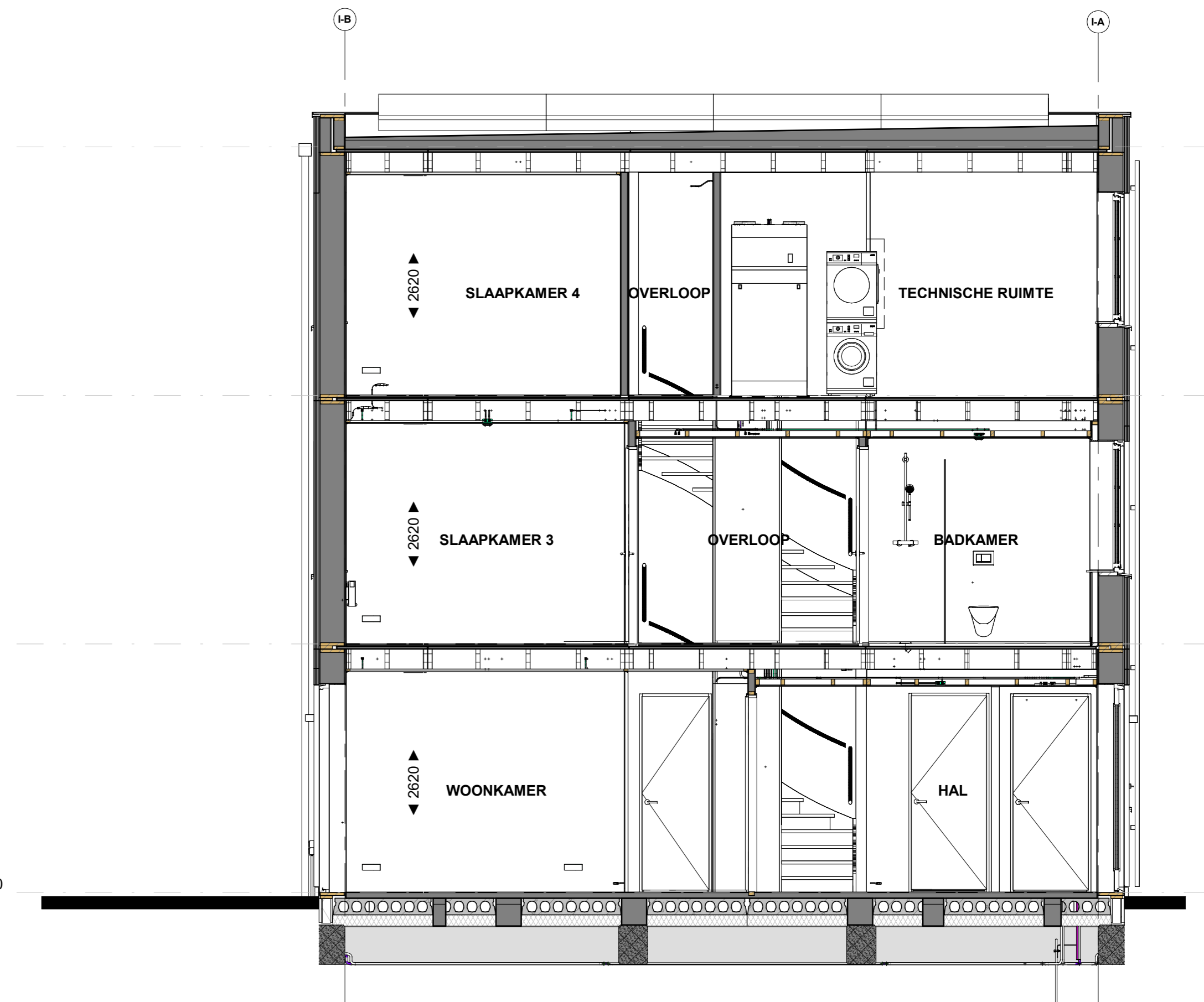
Doorsnede B547
