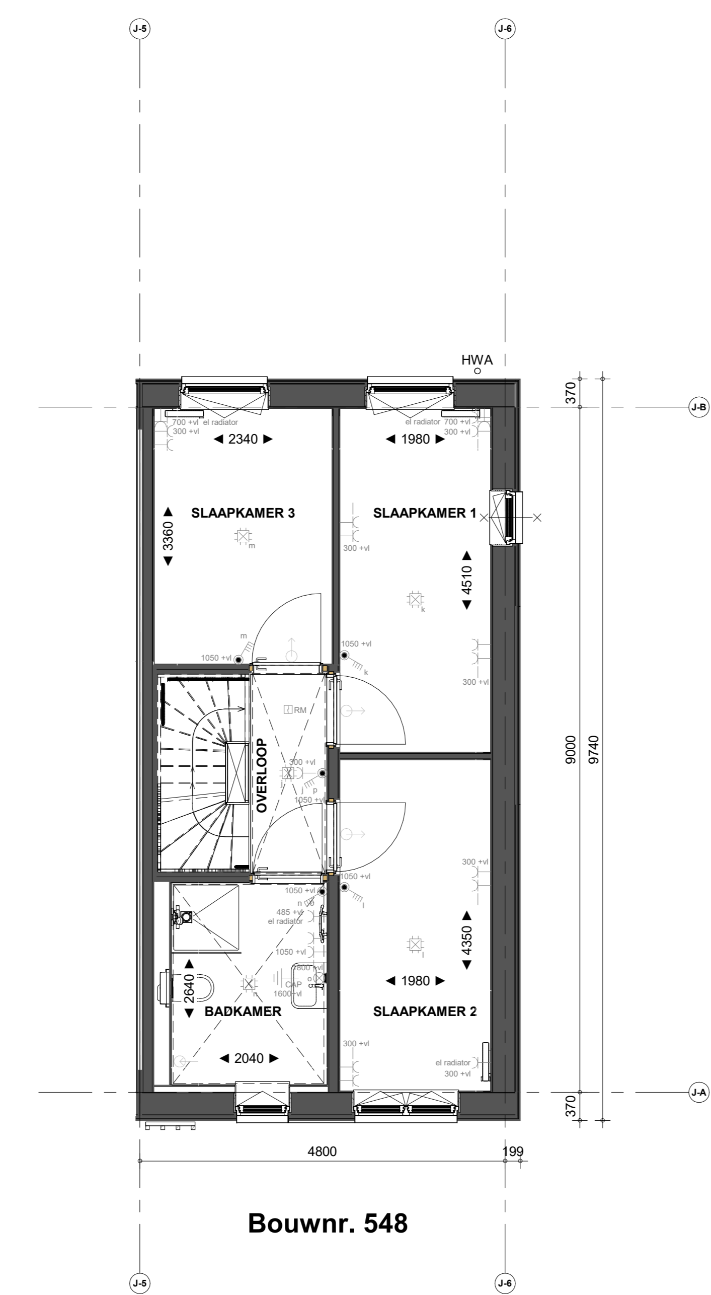
1e verdieping
