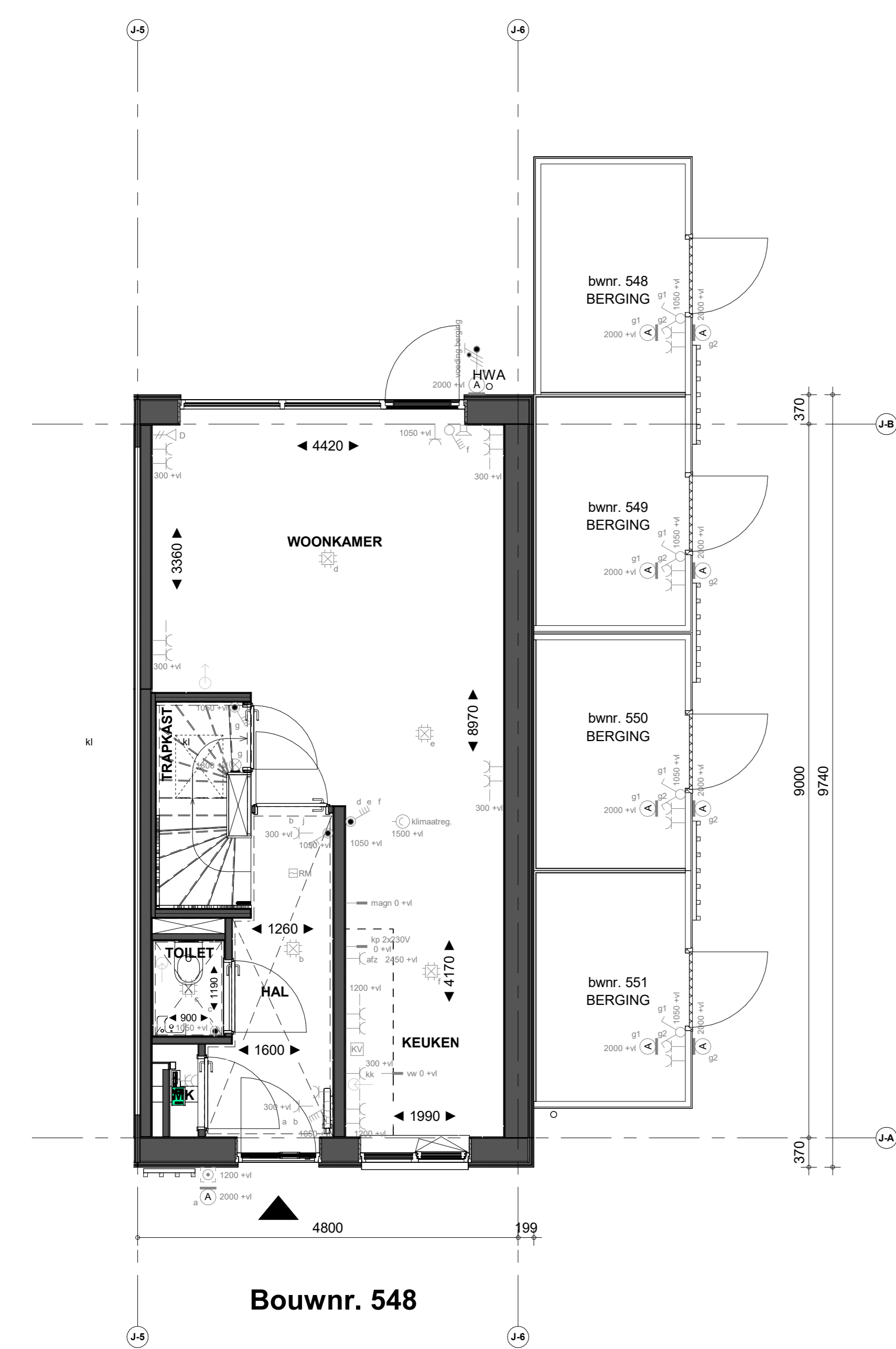
Begane grond
