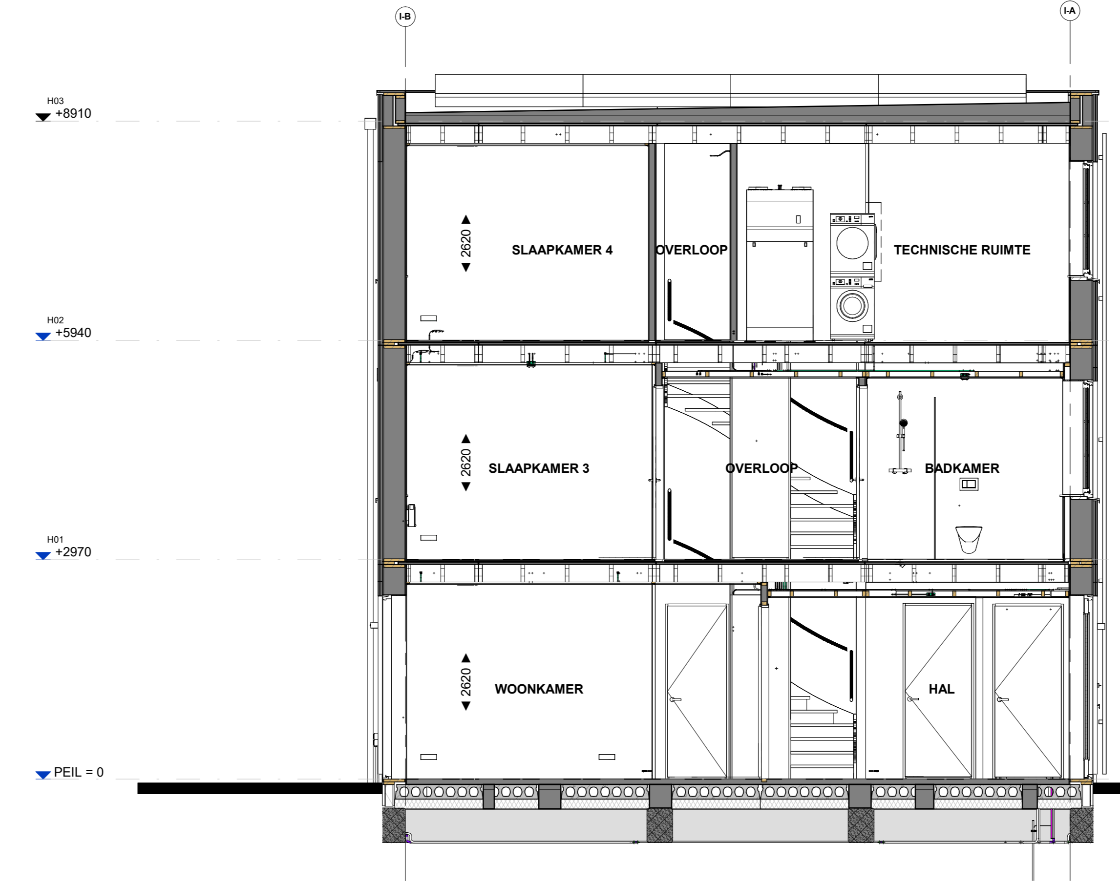
Doorsnede B549
