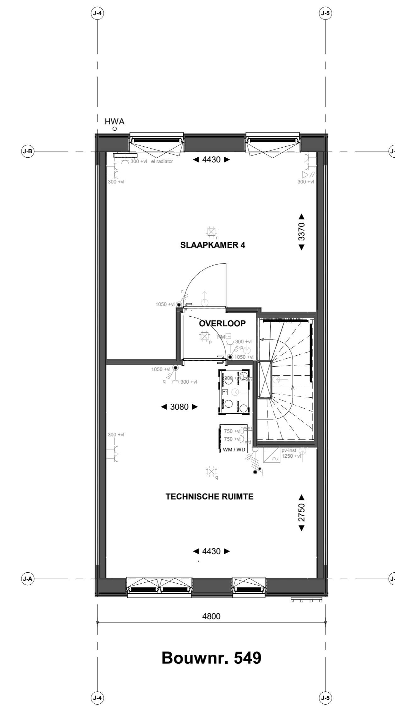
2e verdieping
