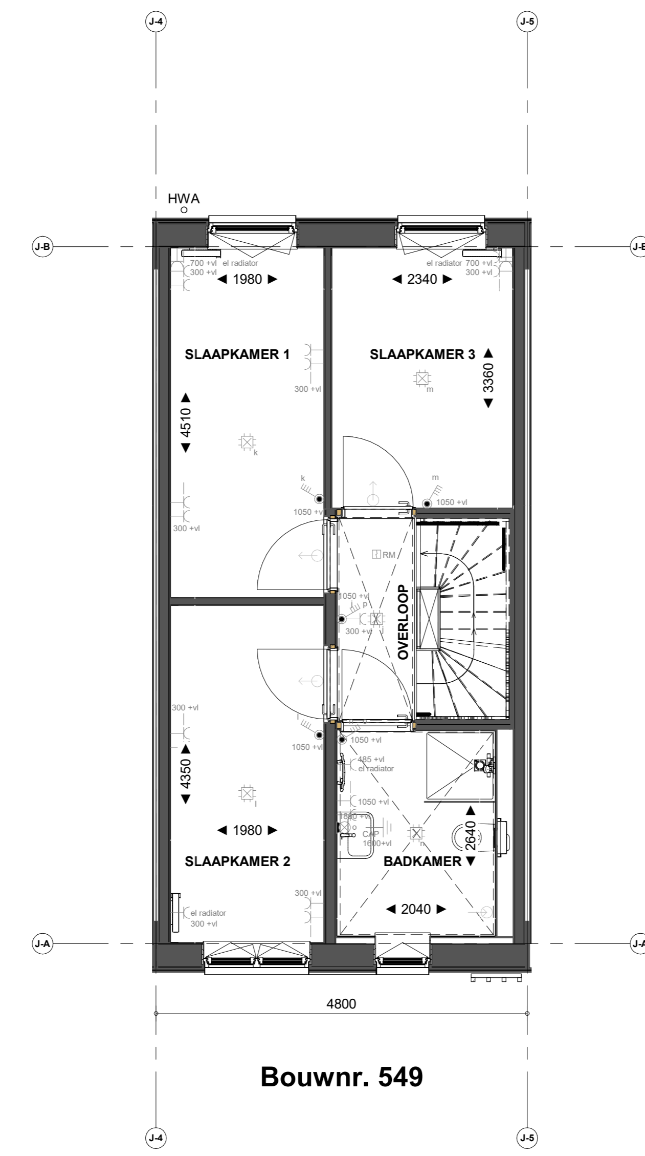
1e verdieping
