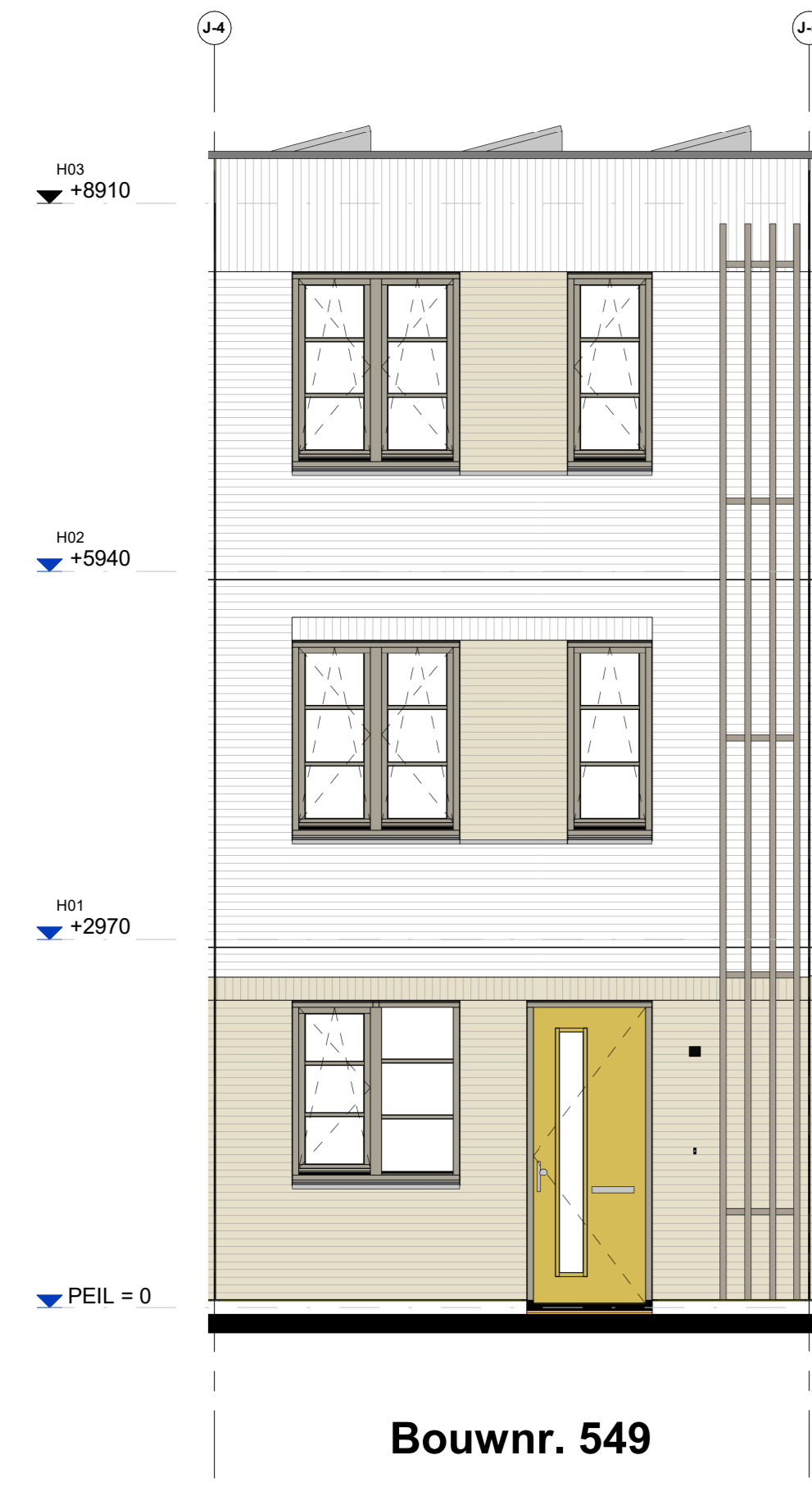
Voorgevel
