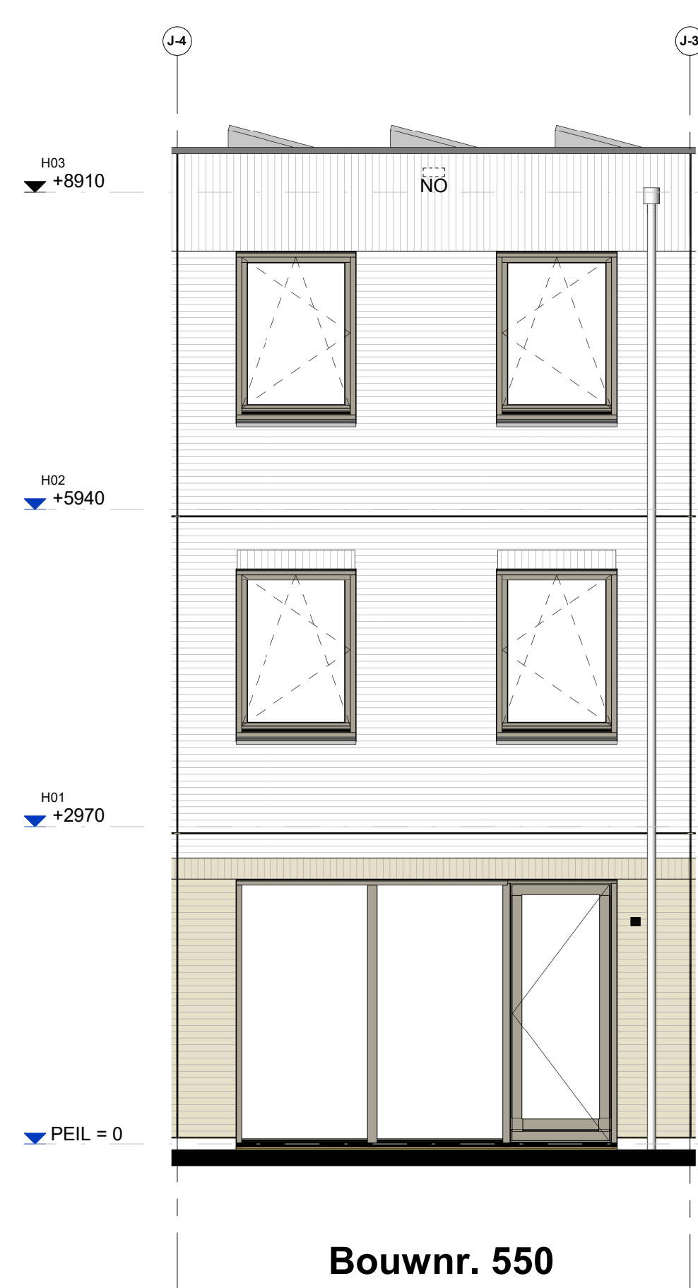
Achtergevel
