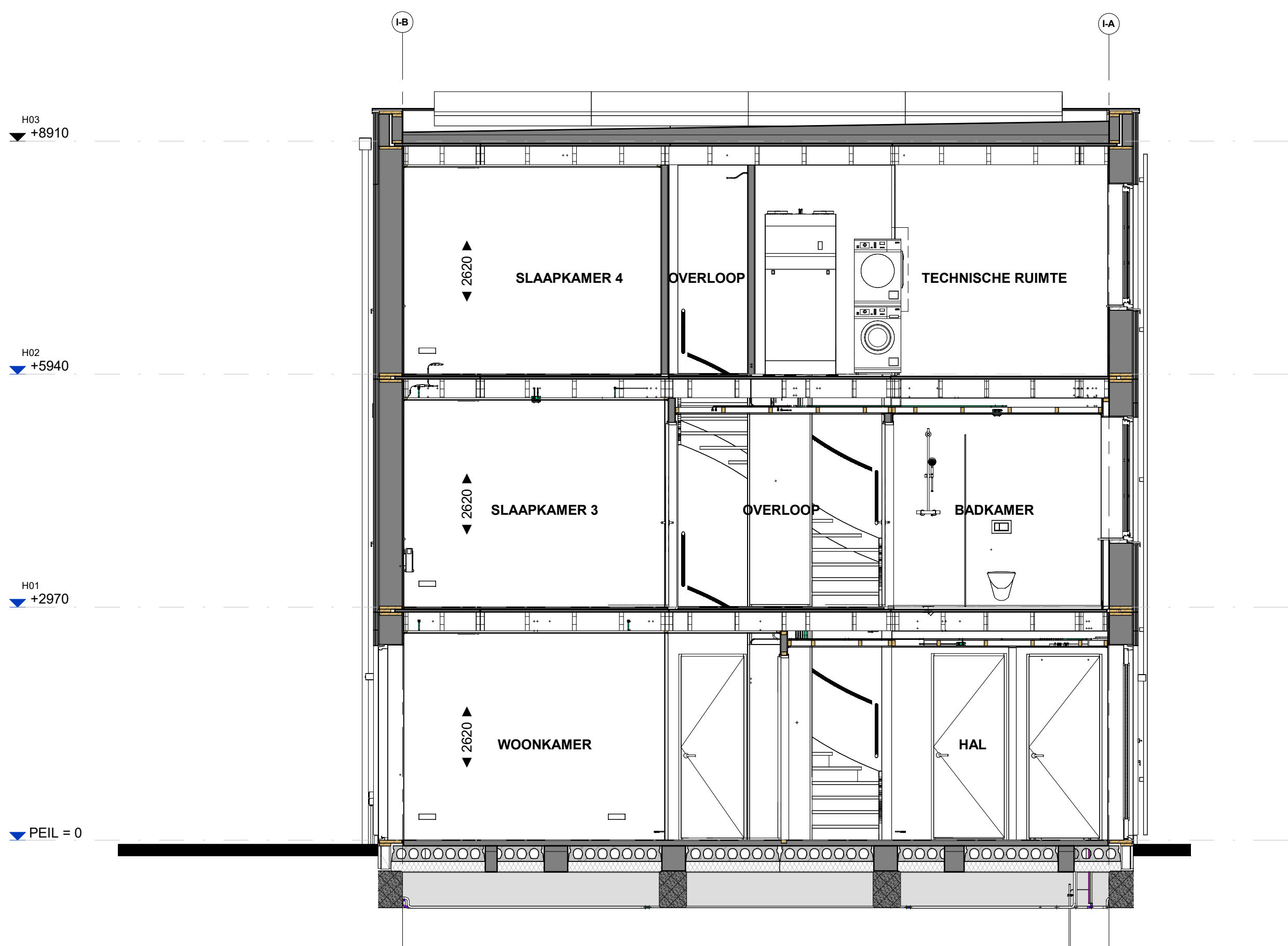
Doorsnede B550
