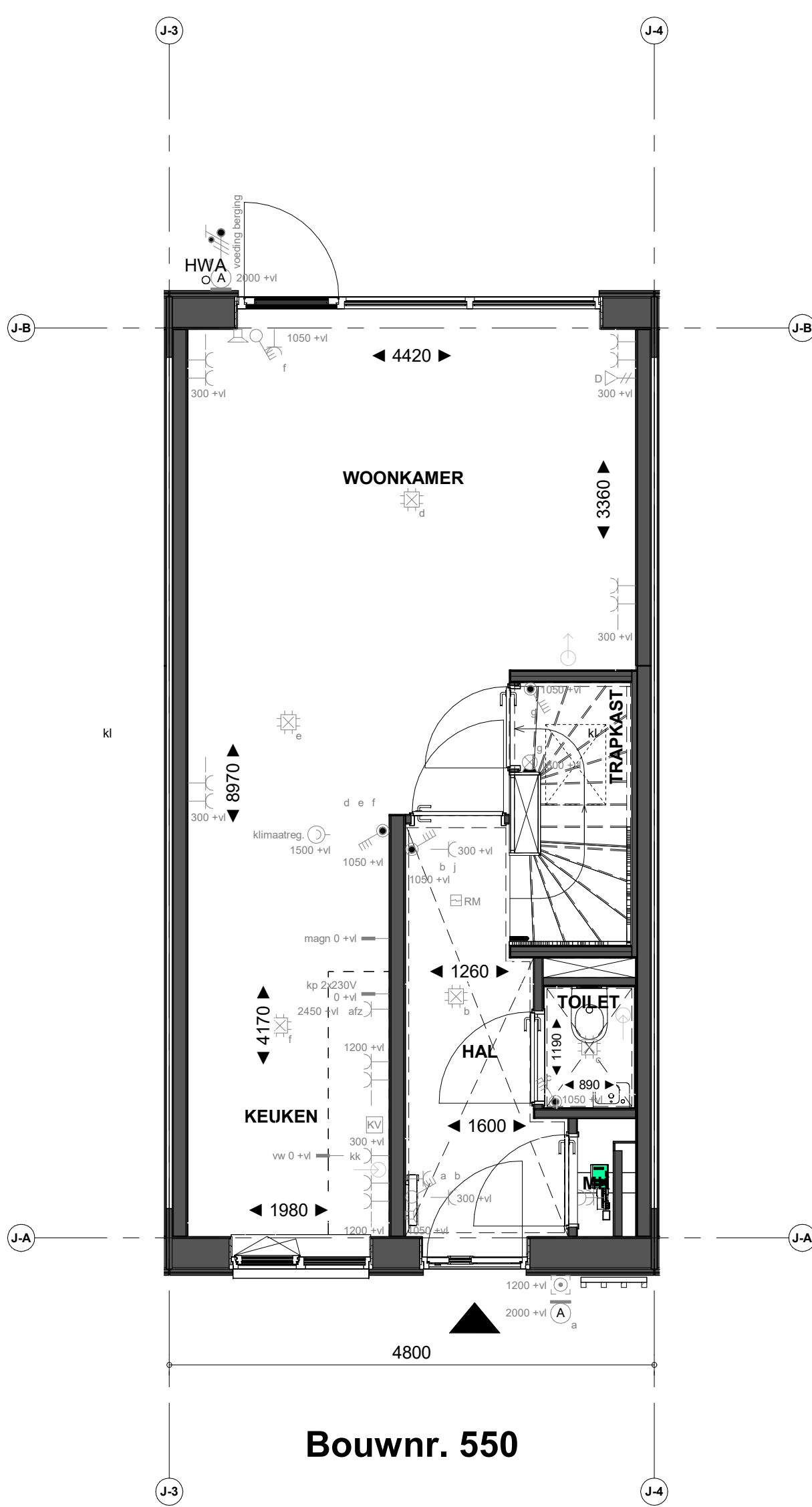
Begane grond
