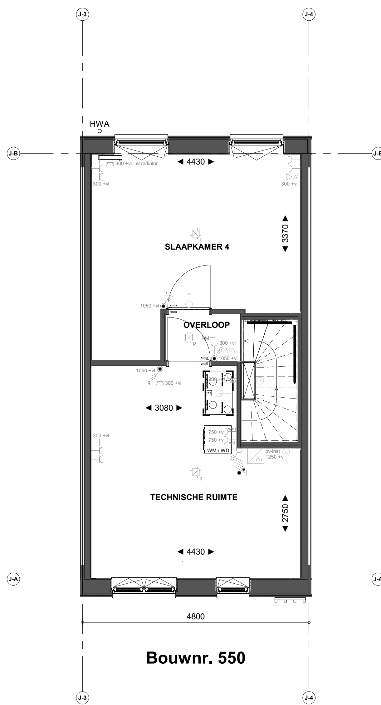
2e verdieping
