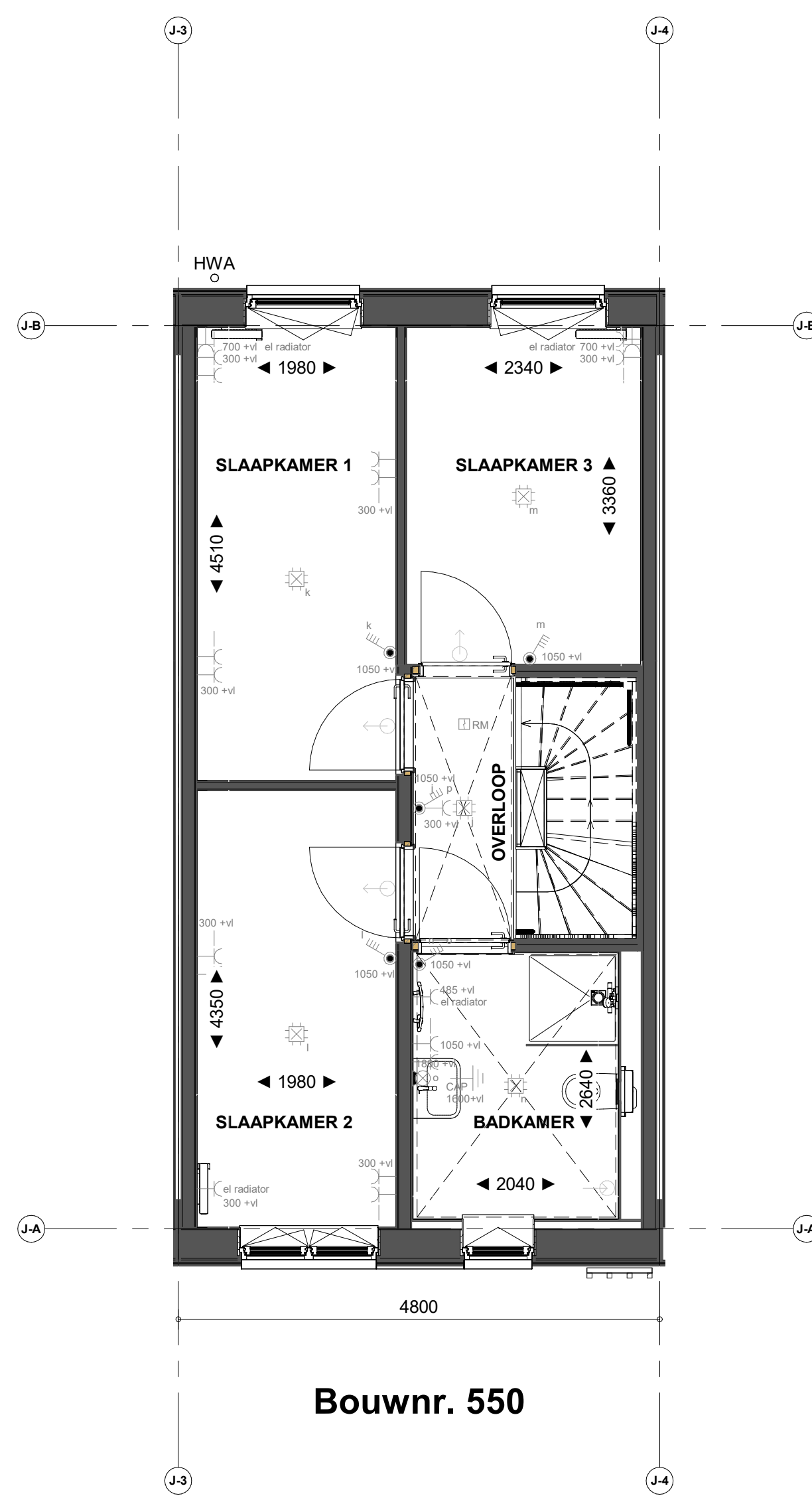
1e verdieping
