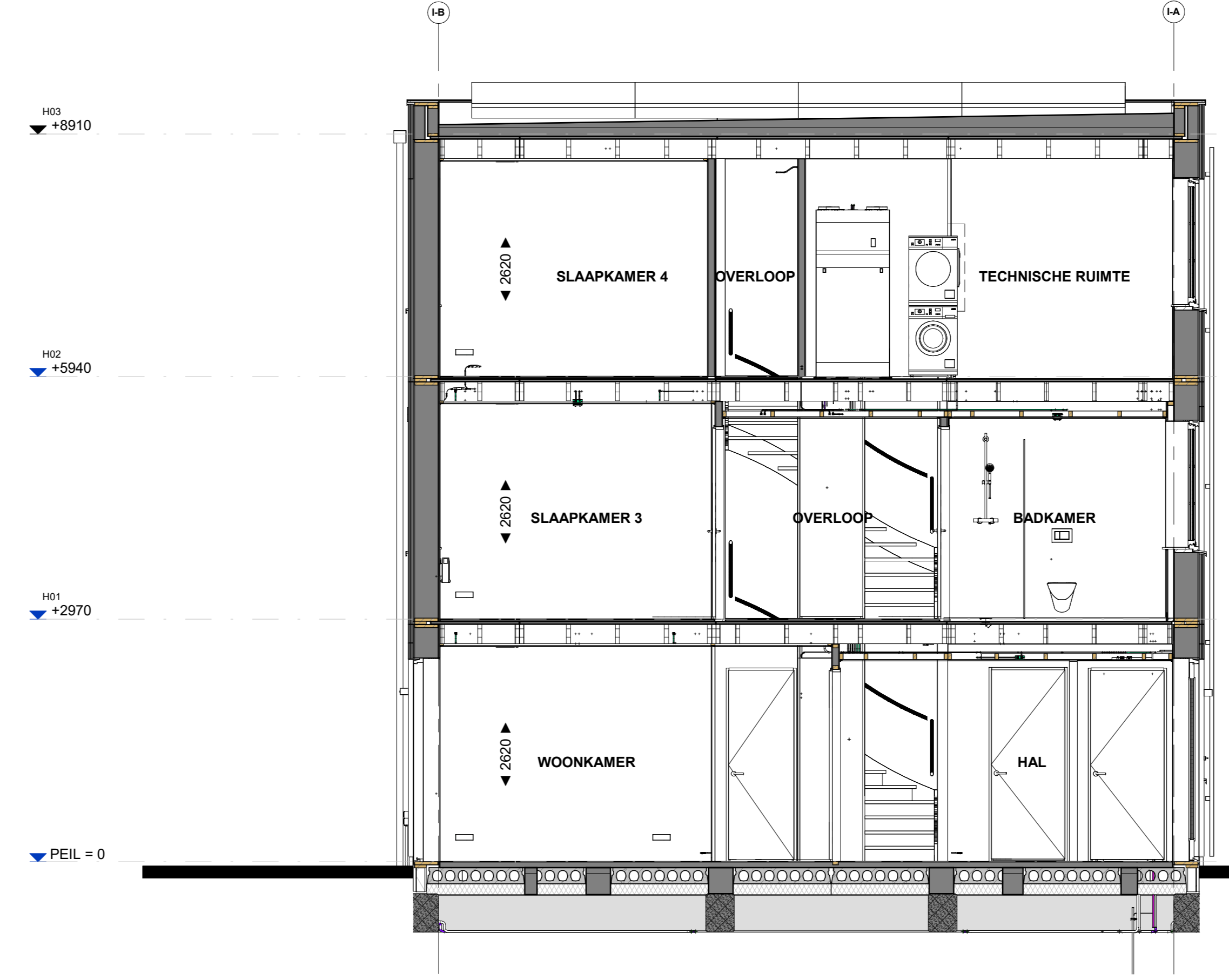
Doorsnede B551
