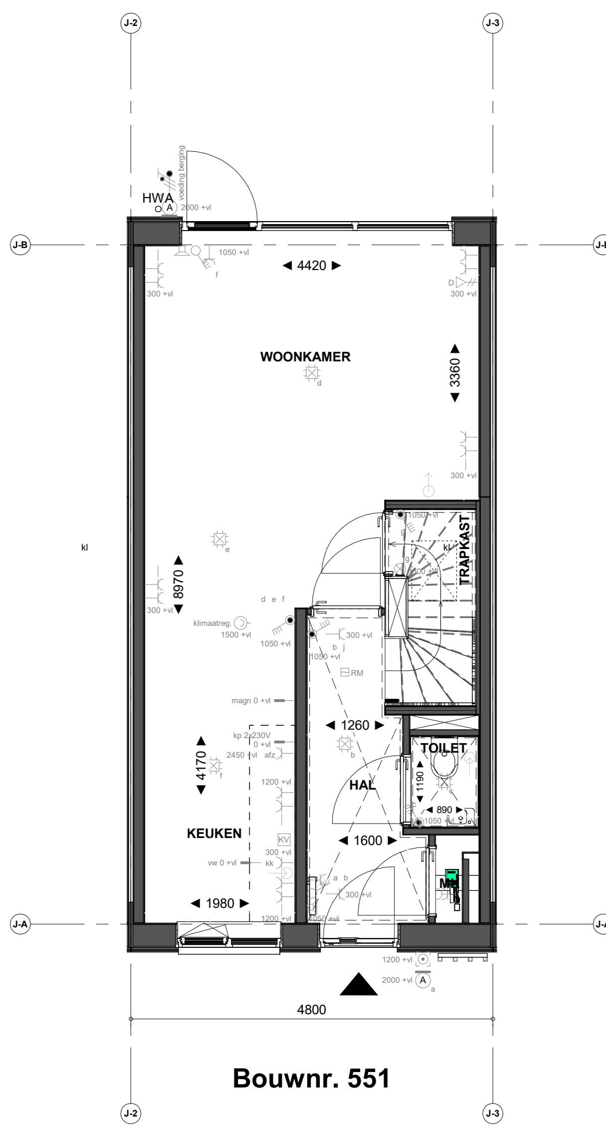
Begane grond
