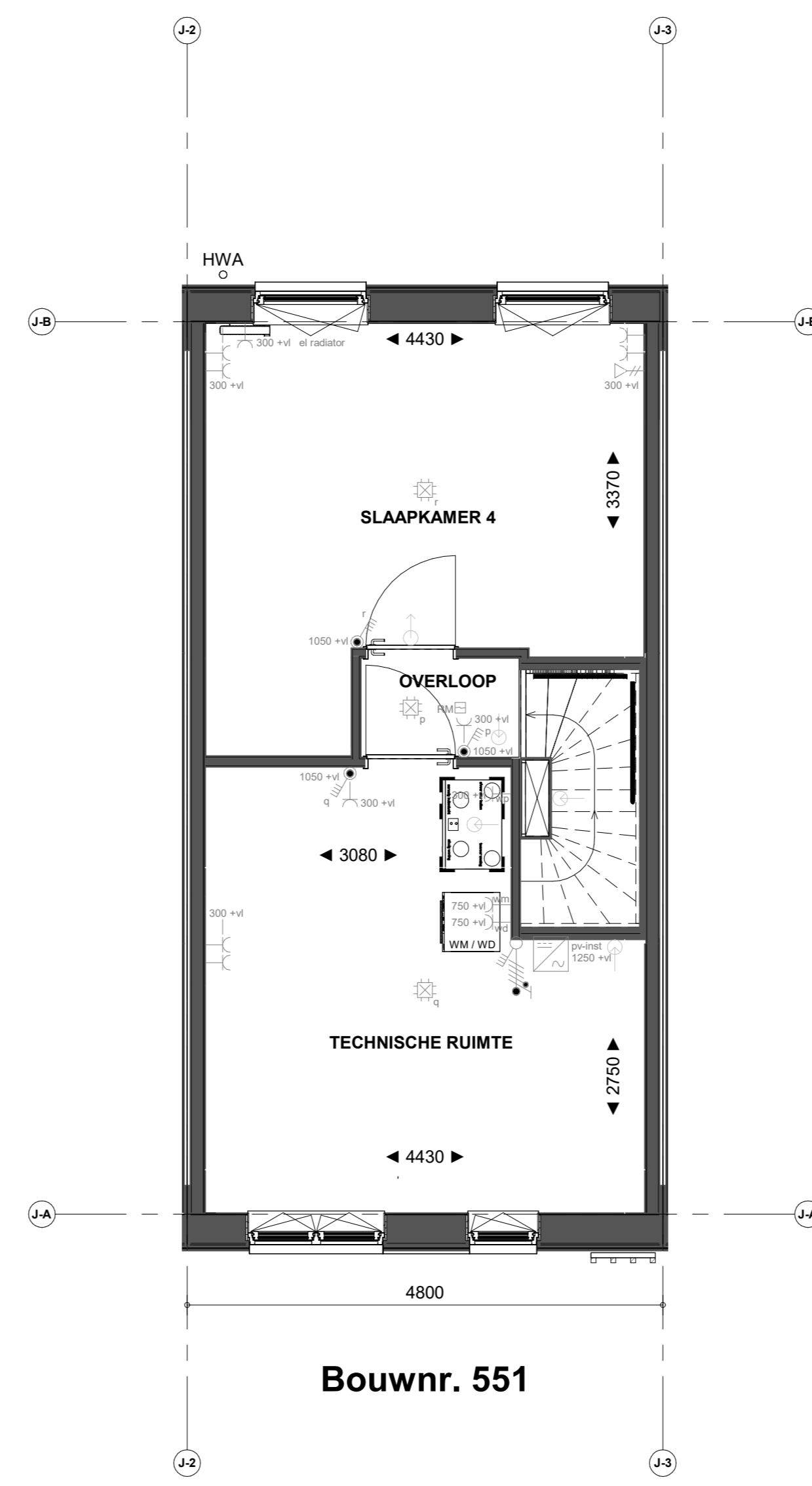
2e verdieping
