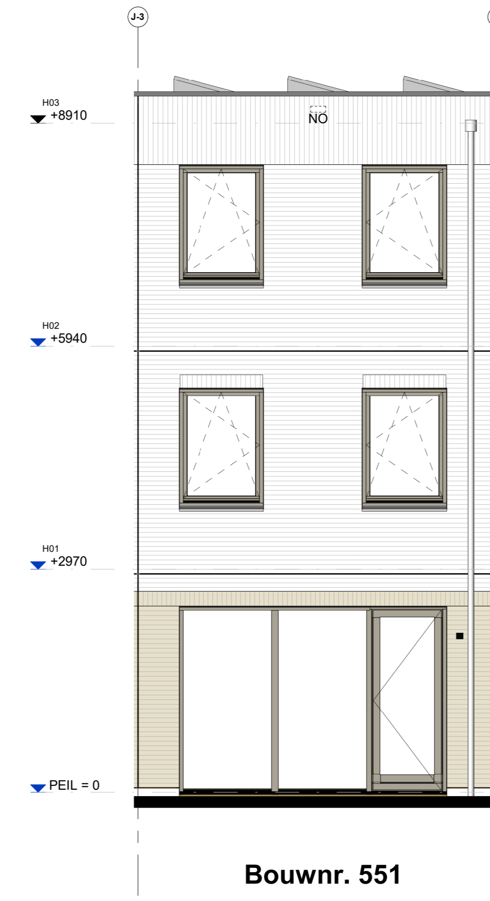
Achtergevel
