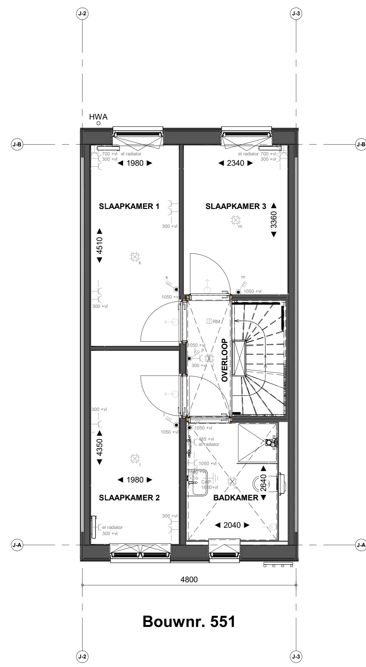
1e verdieping
