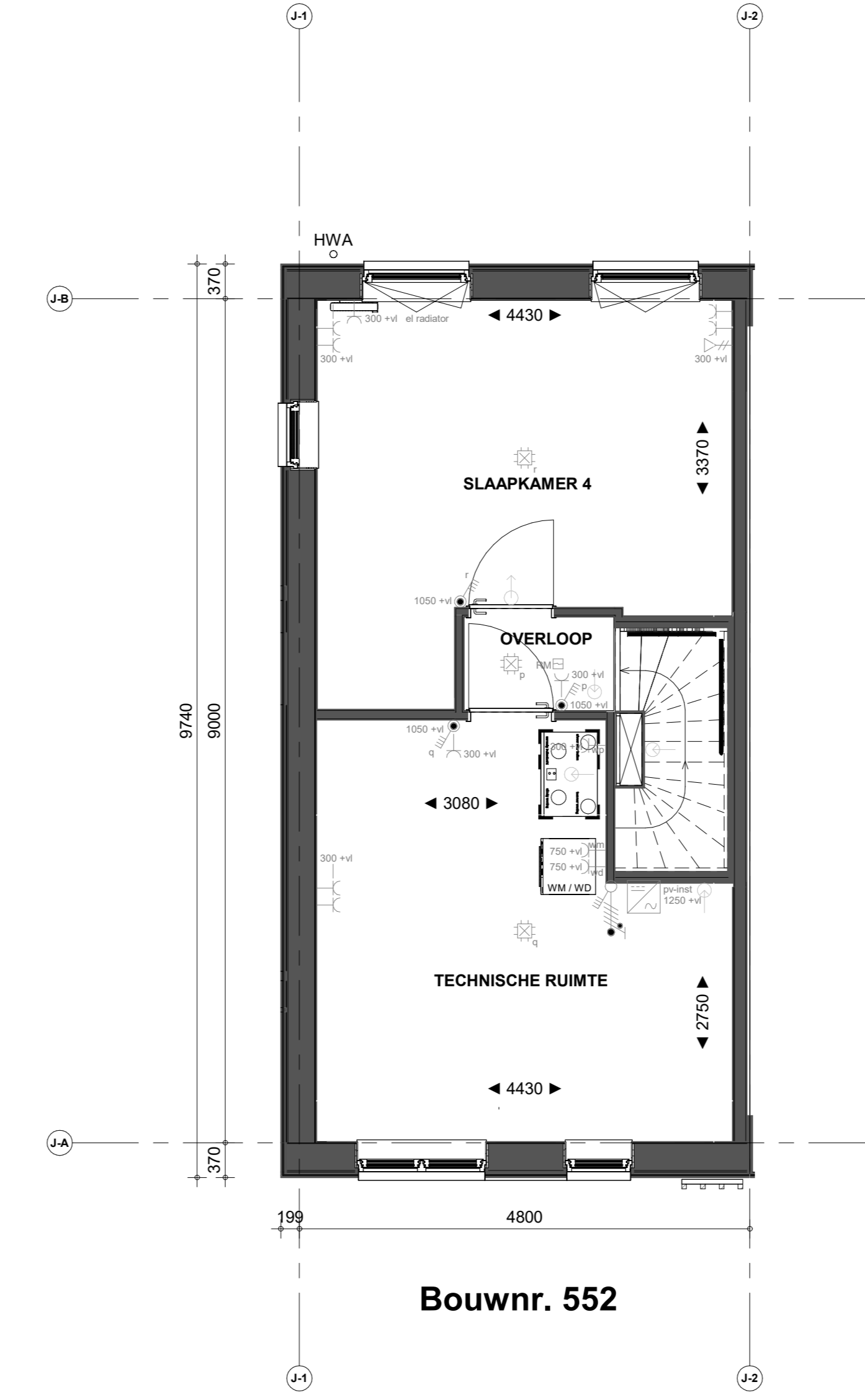
2e verdieping
