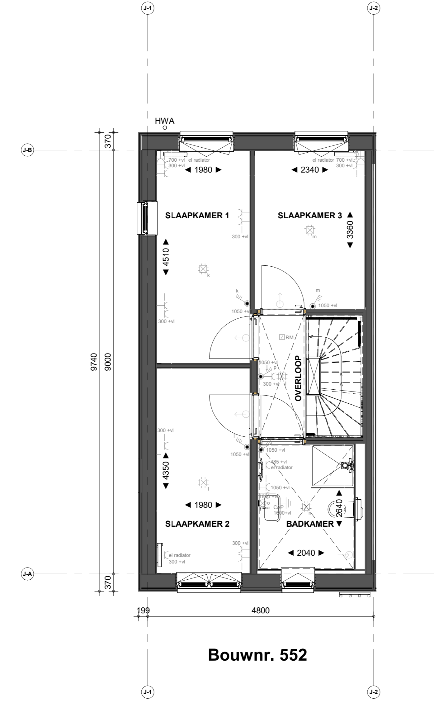
1e verdieping
