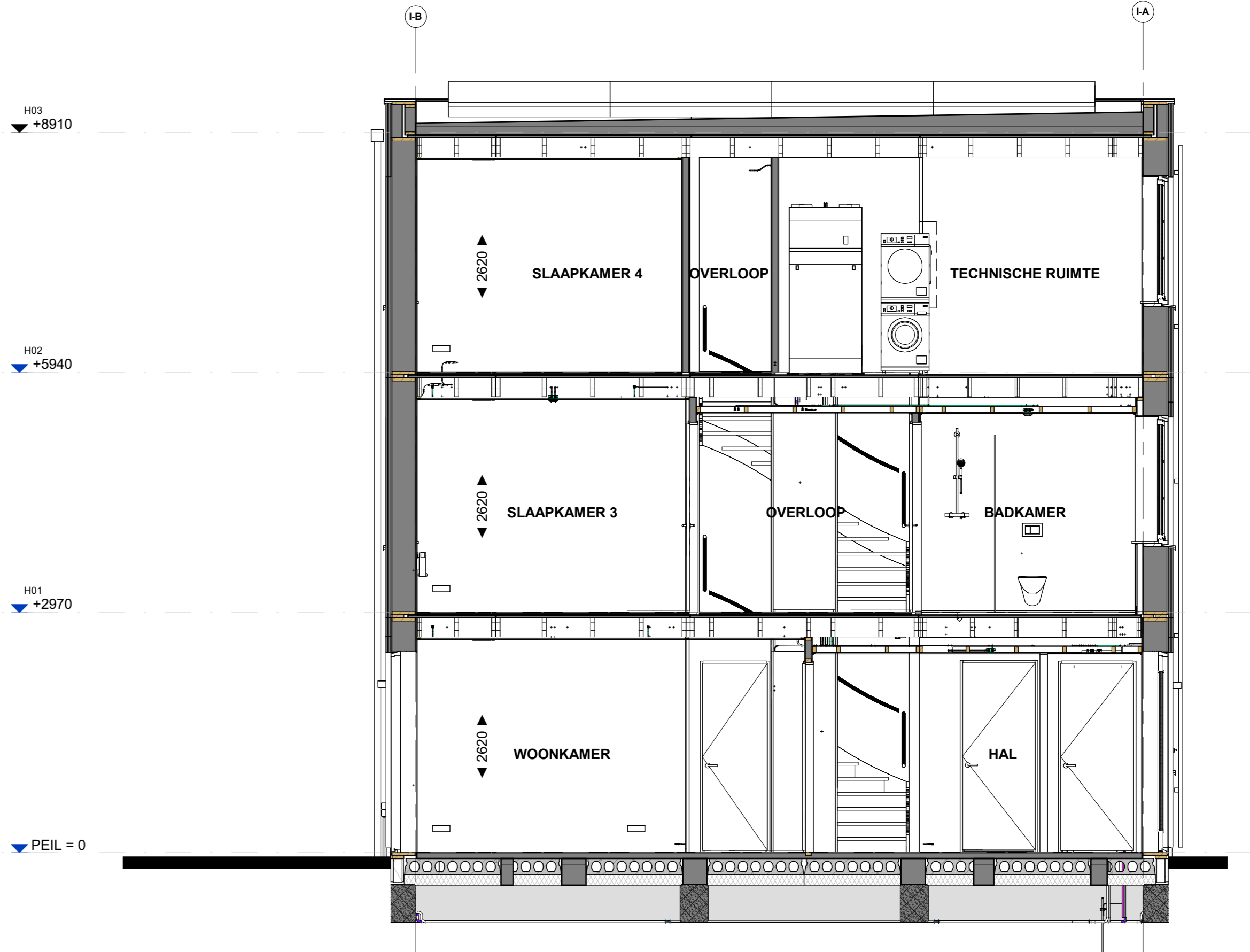
Doorsnede B552
