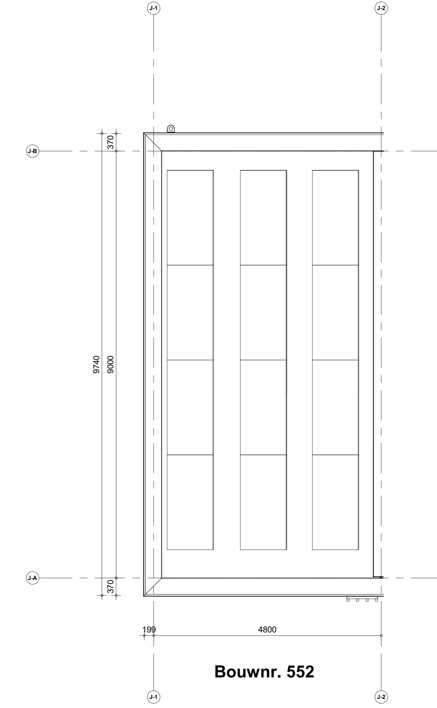
Dakaanzicht
